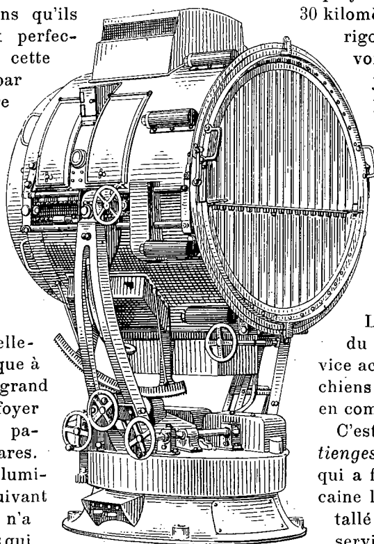
Nouveau projecteur électrique de la marine autrichienne.
