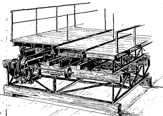
LA PLATE-FORME MOBILE. — Le mécanisme.
