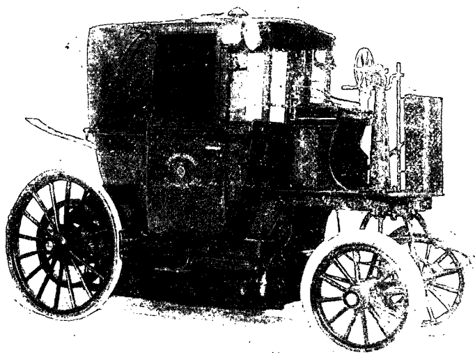
FIACRES ÉLECTRIQUES. — Landaulet.
