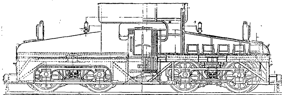
Locomotive électrique du Central London Railway .
