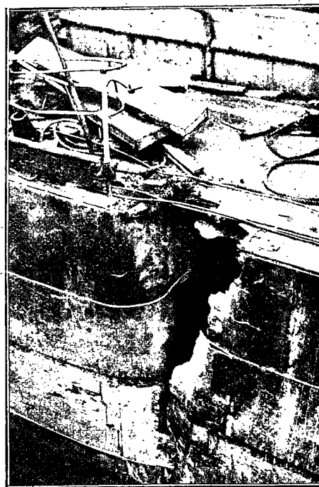
Bordage défoncé d'un navire de 3.000 tonneaux.
