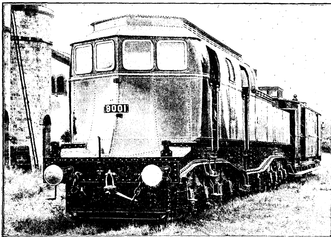
LA NOUVELLE LOCOMOTIVE ÉLECTRIQUE HEILMANN.
