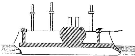
Cuirassé d'escadre. — Les parties hachées sont seules revêtues d'une cuirasse.
