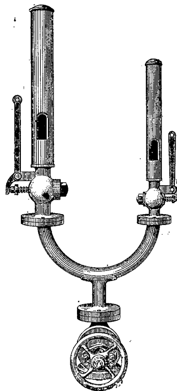
Sirène tubulaire de M. Brunel.
