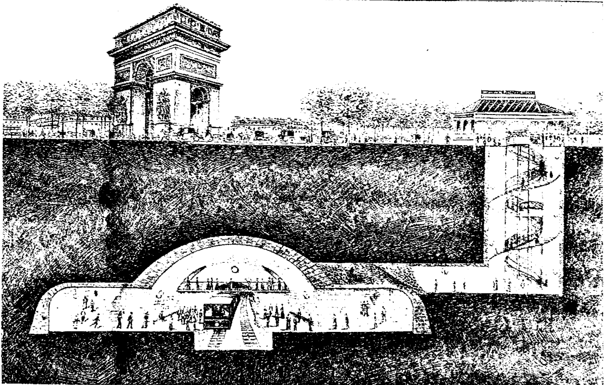
TRAMWAY TUBULAIRE BERLIER. — FIG. 3. — Station de l'Étoile: coupe transversale.
