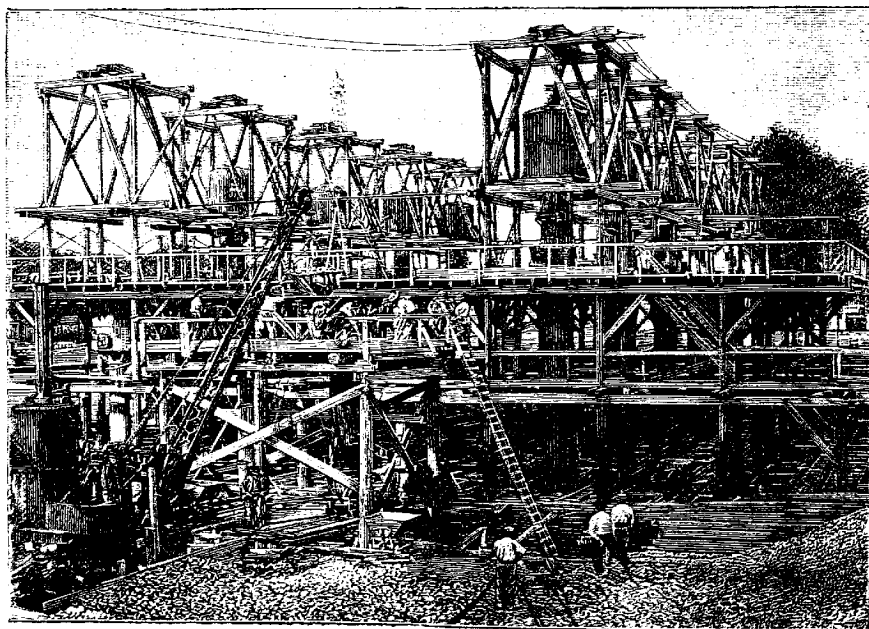
CONSTRUCTION DU PONT ALEXANDRE III. — Vue d'un Caisson (octobre 1897). (Photographie de M. Haby).
