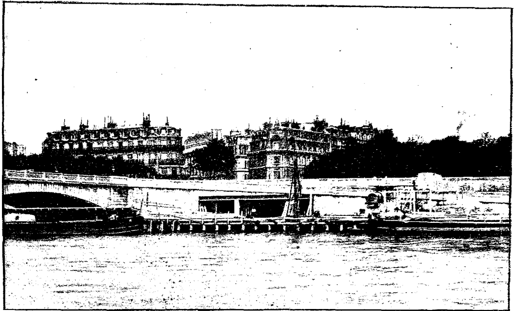
Appontement et tunnel pour le transport des matériaux à pied d'œuvre et l'évacuation des déblais (Phot. de M. Haby).
