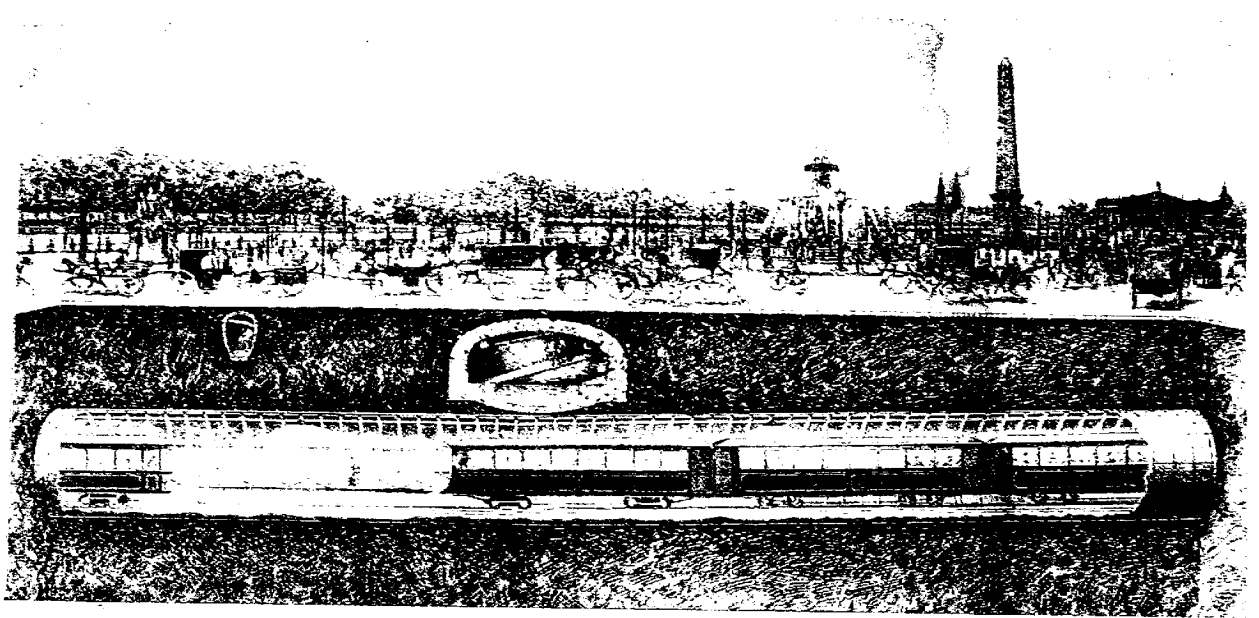
TRAMWAY TUBULAIRE BERLIER. — FIG. 1. — Passage sous le collecteur d'Asnières, place de la Concorde.
