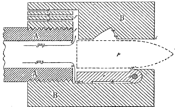
Appareil pour canon de 80 m/m de campagne. Echelle 1/4. A.A. extrémité de la volée du canon. — aa bouche du canon. — BB bloc fixé à l'extrémité du canon par une vis à deux secteurs pleins et deux secteurs interrompus; ce bloc peut se visser et se dévisser avec la plus grande facilité. — c volet mobile autour d'un axe x . — ddd canaux cylindriques très étroits, placés sur des cercles concentriques à l'axe du canon et sur la demi-circumference supérieure. — ff rainure demi-cylindrique dans laquelle débouchent les canaux ddd . — ggg face du bloc contre lequel vient s'appliquer le volet c . — hh espace dans lequel se répandent les gaz de la poudre pour actionner le volet. — x axe de rotation du volet.
