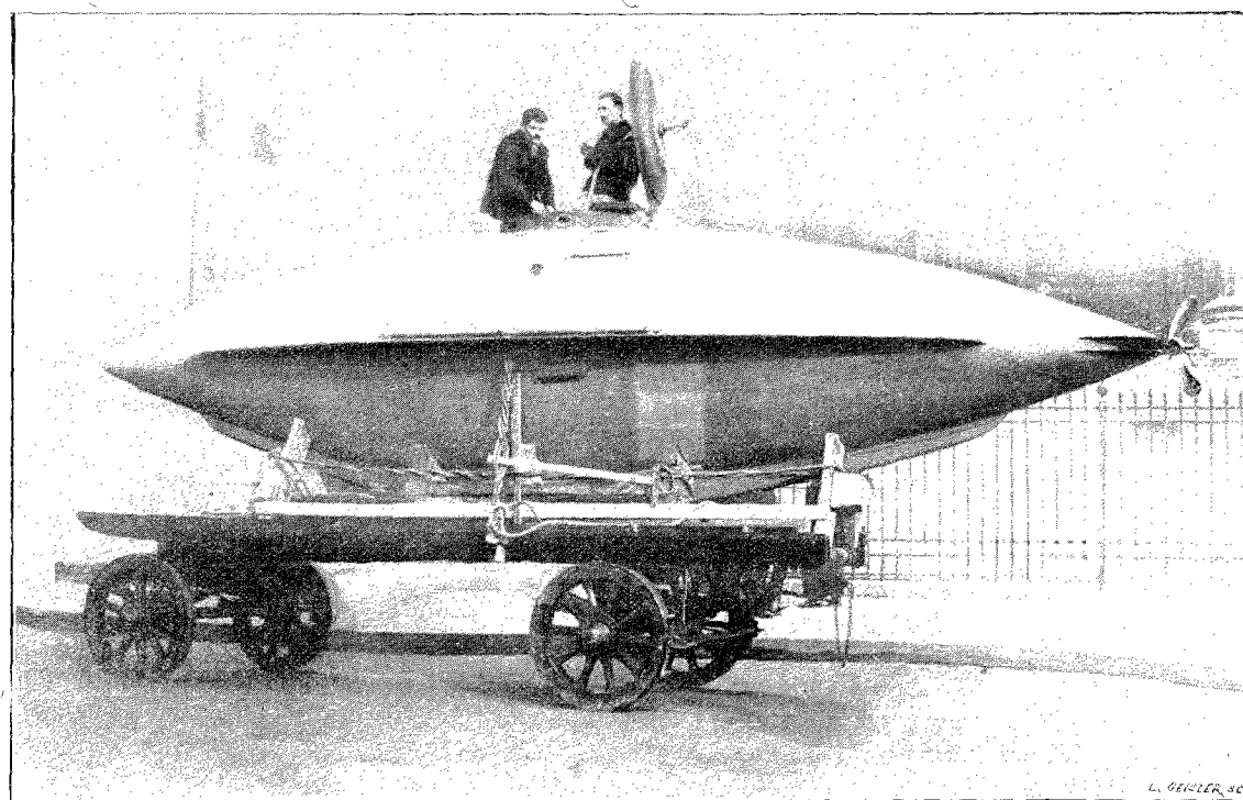
LE GOUBET. — FIG. 1. — En route pour le bassin d'Argenteuil, arrêt devant la Madeleine.
