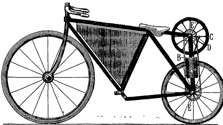
FIG. 3. — Bicyclette à pétrole. — Modèle d'essai.
