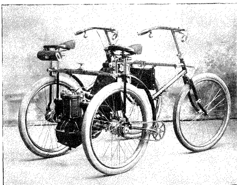
Sociable automobile Morel (moteur de Dion et Bouton), construit avec les bicyclettes pliantes du capitaine Gérard.
