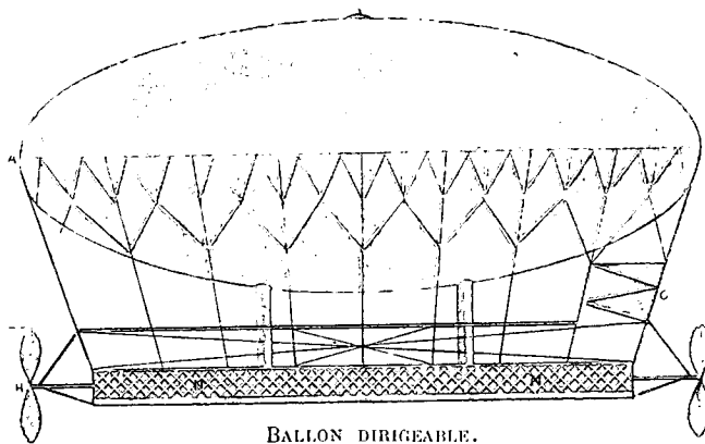
A, avant; B, arrière; G, gouvernail; HH, hélices; NN, nacelle.
