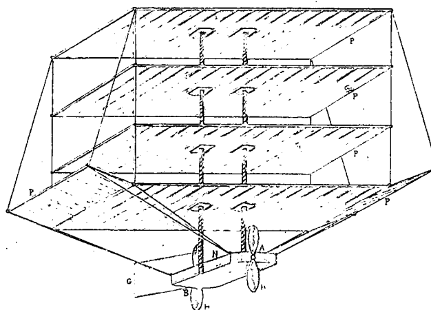
Aérodrome vu par dessous.
