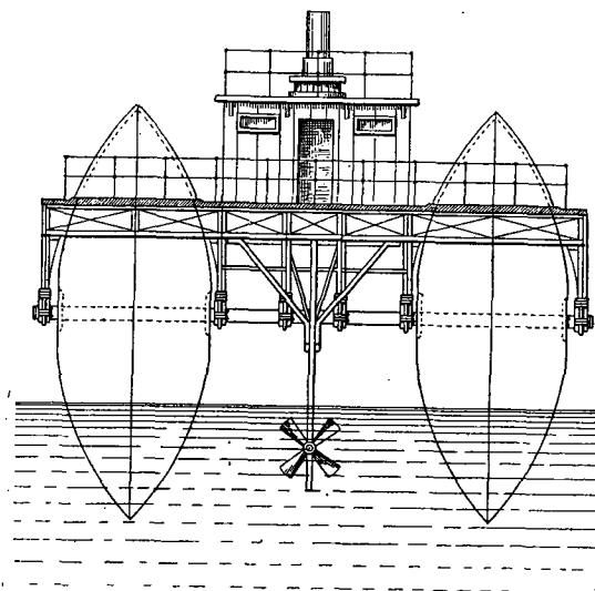
Bateau-rouleur, vu de face.
