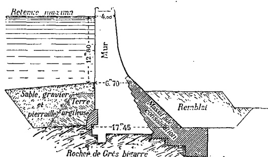
FIG. 2. — Coupe transversale de la digue consolidée en 1889.
