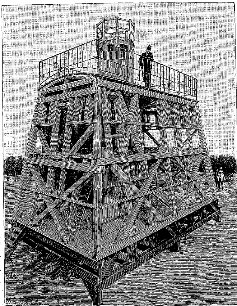
Observatoire construit à Meudon, d'après les plans de M. Janssen, et destiné à être édifié au sommet du Mont-Blanc.
