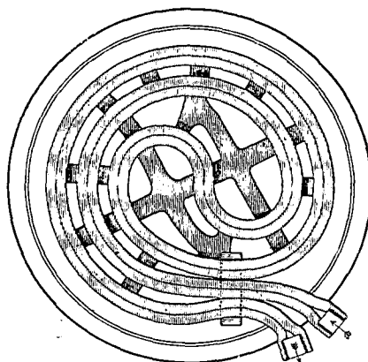
FIG. 1. — Générateur de vapeur du système Serpollet.
