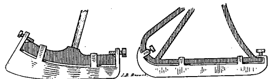
Vélocipède à neige et à glace.
