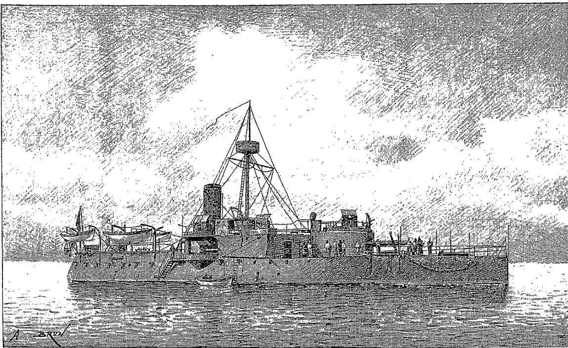
LA MARINE FRANÇAISE DE GUERRE. — Canonnière cuirassée de 1 re classe Styx . — Longueur 58 m. 80.
