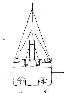
Coupe verticale au maître couple du premier navire à hélices centrales, le Louvre . — A A' Hélices centrales.
