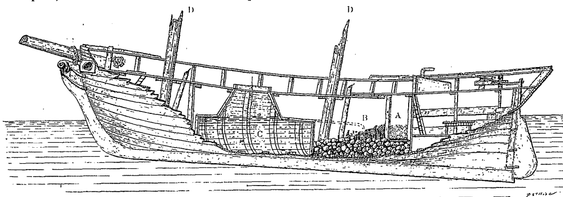
A LA MER. — Les pêcheries modernes à l'étranger. (fig. 2). — Coupe d'un schooner à vivier américain A, Glacière. — B, Morceaux de glace. — C, Vivier. — DD, Mats.
