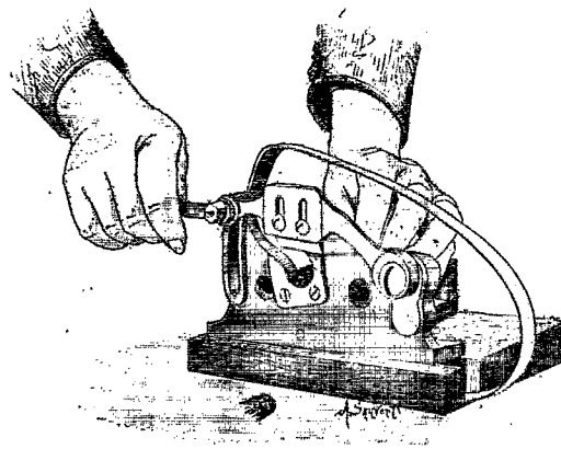
FIGURE 4. — Machine à couper les cigares à la longueur réglementaire.
