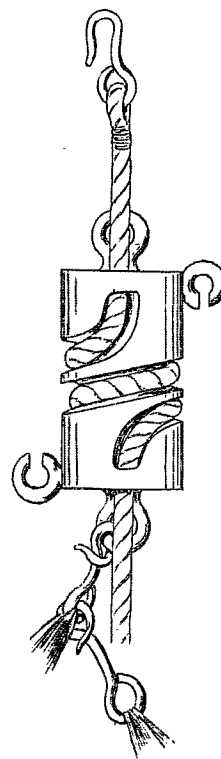
Descenseur à spirale.
