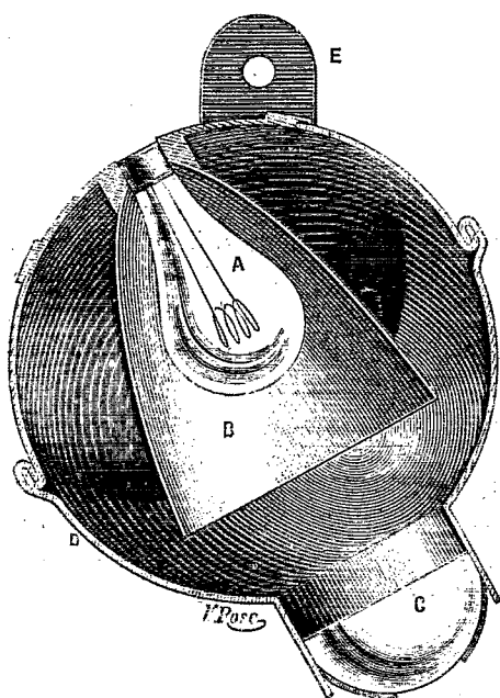
FIG. 1. — Lampe à incandescence suspendue à la voûte du tunnel et projetant sa lumière sur les plaques d'étain des parois. — A, lampe à incandescence. — B, réflecteur parabolique. — C, lentille divergente. — D, boîte en tôle emboutie. — E, patte de suspension.
