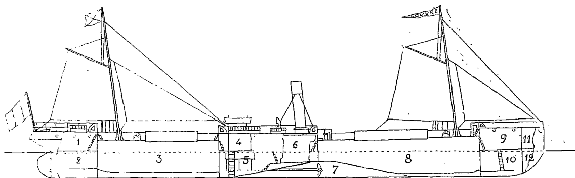
LE Louvre , PREMIER NAVIRE À HÉLICES CENTRALES. — Coupe longitudinale du Louvre : 1, Logements arrière ; 2, Coqueron à provisions ; 3, Cale à marchandises arrière ; 4, Chambre du mécanicien ; 5, Machine ; 6, Chaudière ; 7, Tunnel d'une hélice ; 8, Cale à marchandises avant ; 9, Poste de l'équipage ; 10, Cale à vin ; 11, Magasin ; 12, Coqueron.
