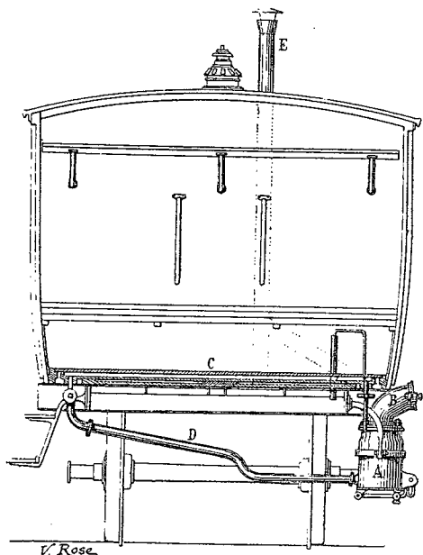
LE CHAUFFAGE DES WAGONS. — FIG. 3. — Appareil à thermo-siphon adapté aux wagons. — Vue latérale d'un wagon muni de l'appareil. — A. Chaudière. — B. Ouverture du foyer de la chaudière. — C. Cana- lisation partant de la partie supérieure de la chaudière et amenant l'eau chaude dans les bouillottes. — D. Cana- lisation ramenant l'eau refroidie dans le bas de la chaudière. — E. Cheminée du foyer.
