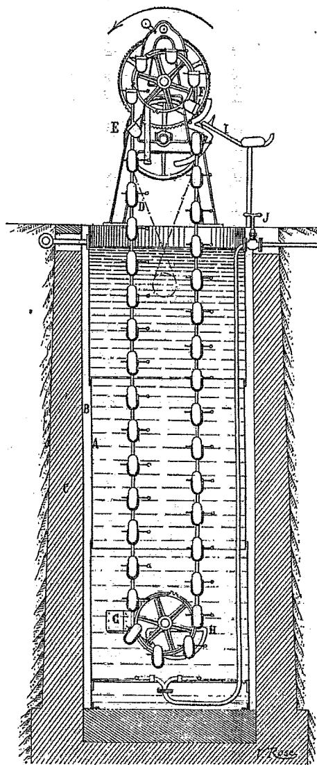
LE CHAUFFAGE DES WAGONS. — Fig. 6. — Appareil à noria pour le réchauffement des bouillottes. — A. Eau chaude. — B. Enveloppe de la cuve. — C. Puits. — D. Paniers destinés à recevoir les bouillottes. — E. Panier recevant la bouillotte froide. — F. Panier renversé laissant tomber la bouillotte chaude. — G.-H. Appareil servant à empêcher les bouillottes de sortir des paniers. — I. Plan incliné par lequel tombent les bouillottes réchauffées. — J. Robinet d'adduction de la vapeur destinée au réchauffage de l'eau de la cuve.
