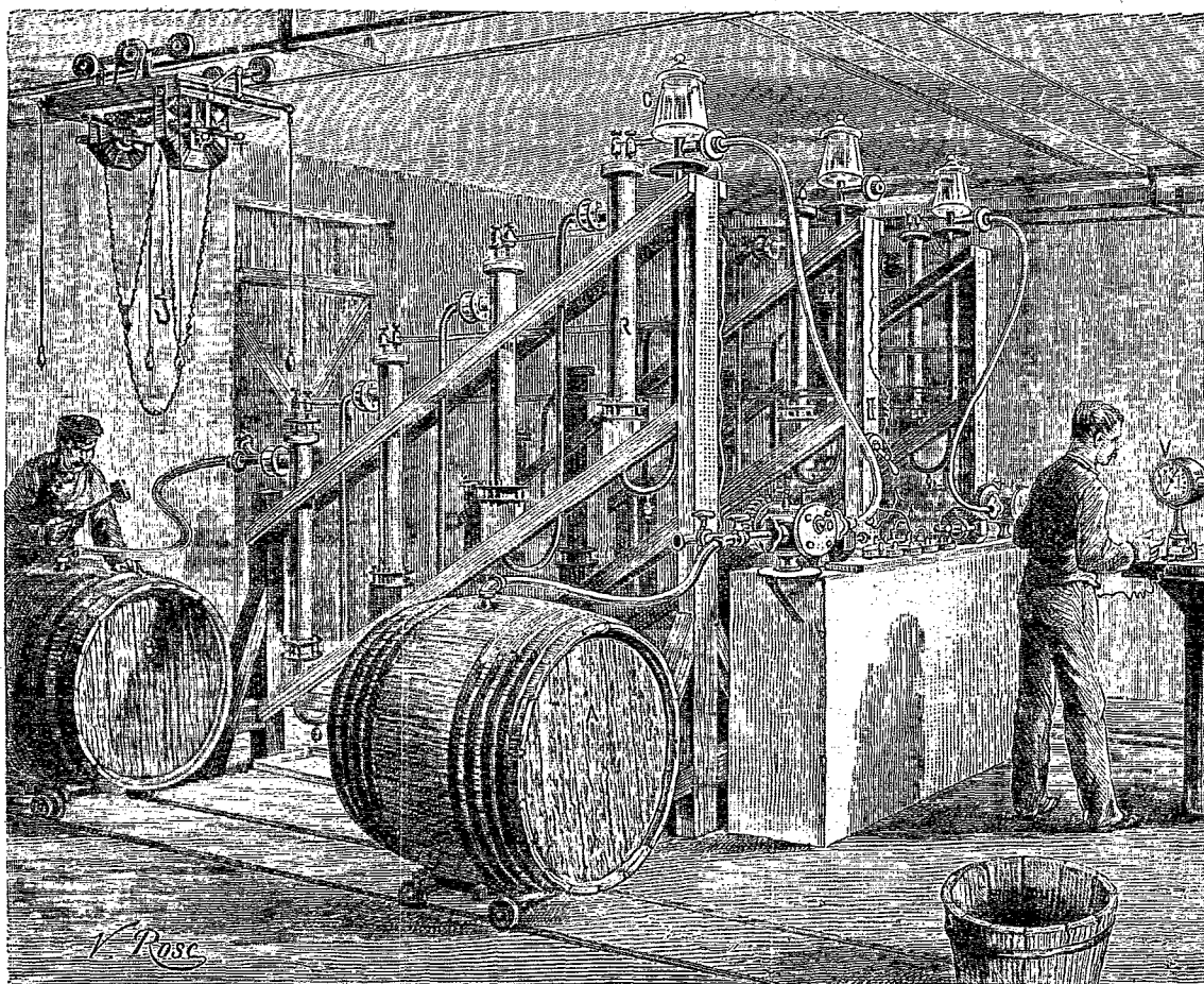
EXPÉRIENCES SUR LA CONSERVATION ET LE VIEILLISSEMENT DES VINS PAR L'ÉLECTRICITÉ AU DÉPÔT DE BERCY (FIG. 2). Vue d'ensemble : A. Tonneau de prise du liquide à traiter. — B. Tonneau récepteur du liquide traité. — C. Réservoir en verre pour constater le niveau du vin dans l'appareil. — P. Pompe. — R. Récipients en grès dans lesquels le vin est soumis aux chocs électriques. — T. Wagonnet-treuil électrique pour le transport et le levage des fûts. — V. Appareil électrique pour mesurer le degré d'alcool des vins.
