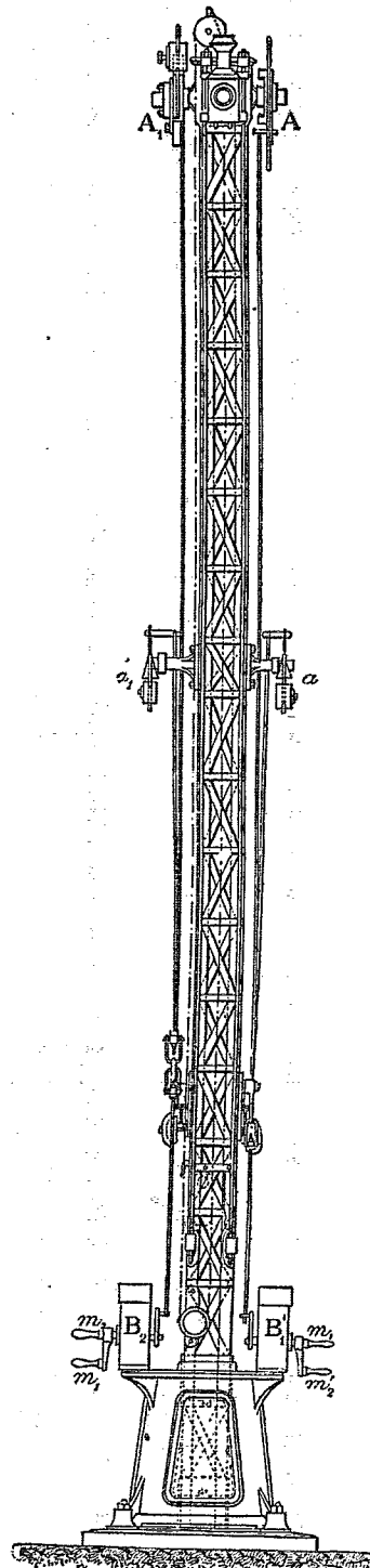
Fig. 2. — Électro-sémaphore (élévation).
