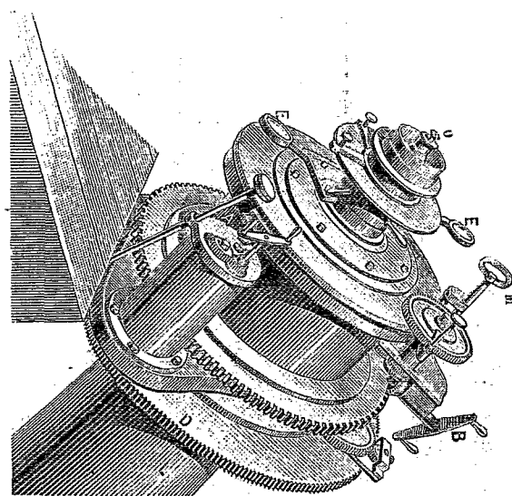
LE NOUVEL ÉQUATORIAL COUDÉ DE M. LÉVY. — FIG. 2. — Extrémité supérieure de la lunette dans le salon de l'observateur. — O. Oculaire de la lunette. — E. E. Lentilles pour la lecture sur le cercle divisé. — M. Manette pour mettre en marche le mouvement d'horlogerie. — A. Manivelle servant à mouvoir le cube terminal. — B. Manivelle servant à faire tourner l'instrument sur lui-même.
