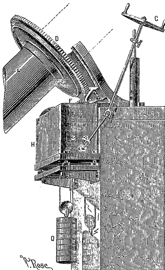
LE NOUVEL ÉQUATORIAL COUDÉ DE M. LÉVY. — FIG. 1. — Détails du mouvement d'horlogerie servant à faire mouvoir l'instrument sur lui-même. — L. Lanette. — G. Manivelle pour remonter le mouvement d'horlogerie. — D. Roue dentée. — F. Vis de commande de la roue D. — H. Boîte renfermant le mouvement d'horlogerie. — Q. Contrepoids.
