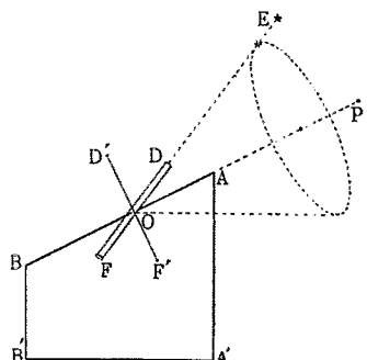
FIG. 5. — Schéma d'un équatorial ordinaire.
