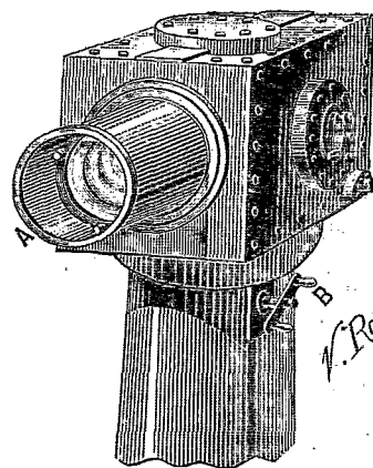
LE NOUVEL ÉQUATORIAL COUDÉ DE M. LÉVY. — FIG. 3. — Cube terminal renfermant l'objectif et le miroir-plan. — A. Miroir plan. — B. Manivelle.
