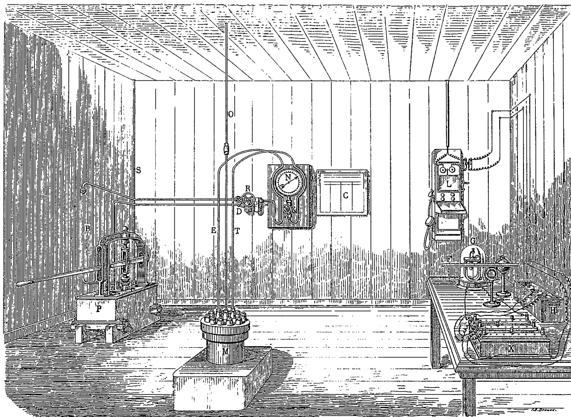
LE MANOMÈTRE DE LA TOUR EIFFEL. — FIG. 4. — Vue du laboratoire installé dans le pilier ouest de la tour. — Dessin de Drouot.
