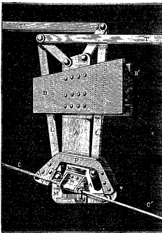
TRAMWAY FUNICULAIRE DE BELLEVILLE. — FIG. 3. — Perspective du grip. — A. Plaque de tôle. — BB'. Plats houlonnés sur la plaque de tôle. — P. Plaque guide. — CC'. Câble. — M. Mâchoire supérieure. — M'. Mâchoire inférieure. — LL. Levier. — TT'. Renvoi de commande.
