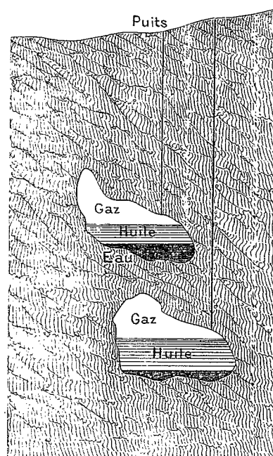
Graphique hypothétique des gisements pétroliers.
