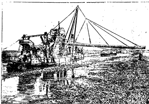
Le dessèchement des marais de Fos. — Dragage à long couloir, dans le genre des dragues employées pour le canal de Suez. Le couloir conduit les déblais jusqu'à la distance convenable pour élever la digue.
