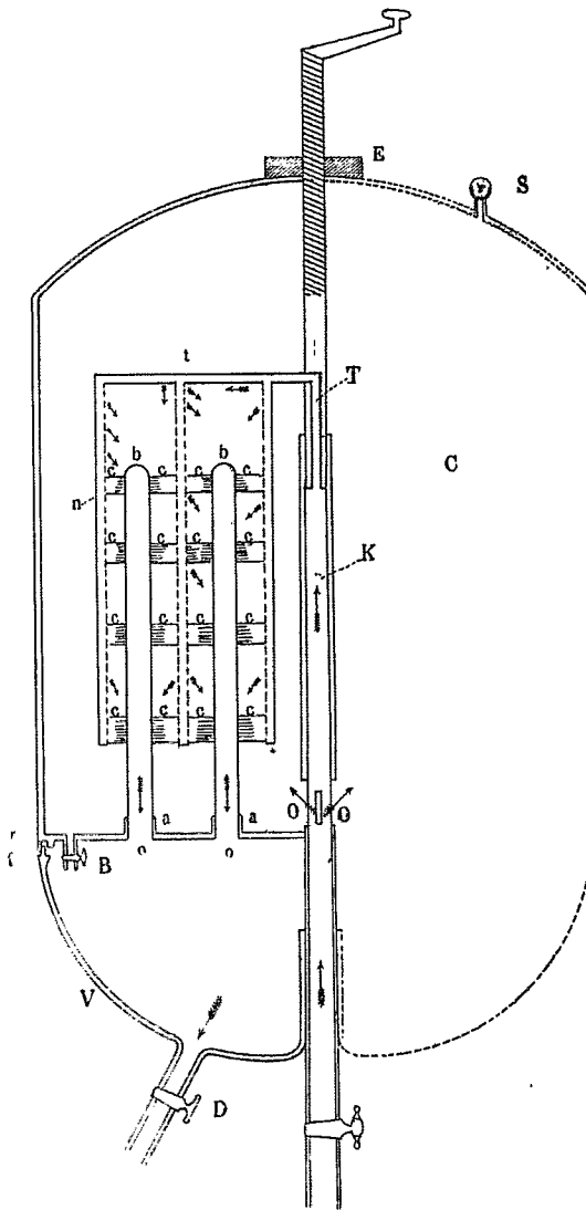
Schéma d'un filtre applicable aux fontaines publiques.
