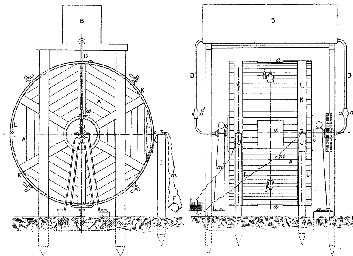
Le tannage des peaux par l'électricité. — Vue latérale et vue de face de l'appareil de tannage.
