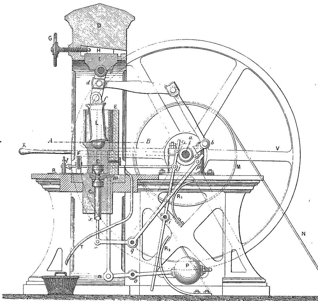
PRESSE MONÉTAIRE. — ÉLEVATION.
