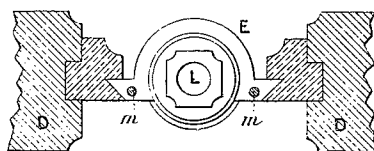
FIG. 3. — D , bâti. — L , pièce actionnée par le levier e f . — E , pièce maintenant la boîte à coin supérieure et soulevée par le levier m n o p qui aboutit en m m .
