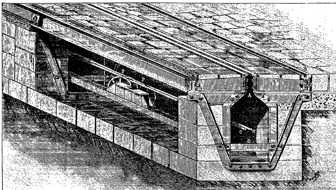
TRAMWAY FUNICULAIRE DE BELLEVILLE. FIG. 4. — Coupe de la voie. — A. Fer en Z. — B. Rail système Broca. — EE'. Entretoises. — CC'. Câble aller et retour. — D. Traverse. — PP'. Poulies.
