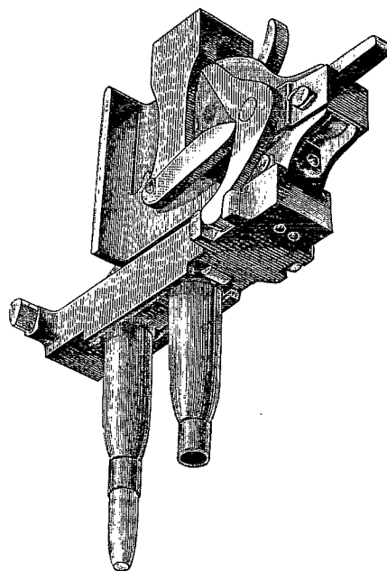
FIGURE 5. — Mitrailleuse Maxim. — Culasse mobile.
