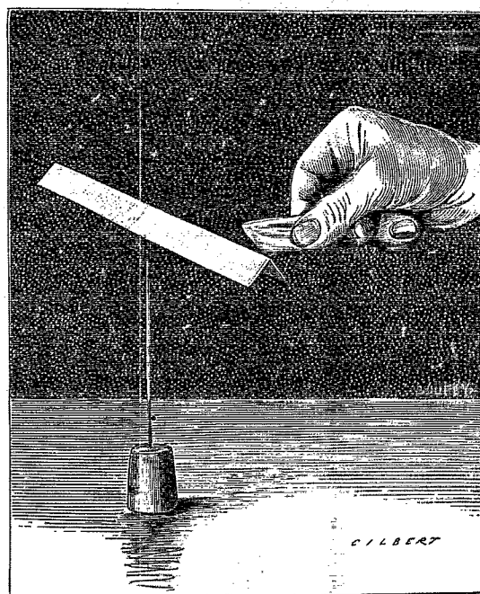
La science au coin du feu. — Électroscope formé d'une longue aiguille piquée dans un bouchon et d'une bande de papier pliée en deux.
