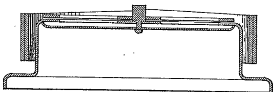
Coupe verticale du régulateur automatique.
