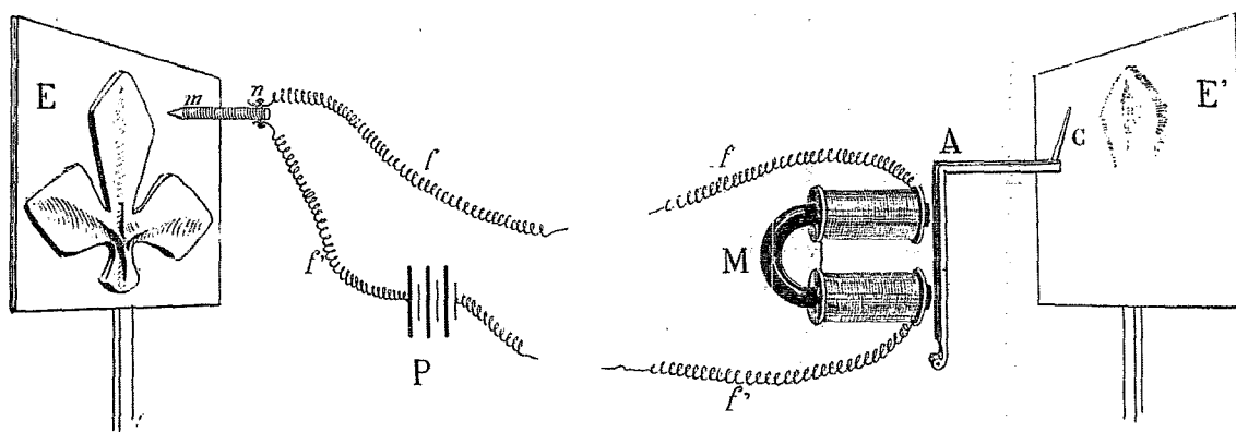
Schéma théorique du téléphote.
