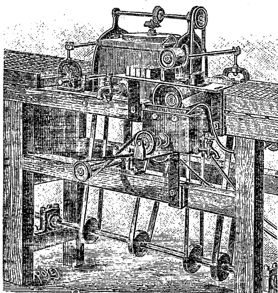
L'Industrie des allumettes. — Détail d'une machine à appliquer le « gratin » sur les boîtes d'allumettes.
