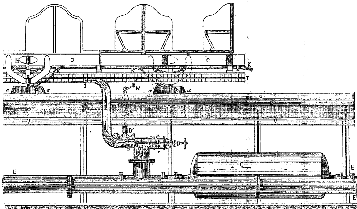
FIG. 4. — Coupe longitudinale du chemin de fer glissant (Se reporter, pour les indications des lettres, à la légende de la figure 5.)
