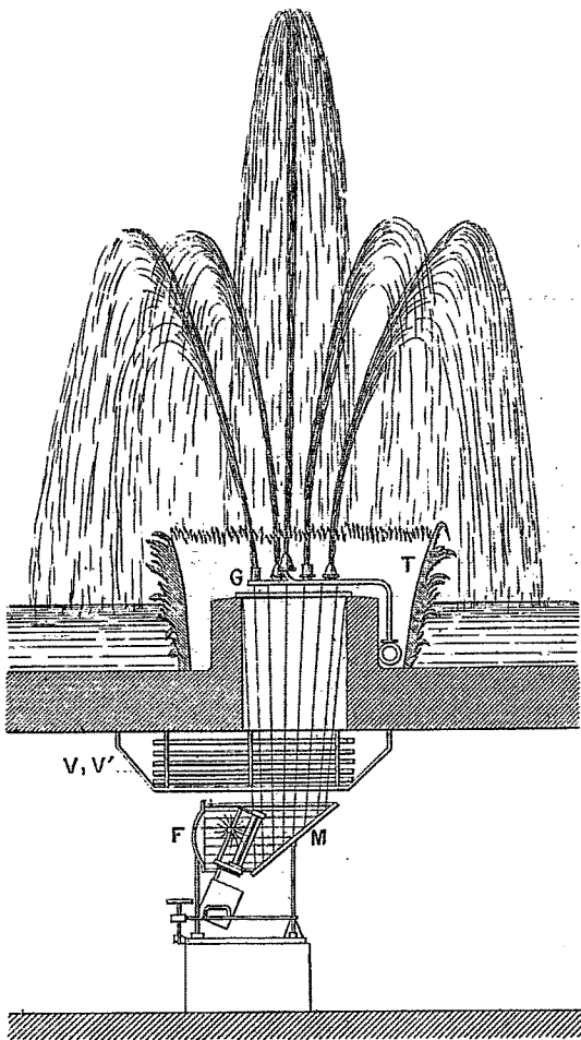
Coupe verticale de l'ensemble des fontaines. — A gauche, un des deux hommes d'équipe, placé dans une chambre souterraine au-dessous du bassin. — A droite, le chef d'équipe installé dans un pavillon élevé de trois mètres au-dessus du sol.
