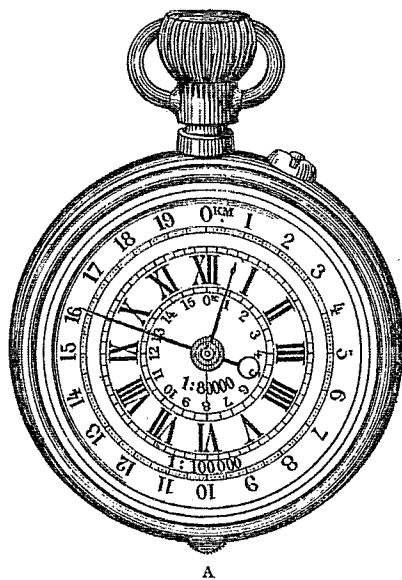
Fig. 1. — Montre avec curvimètre.
