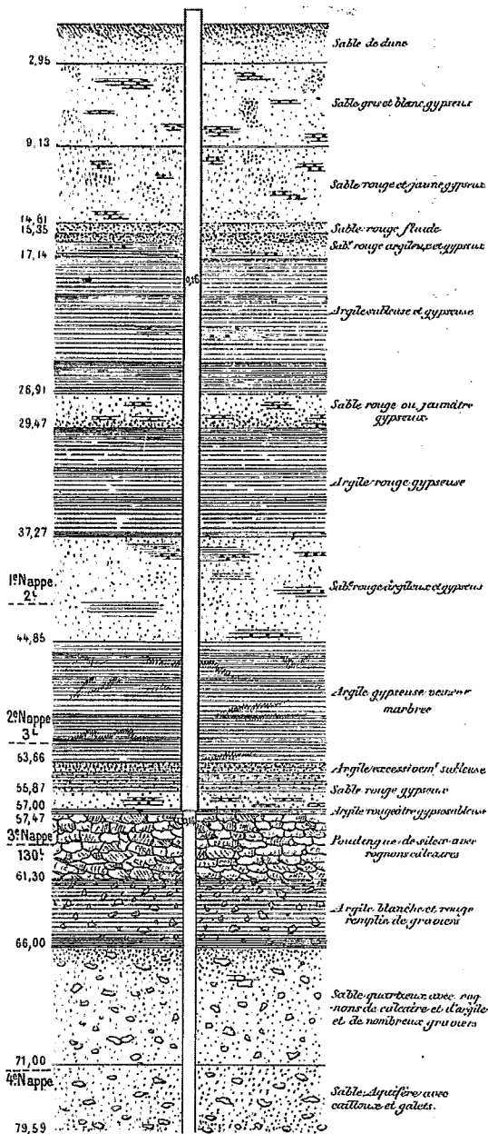
Coupe verticale du puits Séraphin, à Tigomime (Ourlana). — Débit total : trois mille litres par minute.
