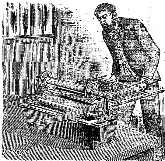
L'industrie des allumettes. — Machine servant à enduire l'extrémité des allumettes d'un bouton de pâte phosphorée.
