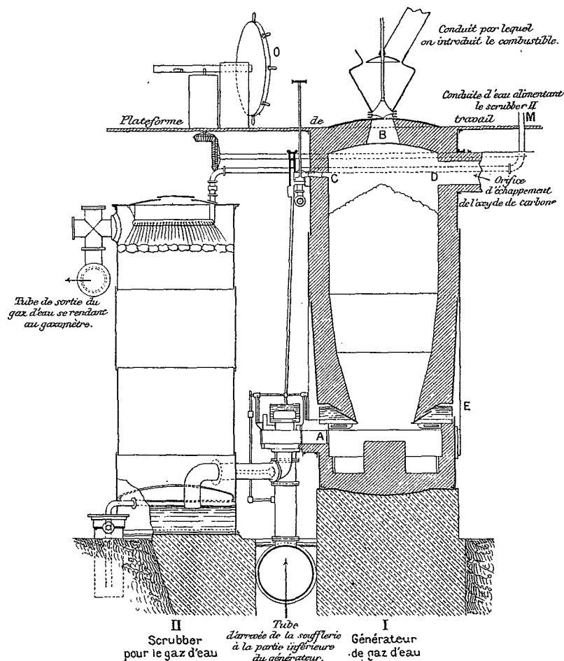
Appareil servant à fabriquer le gaz d'eau.
