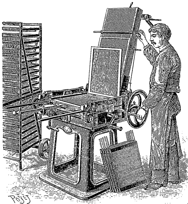
La fabrication des allumettes. — Machine à mettre les allumettes en presse.
