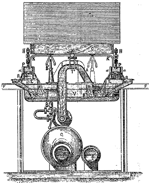
FIG. 5. — Coupe transversale du chemin de fer glissant. — A. Amortisseur. — B. Robinet de manœuvre du propulseur. — B' Tige du robinet. — C. Châssis du wagon. — D. Conduite pour recueillir l'eau des patins. — E. Conduite principale d'eau sous pression. — E'. Conduite de retour d'eau. — F. Fer du plancher de la voie. — H. Tige de suspension du wagon. — I. Buse du propulseur. — K. Tuyau d'eau sous pression pour l'alimentation des patins. — L. Lougrine en sapin qui supporte le rail. — M. Maneton de la tige du robinet de manœuvre. — P. Patin hydraulique. — Q. Accumulateur placé sur la conduite principale. — R. Rail. — S. Propulseur. — T. Turbine double rectiligne. — V. Bâche ou canal collecteur qui recueille toute l'eau dépensée. — a. Guide du patin. — c. Cylindre du propulseur. — p. Piston du propulseur.
