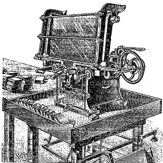
L'industrie des allumettes. — Machine à remplir d'allumettes les boîtes-portefeuilles.
