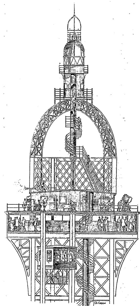
La tour Eiffel. — Coupe verticale de la partie supérieure de la tour.
