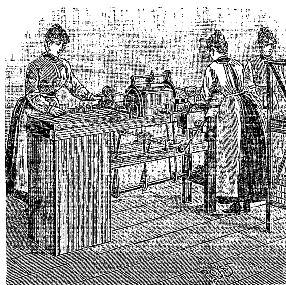
L'industrie des allumettes. — Machine à gratiner les boîtes d'allumettes. — Ensemble de la machine.
