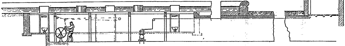
Coupe verticale de l'ensemble des fontaines. — A gauche, un des deux hommes d'équipe, placé dans une chambre souterraine au-dessous du bassin. — A droite, le chef d'équipe installé dans un pavillon élevé de trois mètres au-dessus du sol.
