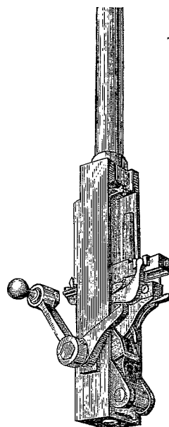
FIGURE 4. — Mitrailleuse Maxim. — Mécanisme de emeture.
