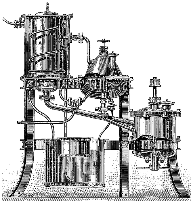
La fabrication des allumettes. — Machine à fabriquer le phosphore.
