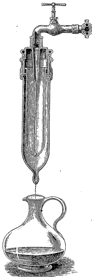
Aéri-filtre Mallié.
