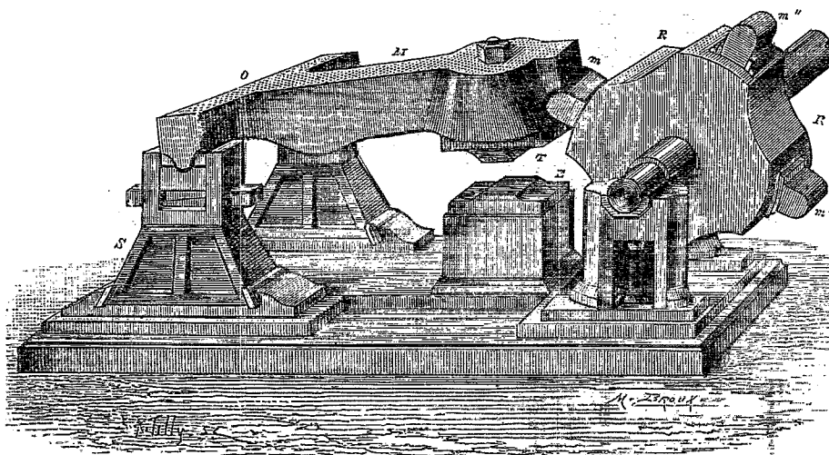
Marteau frontal.
