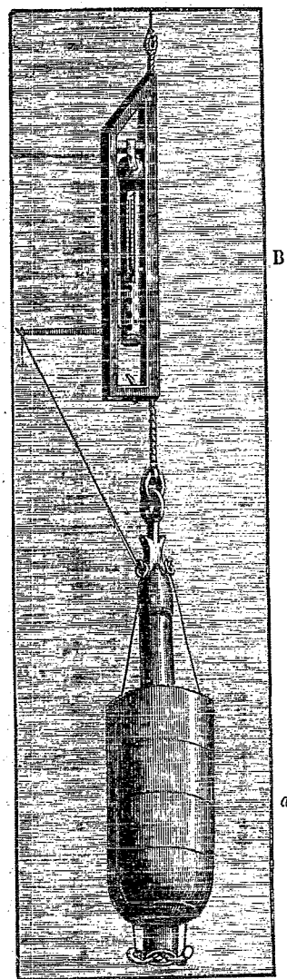
FIG. 1. a Sondeur. B Thermomètre du Talisman .
