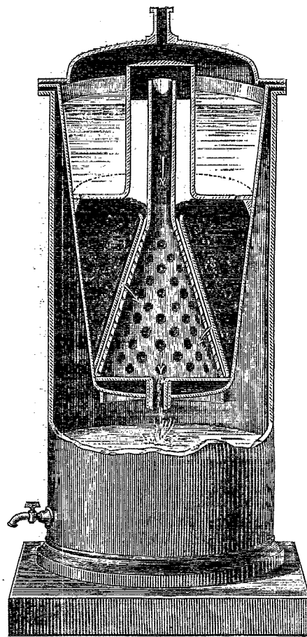
Filtre de ménage, système Maignen.
