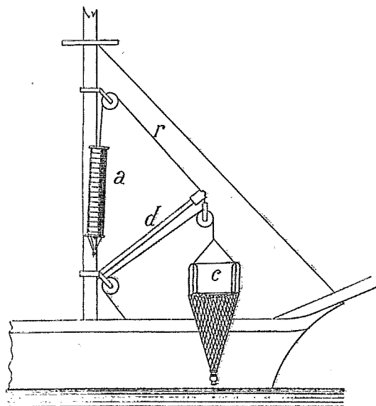
Schéma de l'accumulateur et du mode de suspension du chalut. a, accumulateur. — d, espar. — c, chalut. — r, pantoire.
