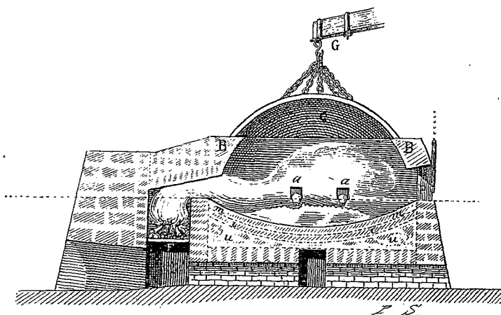
FOURNEAU DE COUPELLE. — F, foyer. — m m , coupelle formée de plusieurs lits de cendre et d'argile bien battue ( u u , i i ). — a a , tuyères des soufflets. — P, cheminée. — B B, voûte de la coupelle. — C, couvercle de fer garni de terre réfractaire, manœuvré par une grue G.
