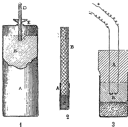
1 Cartouche amorcée : A cartouche de parchemin, B dynamite, C capsule, D mèche, E ligature réunissant la mèche à l'enveloppe de parchemin. — 2. Capsule avec mèche : A étui de cuivre, B mèche Bickford, C fulminate de mercure. — 3. Capsule avec conducteurs électriques : a a conducteurs, A soufre et verre pilé, B fulminate, C poudre au chlorate, I enveloppe de cuivre.
