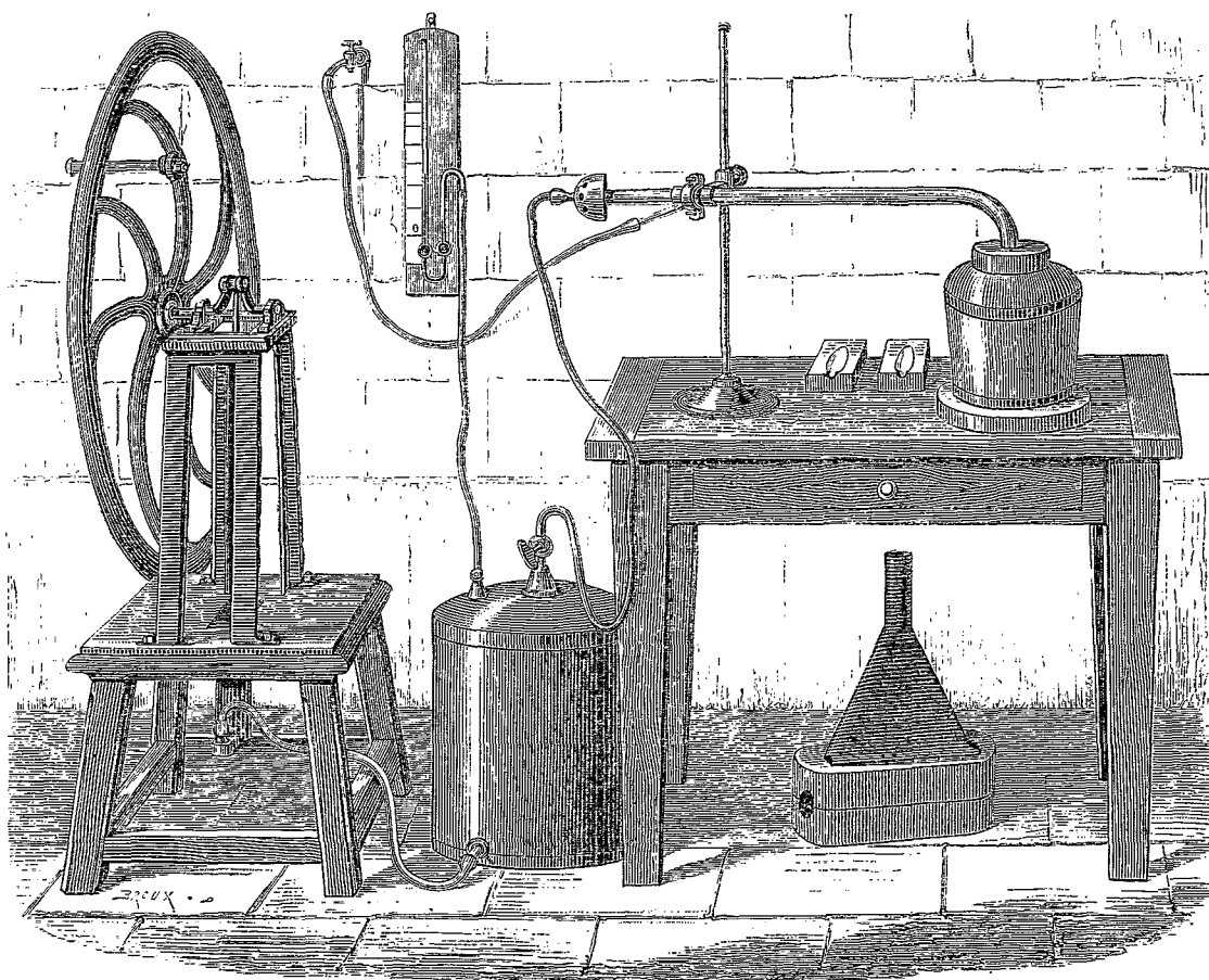
FIG. 1. — Chalumeau Schloësing. — Pompe foulante. — Dessin de Broux.
