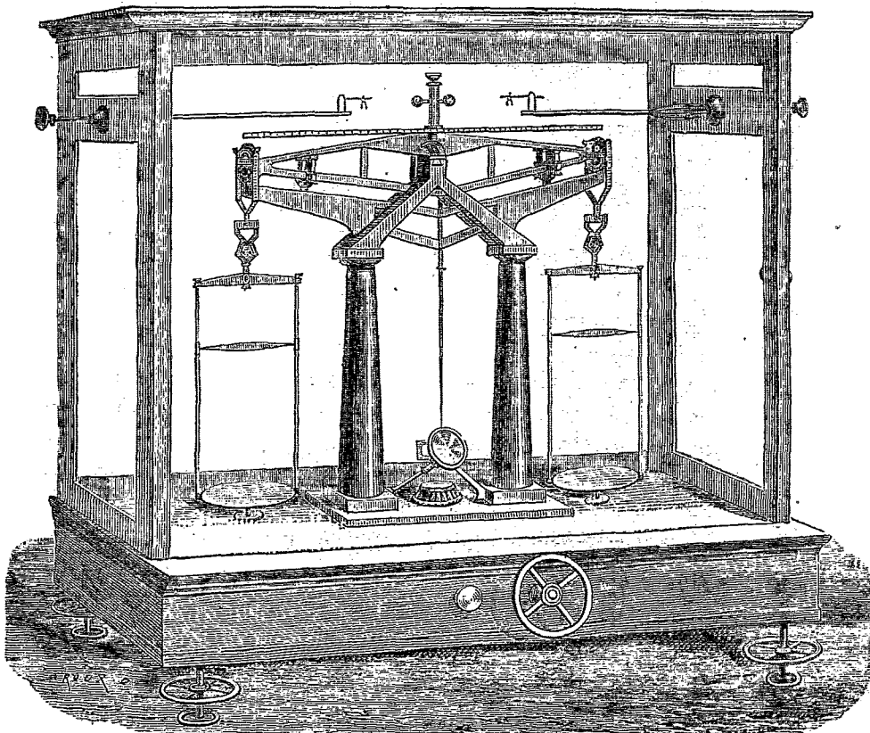
Balance de précision. — Dessin de Broux.
