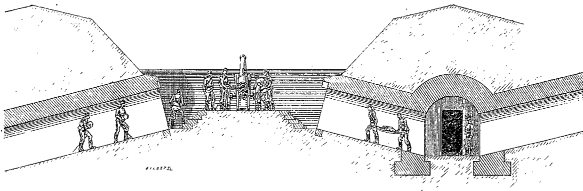
Mode de disposition des traverses-abris sur le rempart.
