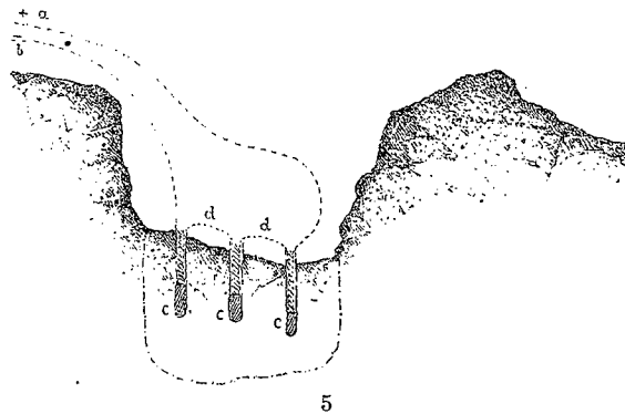
5. Disposition de trois charges devant partir ensemble : a conducteur positif, b conducteur négatif, c c c trois charges, d d fils de jonction.
