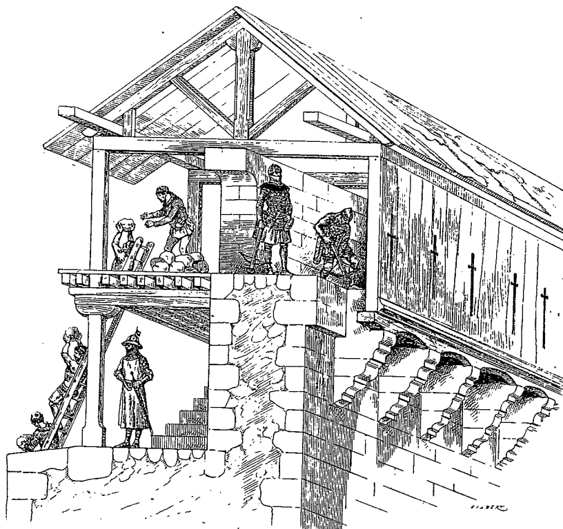
FIG. 4. — Hourd du quatorzième siècle. — Dessin de Gilbert.
