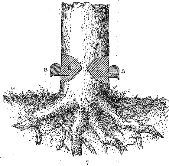
7. Abatage d'un arbre : BB boudin de dynamite, EE partie enlevée par l'explosion.
