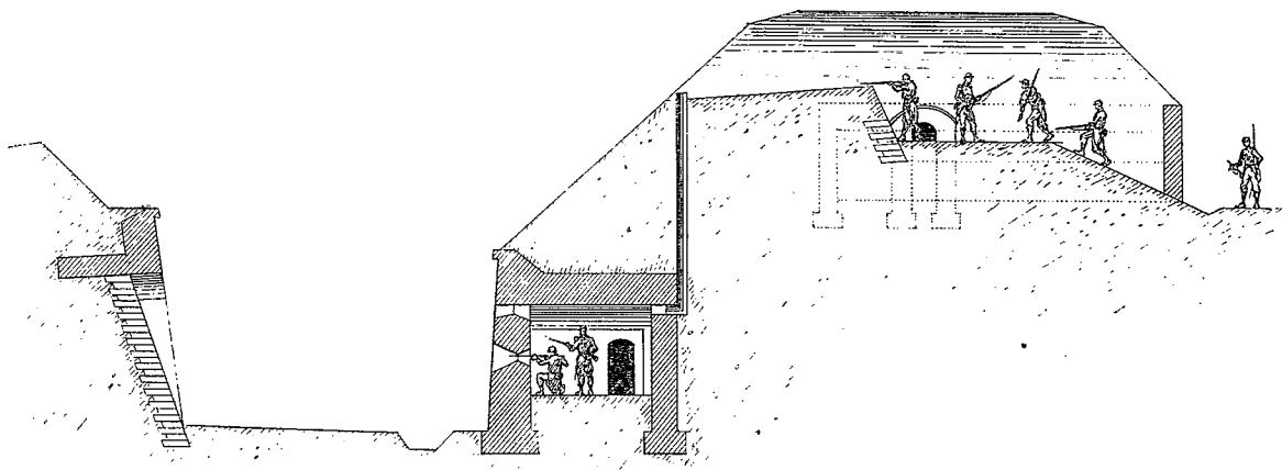
Coupe du rempart d'un fort d'enceinte sans cavalier.
