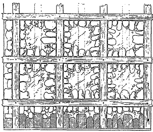
FIG. 1. — Fortifications gauloises au temps de Jules César. Plan d'un mur d'escarpe.
