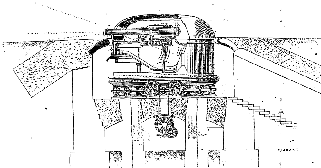
Tourelle cuirassée à coupole.
