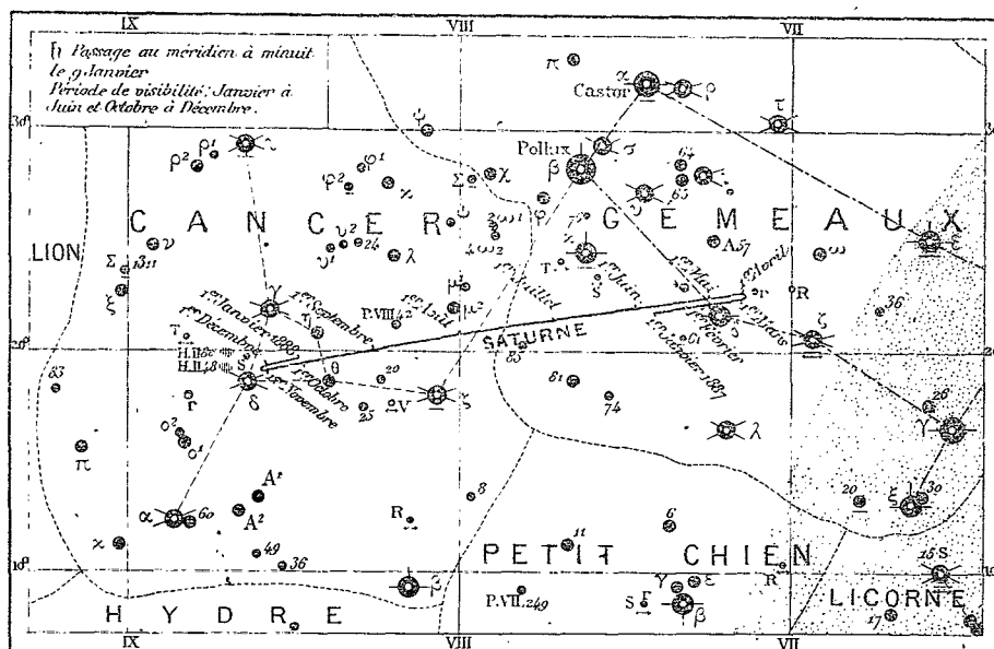
Marche et positions de Saturne pendant l'année 1887.
