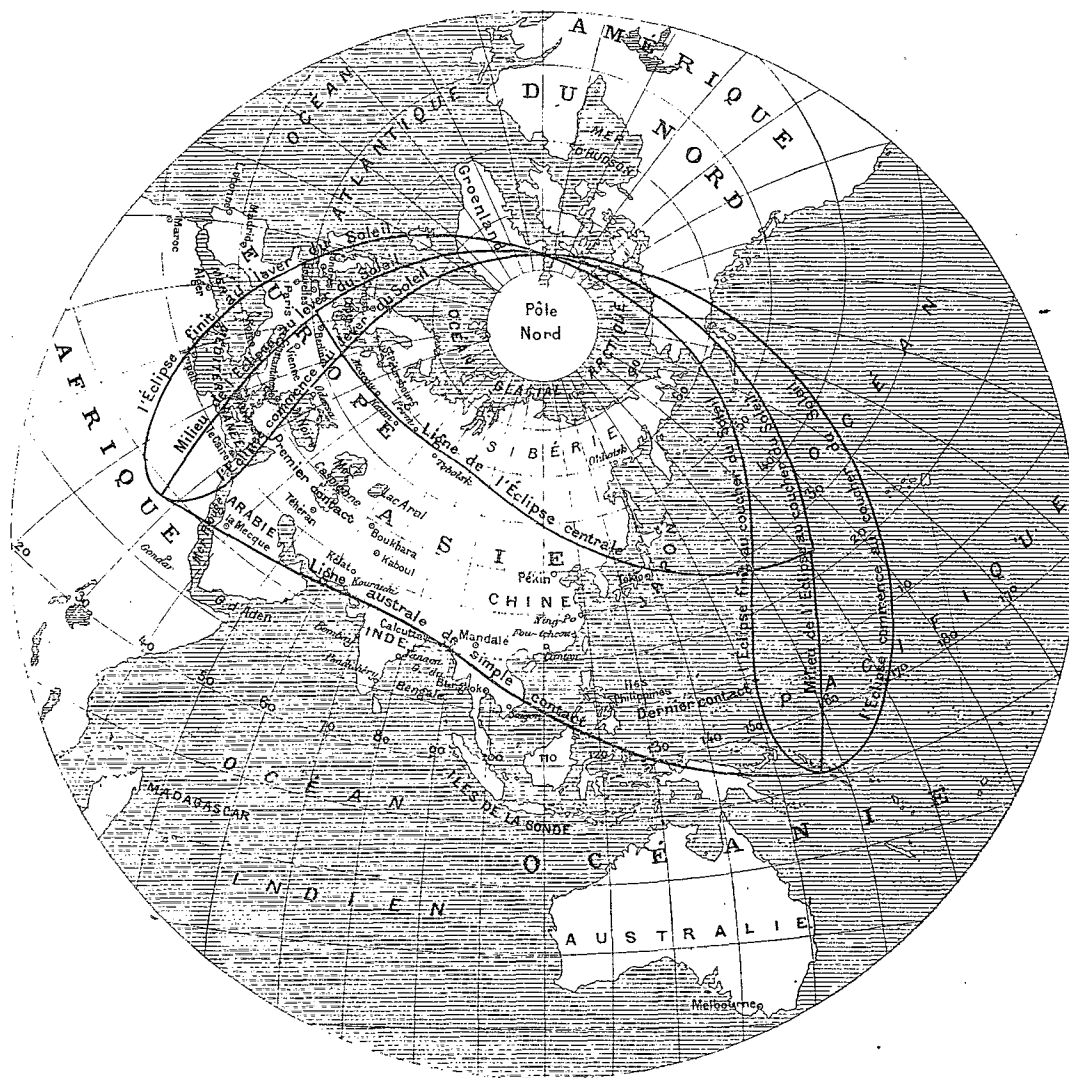
Marche de l'ombre de la Lune sur le globe pendant l'éclipse totale de Soleil du 19 août 1887.
