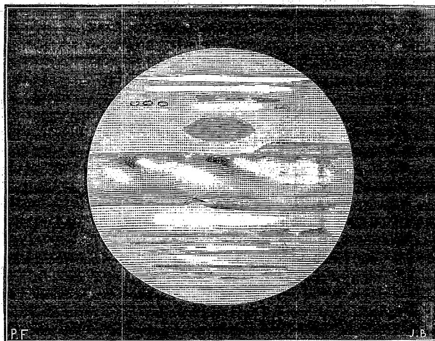
Jupiter et sa tache rougeâtre.
