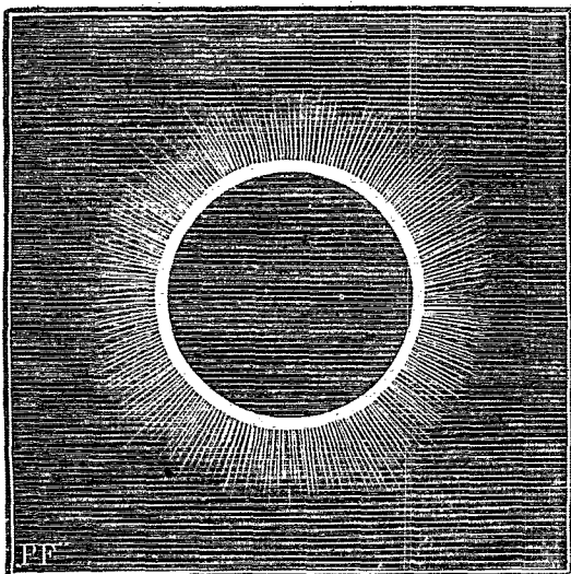
Éclipse annulaire de Soleil du 22 février 1887.
