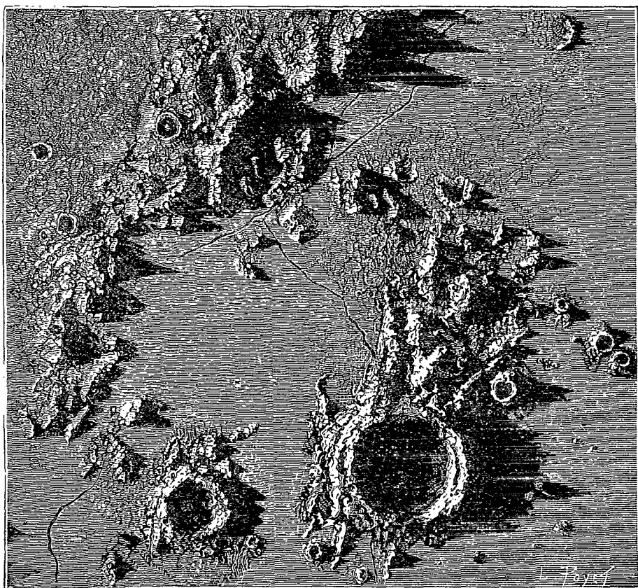
Paysage lunaire. — D'après une photographie.
