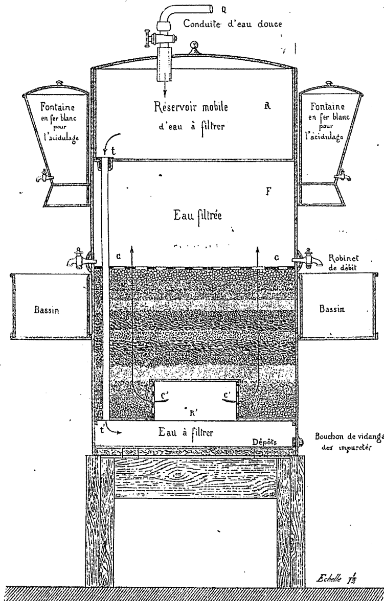
CONSTRUCTION D'UN FILTRE DE 1 m .20 DE HAUTEUR ET DE 0 m .60 DE DIAMÈTRE.
