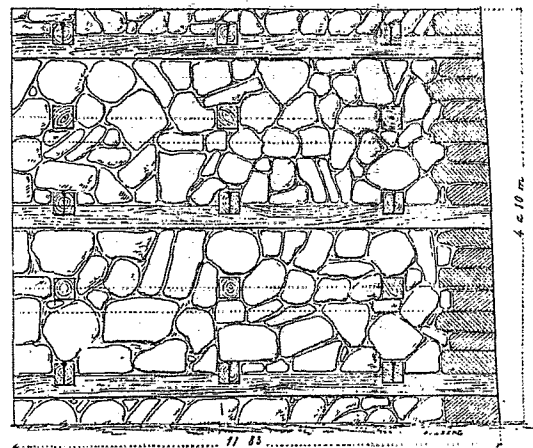
FIG. 2. — Profil du mur.
