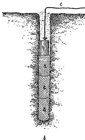
4 Chargement d'un trou de mine : a a a cartouches, b, cartouche amorcée, C mèche Bickford, d sable de bourrage.
