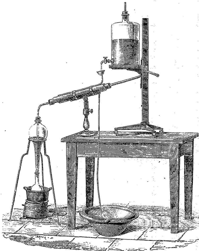
FIG. 2. — Appareil à épuisement de Cloëz. — Dessin de Broux.
