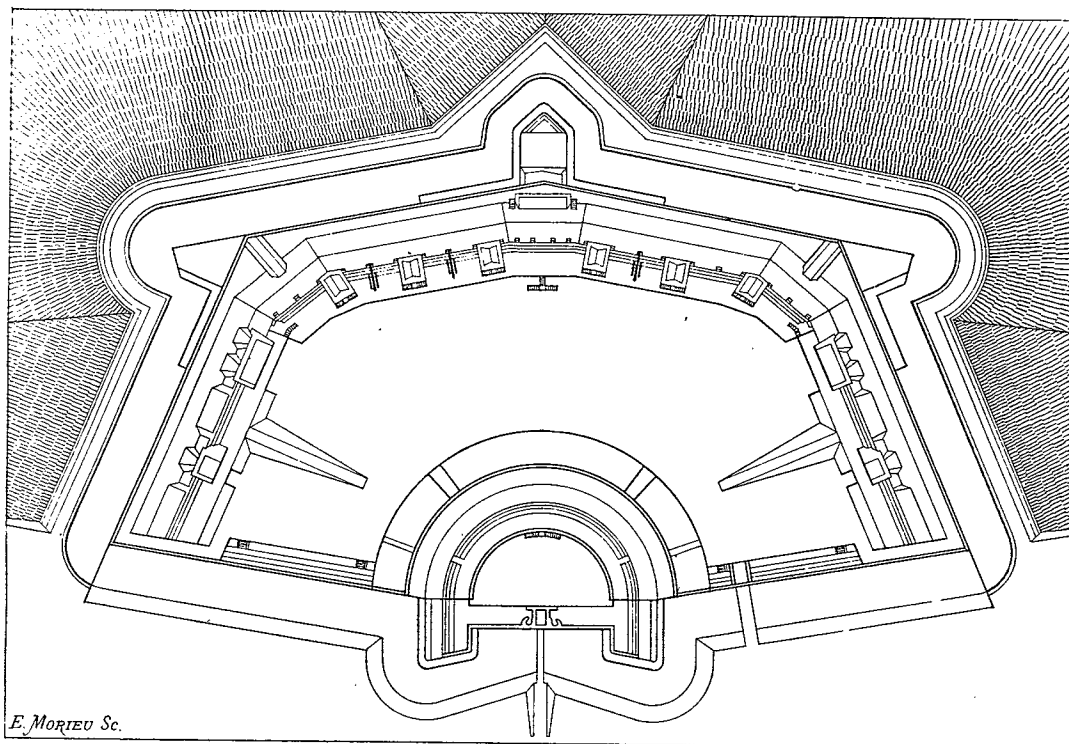
Prototype de fort d'enceinte. — Plan d'ensemble d'un des forts de Gosport (Portsmouth).
