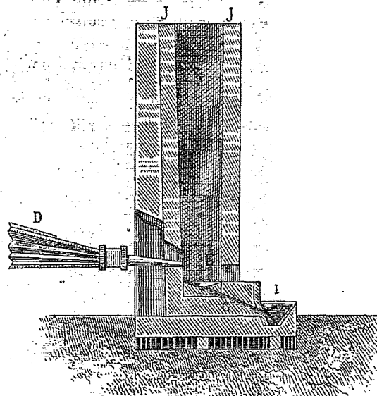
FOURNEAU A MANCHE. — J J E, cuve dans laquelle on entasse le charbon et le minerai grillé. — D, soufflet (en espagnol, mancha , d'où le nom du fourneau). — G, conduit par lequel le plomb s'écoule dans le bassin I ménagé en devant du fourneau.
