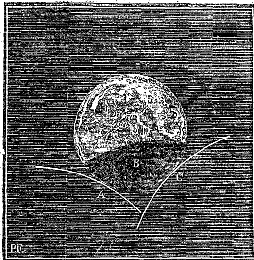
Éclipse partielle de Lune du 3 août 1887.
