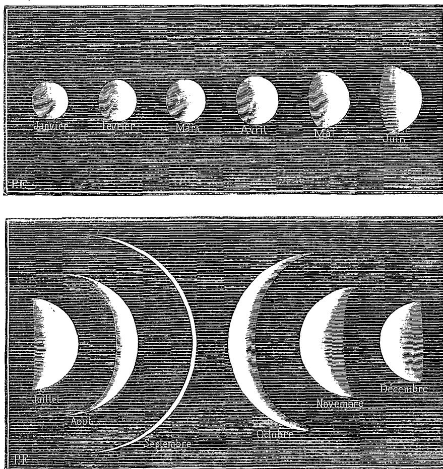
Phases de Vénus pendant l'année 1887.
