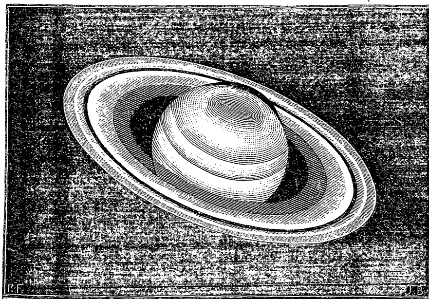
Aspect actuel de Saturne et de ses anneaux.
