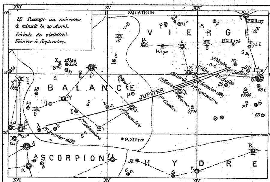
Marche et positions de Jupiter pendant l'année 1887.
