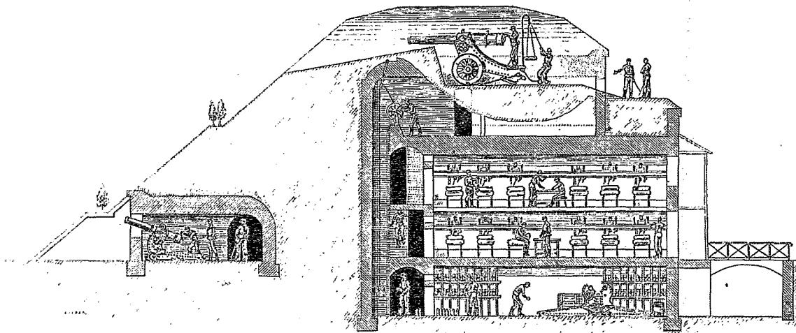
Coupe d'un cavalier de fort d'enceinte.
