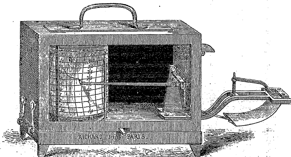
FIG. 3. — Thermomètre enregistreur.
