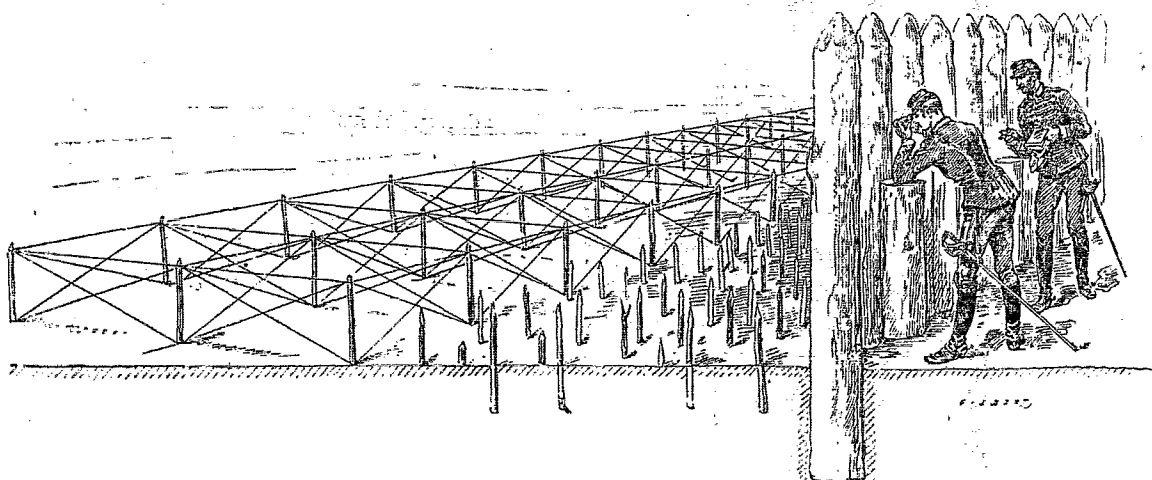
FIG. 7. — Palanques.
