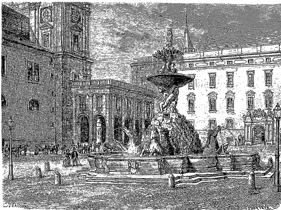
La Fontaine aux chevaux marins, à Salzbourg, par Antoine Dario (1664).
