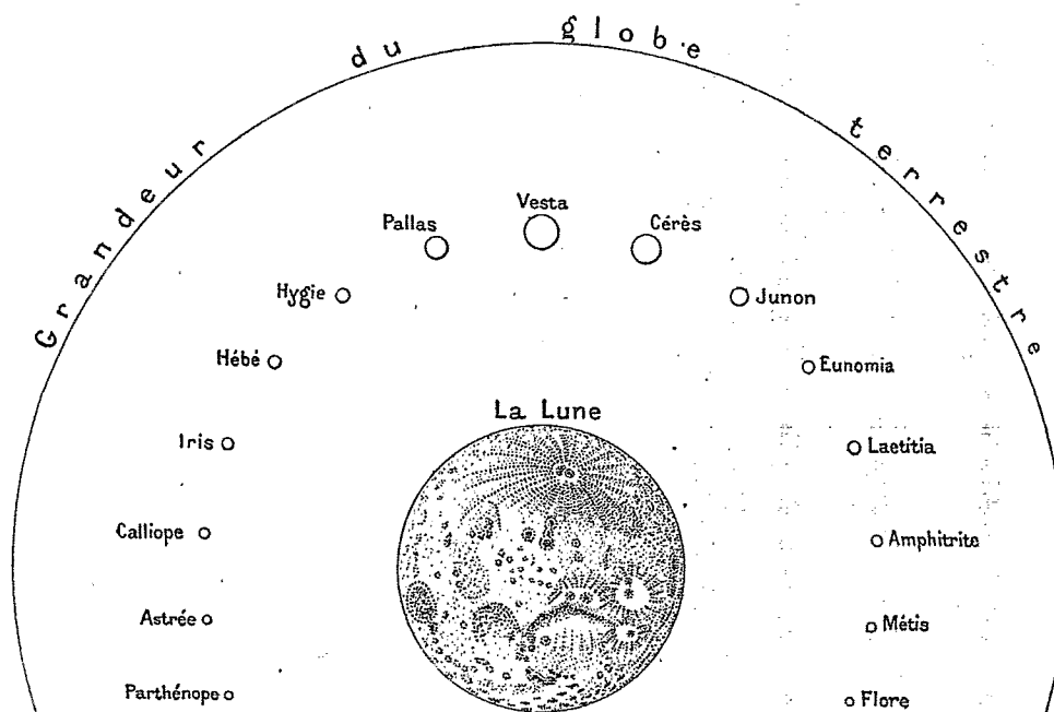
Grandeurs comparées de la Terre, de la Lune et des principales petites planètes. (Le cercle extérieur représente la dimension de la Terre.)
