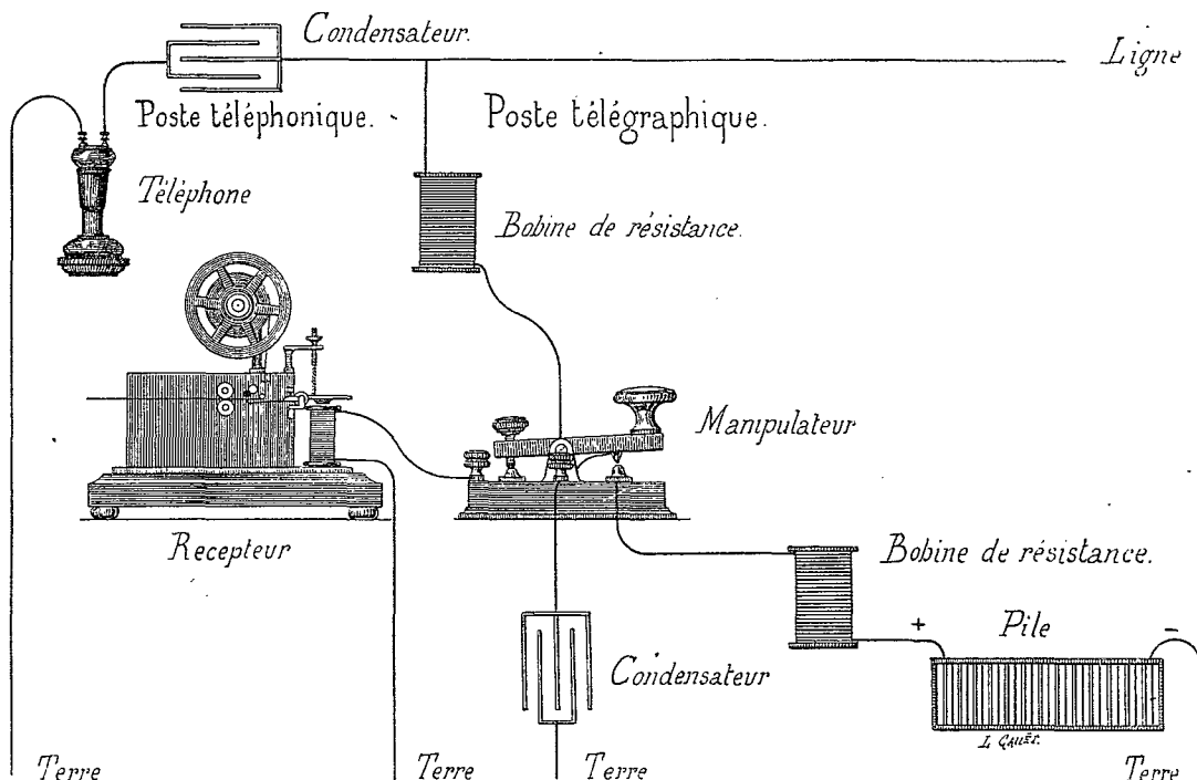
Télégraphie et Téléphonie simultanées. — Système de M. Van Rysselberghe.
