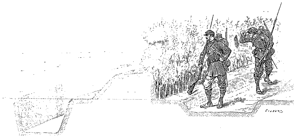
FIG. 12. — Haie vive organisée défensivement avec parapet et fossé.
