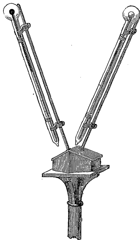
Actinomètre.
