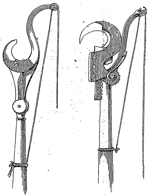
Échenilloir émondeur.
