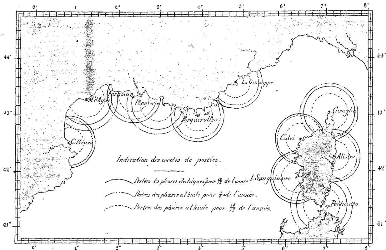
FIG. 1. — Portées de lumière des phares.
