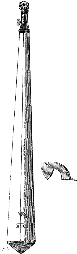
Trompette marine. — D'après l'ouvrage du P. Mersenne intitulé : l'Harmonie universelle (1636).
