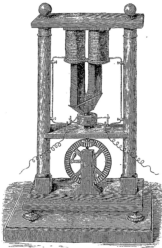
FIG. 2. — Machine dynamo-électrique de Pixii.
