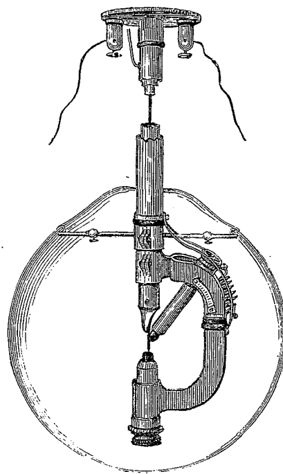
FIG. 4. — Lampe Reynier
