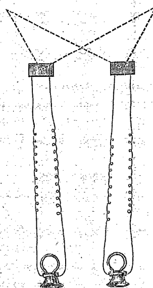
FIG. 3. — Diagramme des auditions théâtrales téléphoniques.
