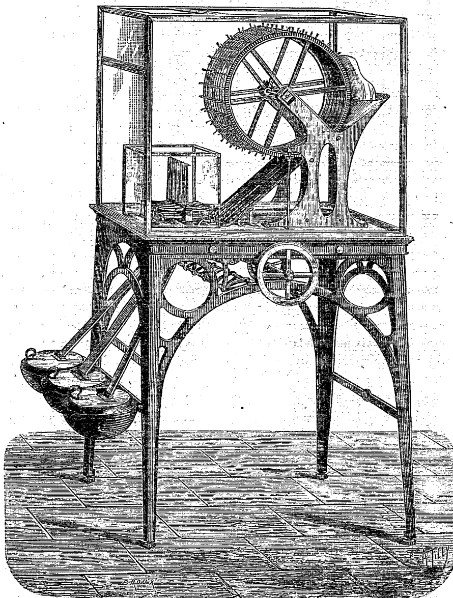
Balance automatique du baron Séguier, à la Monnaie de Paris.
