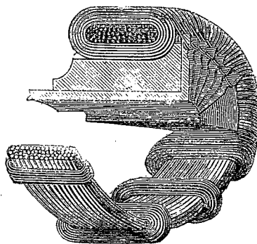
FIG. 6. — Coupe de la bobine Gramme.
