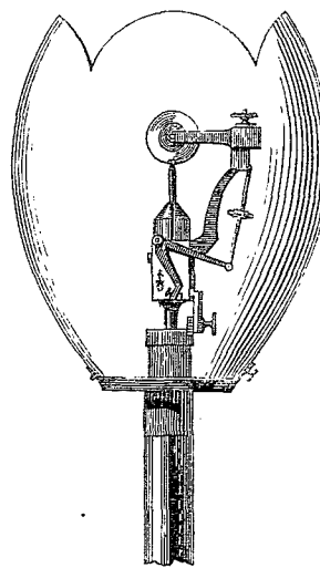
FIG. 4 bis. — Lampe Werdermann.
