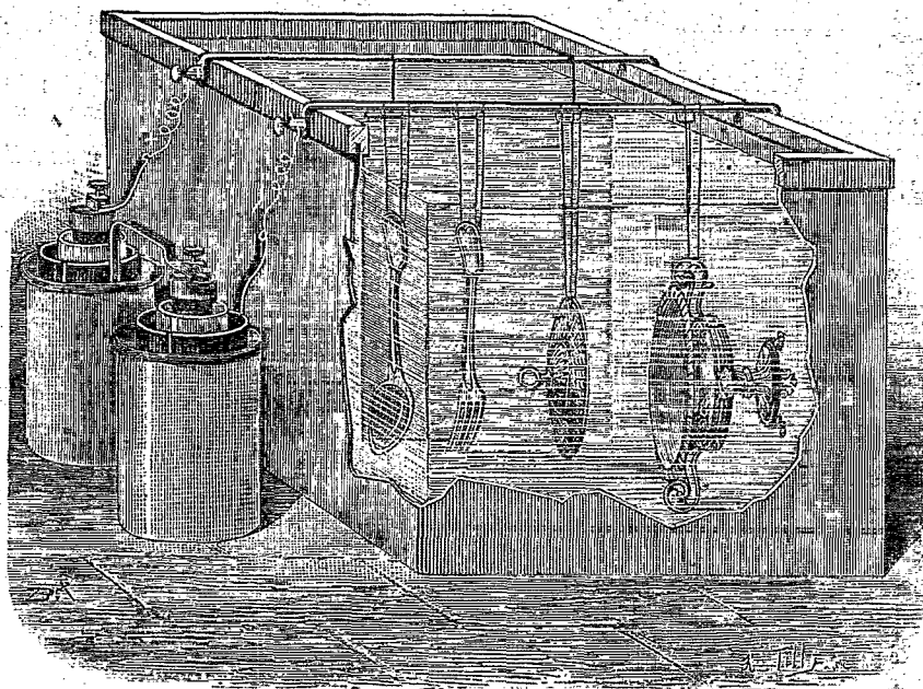
Appareil pour la nickelure galvanique.
