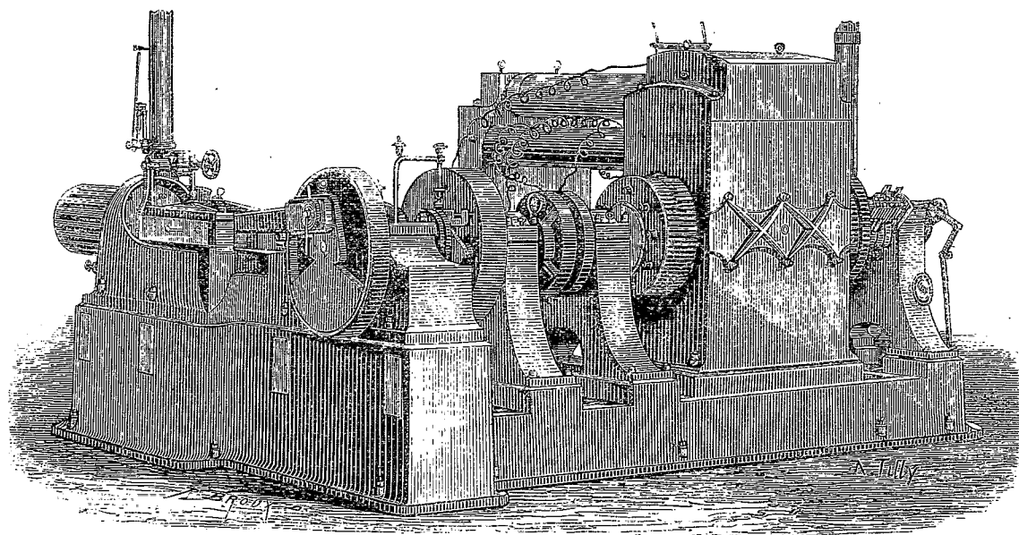
FIG. 7. — Machine électro-dynamique d'Edison.
