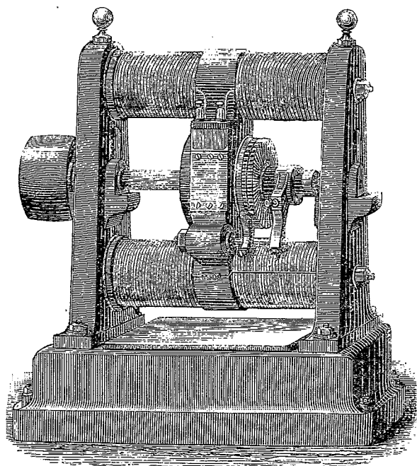
FIG. 5. — Machine Gramme.
