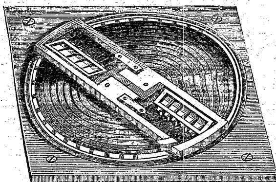
Fig. 2. — Combinateur électrique de M. Baudot.
