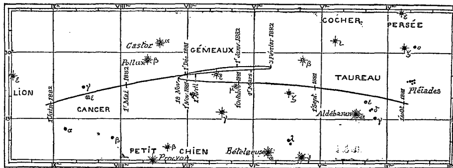
FIG. 4. — Mouvement et positions de la planète Mars.
