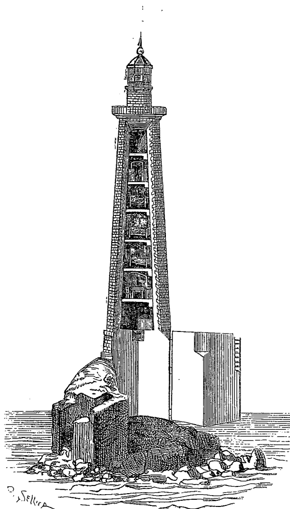
Coupe du Phare (voy. ci-contre, en a). — Dessin de Sellier.
