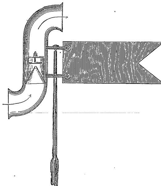
Aéroscope.
