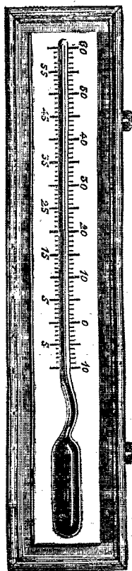
Thermomètre à maxima de Negretti et Zambra.
