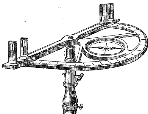
FIG. 3. — Graphomètre.
