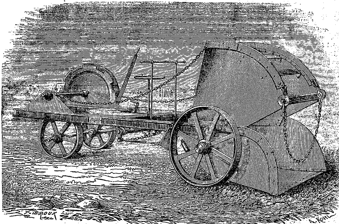
Le Steamscop, ou Écope à vapeur, de John Fowler.
