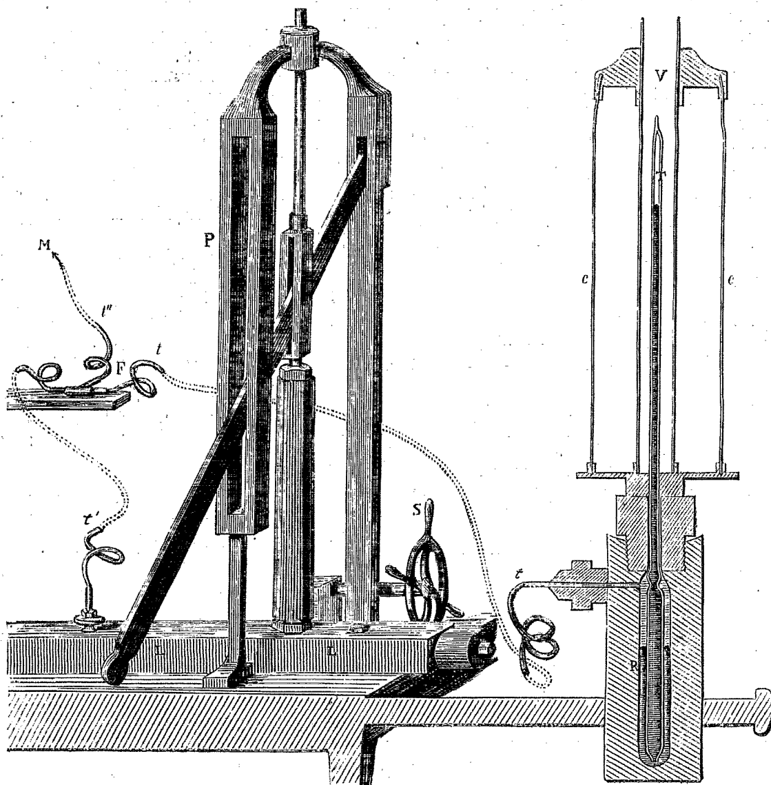
Appareil Cailletet pour la liquéfaction de l'air. — Dessin de G. Bonnier.
