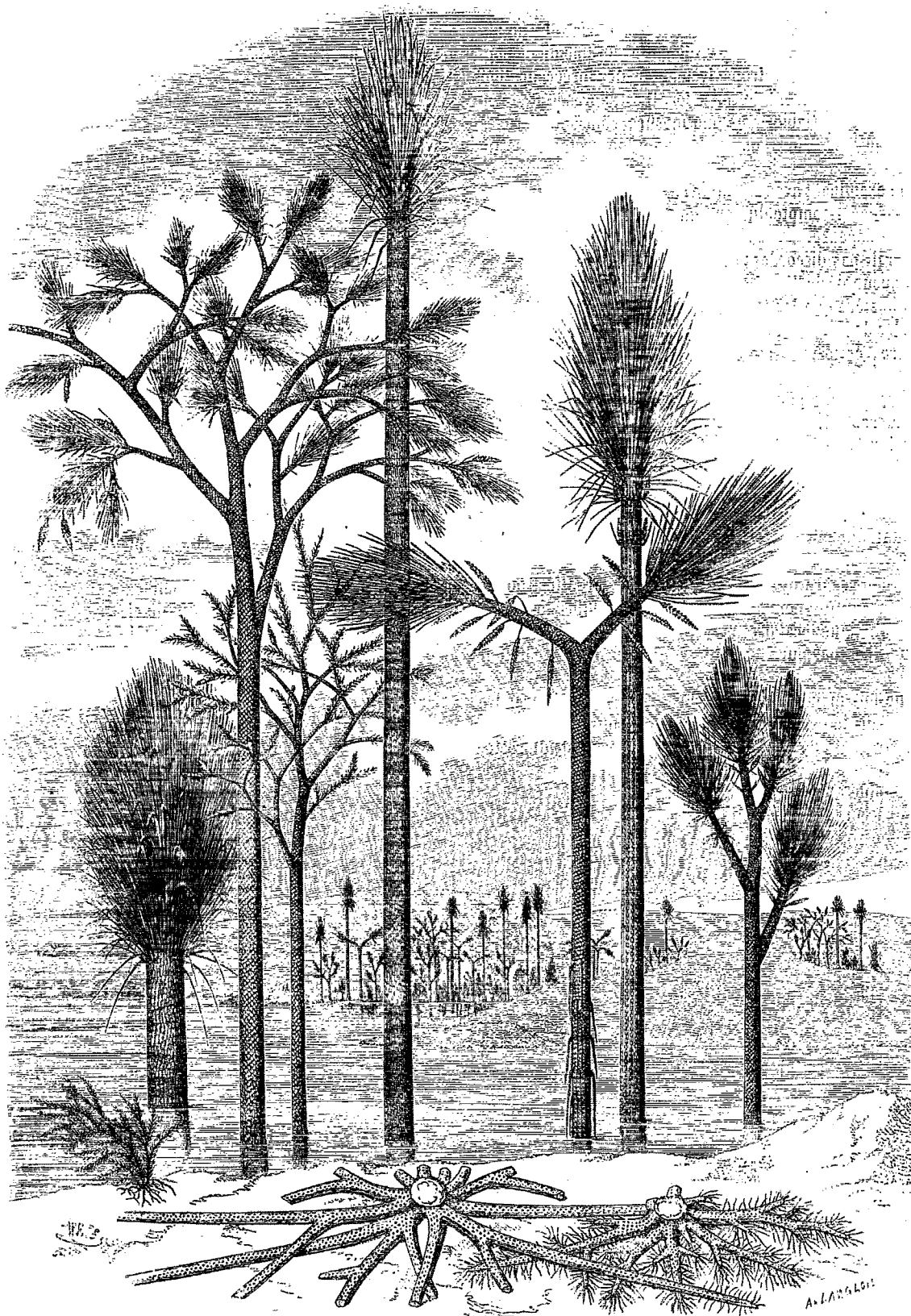
Lépidodendrées.
