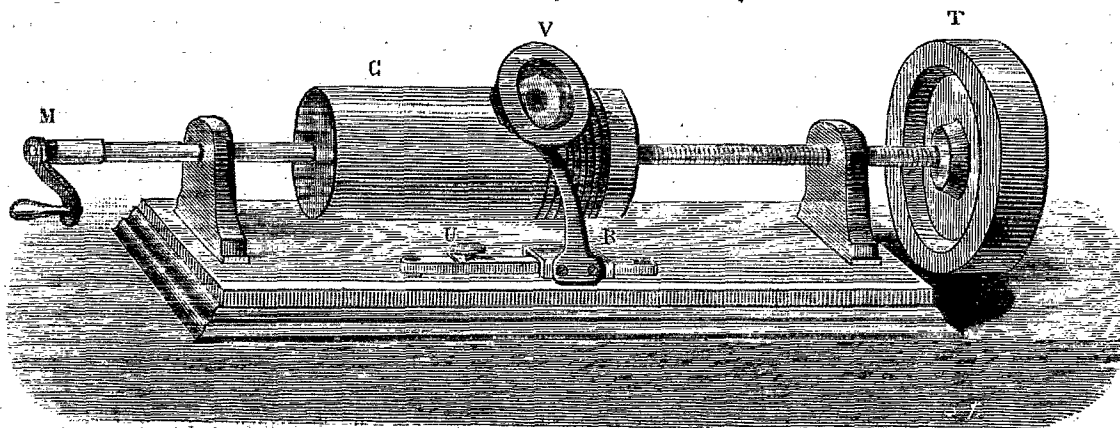
Le Phonographe, instrument qui conserve et reproduit les paroles.
