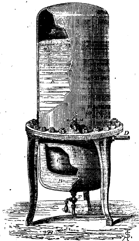
Filtre à air comprimé, système Chanoit.
