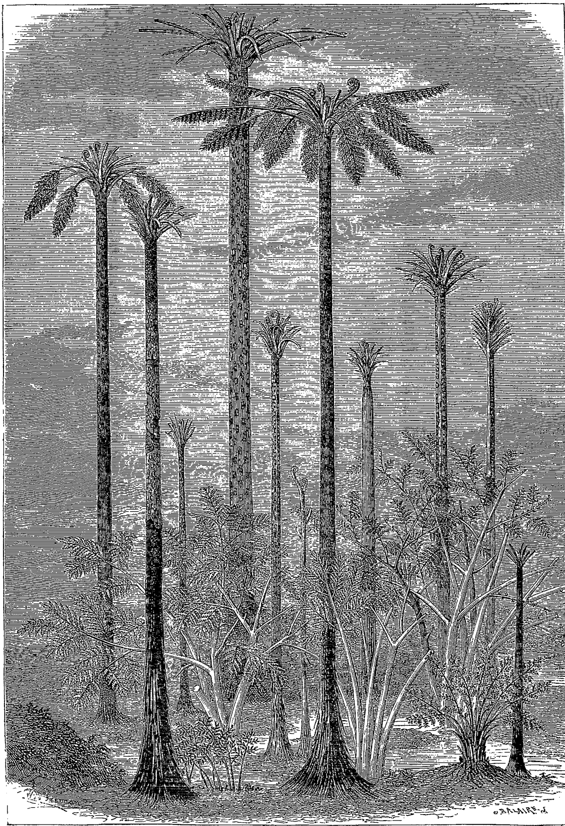
Pécoptridées.
