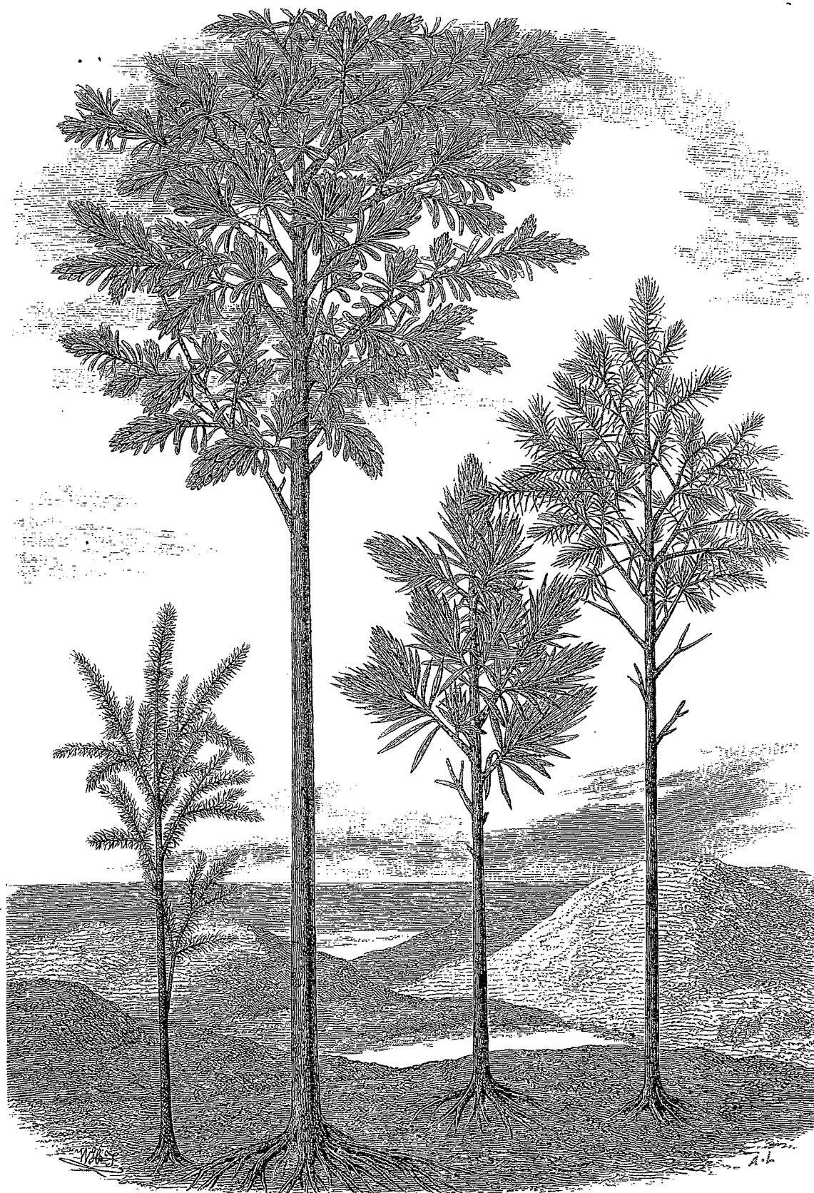
Dicranophyllum.
