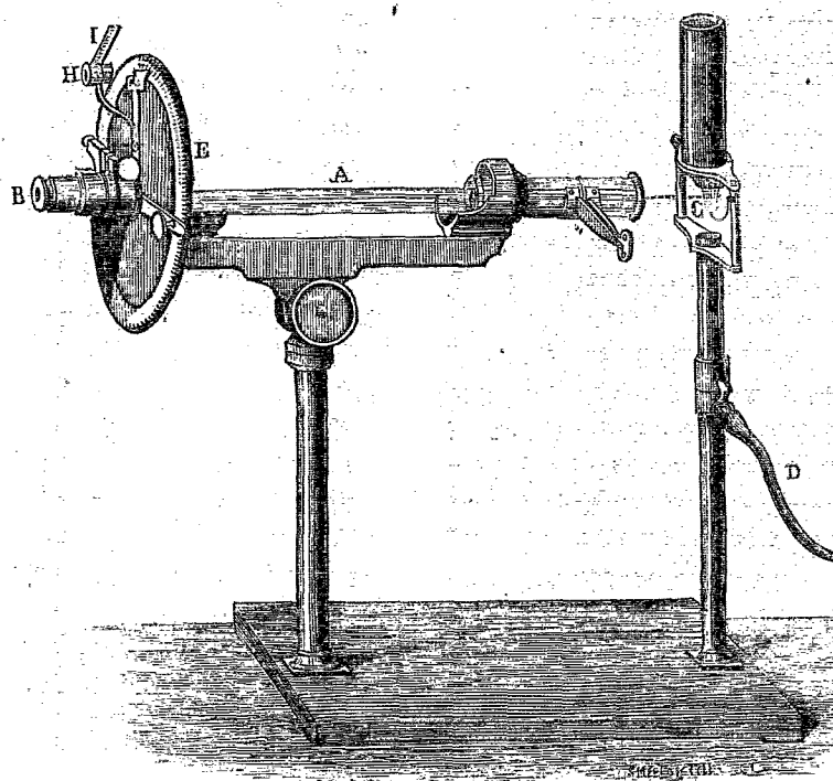
Le Saccharimètre.
