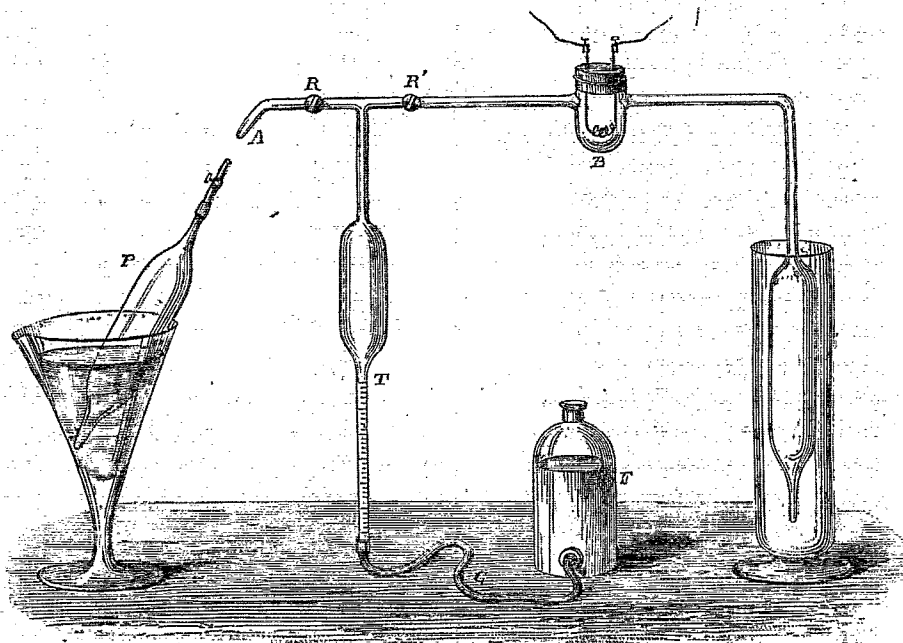
Grisomètre.
