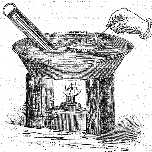
Appareil Mead pour l'essai du pétrole.
