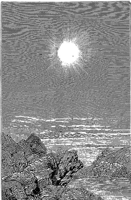
La Terre vue de Jupiter.
