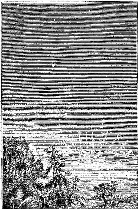
La Terre vue de Mars.
