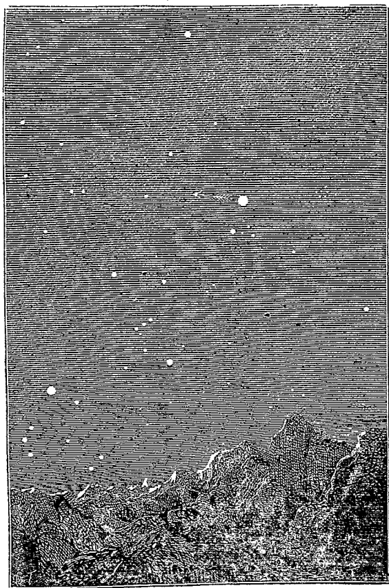
La Terre vue de Mercure.
