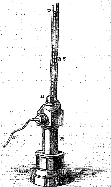
Nouveau Manomètre pour mesurer les hautes pressions.
