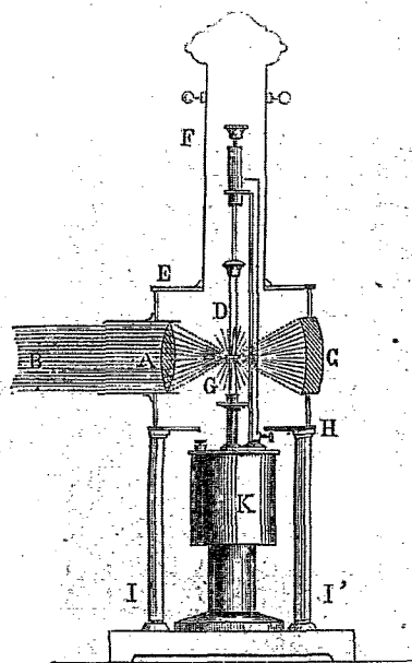
FIG. 3. — Coupe de l'appareil d'éclairage électrique.
