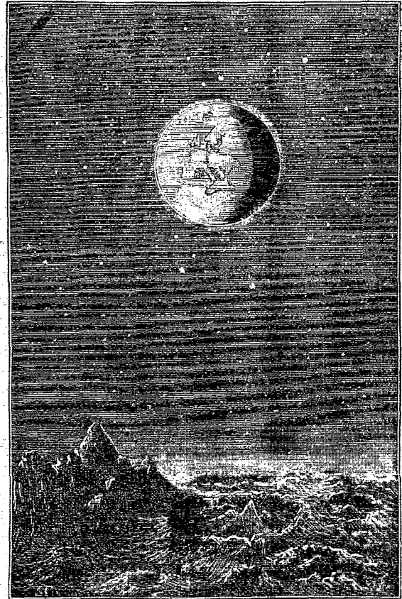
La Terre vue de la Lune.
