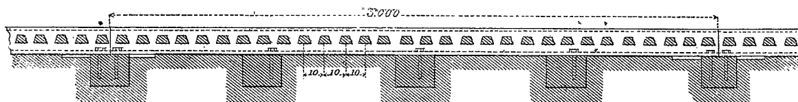
Coupe en long de la crémaillère.
