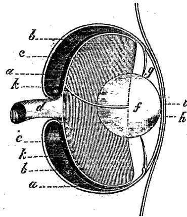
FIG. 6. — Détails de l'œil du poisson.
