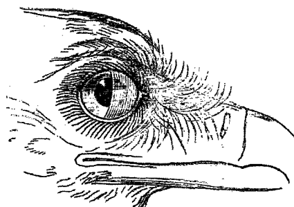
FIG. 4. — Œil du Secrétaire ou Serpentaire. — Cette figure montre la membrane clignotante à demi fermée.
