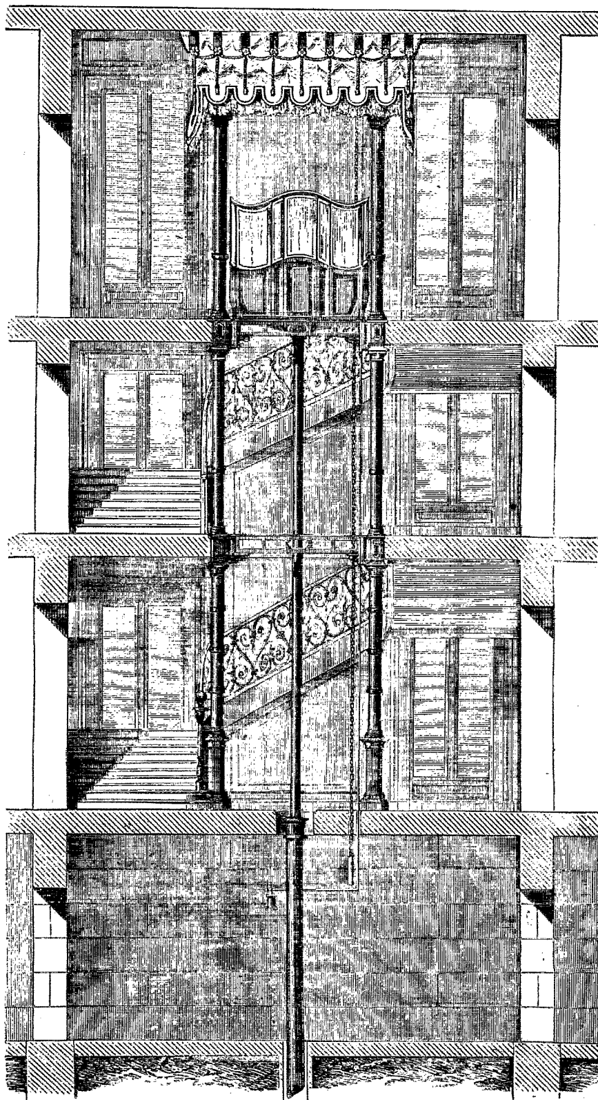
L'Ascenseur de l'hôtel du Louvre. — Dessin de Pérot.
