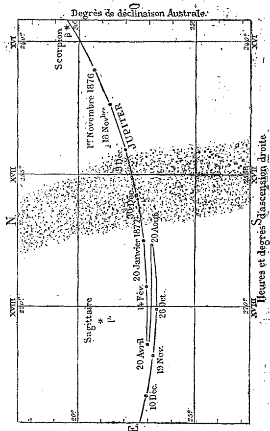
MOUVEMENT ET POSITIONS DE JUPITER pendant l'année 1877.
