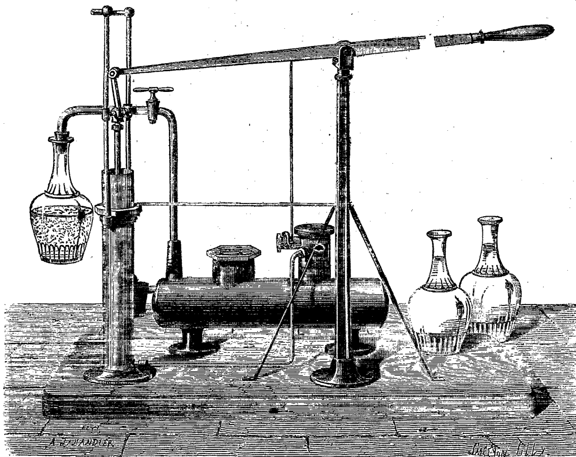
Appareil Carré pour frapper les carafes. — Dessin de Jahandier.
