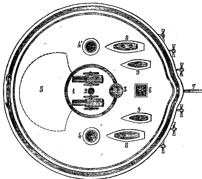
La Popoffka, nouveau garde-côtes russe. — Plan.
