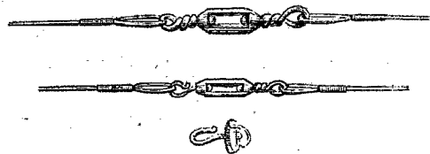
FIG. 28, 29, 30. — Émérillons divers.
