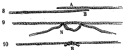
Fig. 8, 9, 10. — Nœud de pêcheur. — A, B, les deux bouts en présence; N, le nœud préparé; R, le nœud serré.
