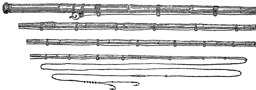
FIG. 1. — Canne en bambou à moulinet; quatre brins.
