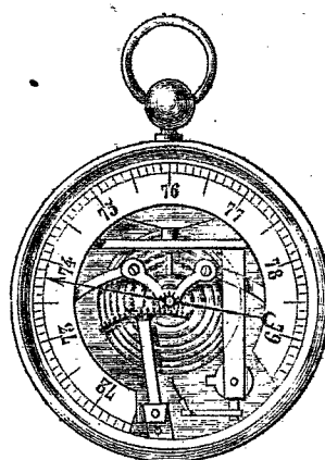
Baromètre Bréguet.
