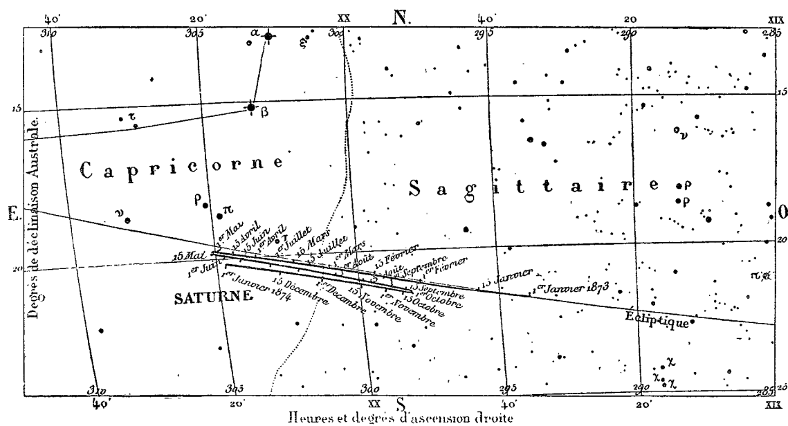
Mouvement et positions de Saturne pendant l'année 1873.
