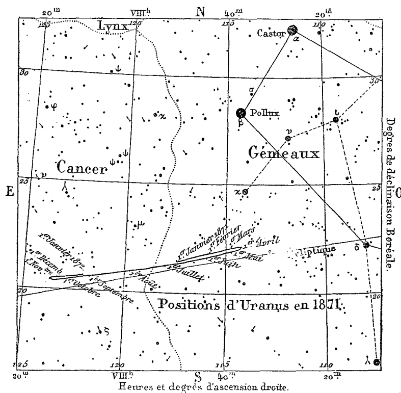
MOUVEMENT ET POSITIONS D'URANUS pendant l'année 1871.
