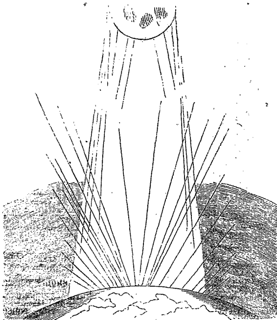
Influence des rayons de la Lune.
