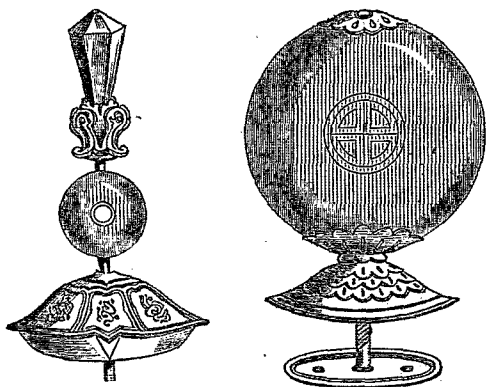
Globules se vissant au chapeau.
