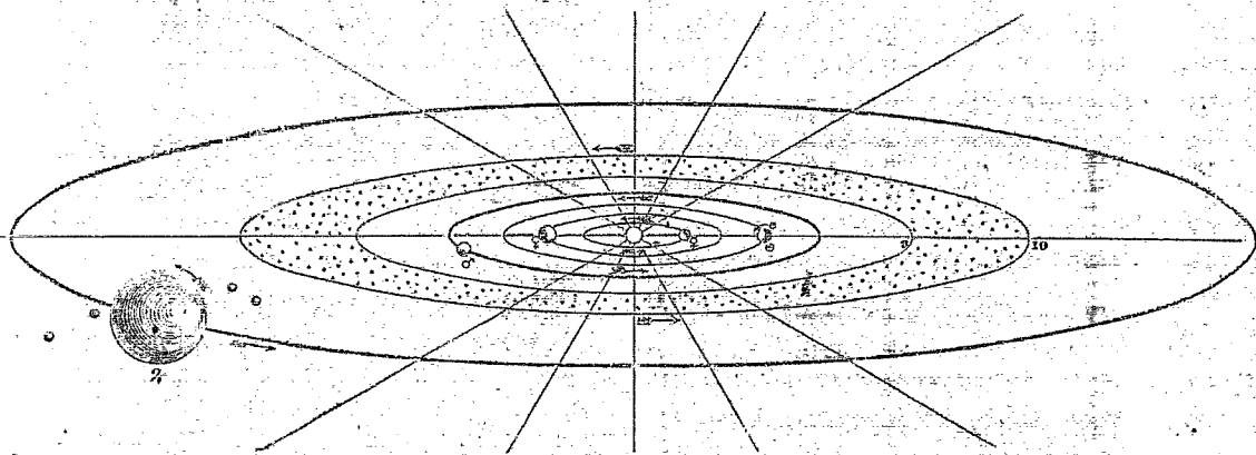
Orbites de Jupiter et des petites planètes.
