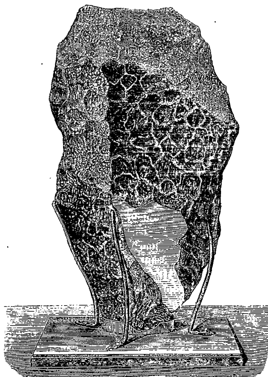
FIG. 1. — Fer météorique du Mexique, pesant 780 kilogrammes.
