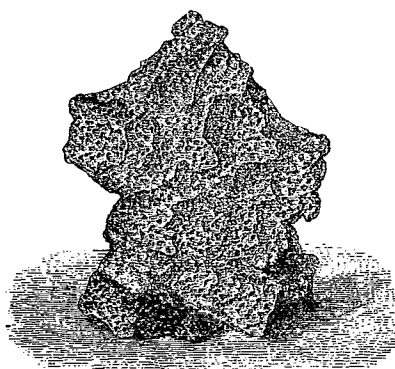
FIG. 3. — Aérolithe tombé au Chili.
