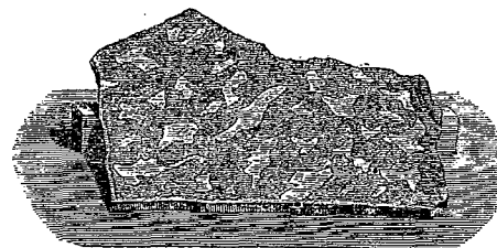
FIG. 6. — Aérolithe trouvé en Saxe.
