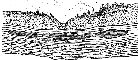
FIG. 3. — Amas métalliques.
