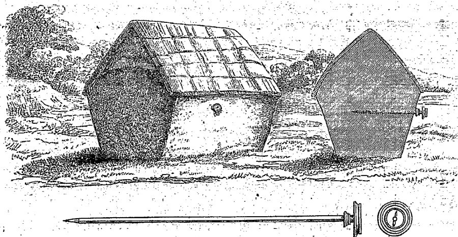
Pyromètre pour meules. — Dessin de Féart.
