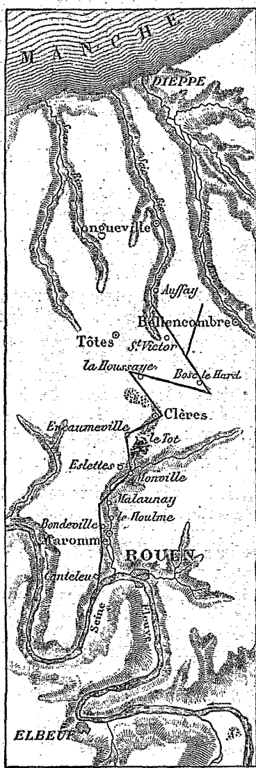
Marche de la trombe de Monville, en 1845.
