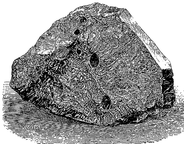
FIG. 2. — Fer météorique du Var ; poids, 591 kilogrammes.
