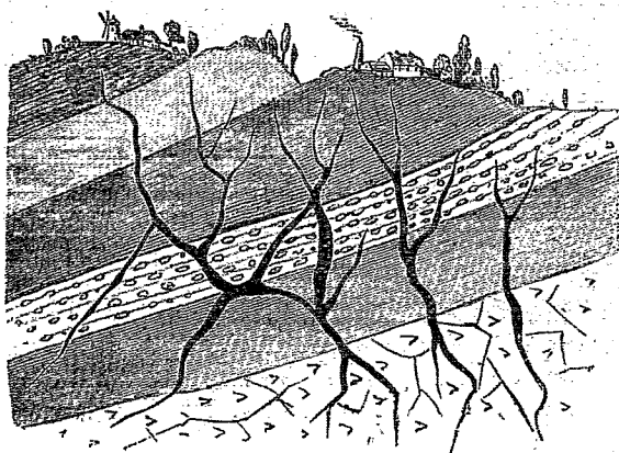
FIG. 1. — Filons croiseurs.
