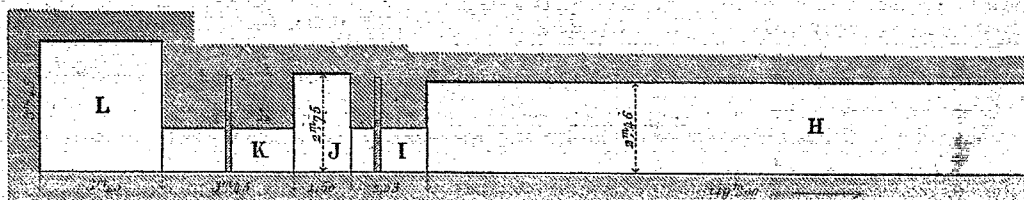
Coupe des entrées du Tombeau, de la grande galerie et du caveau sépulcral, à l'échelle de 5 millimètres pour 1 mètre.
