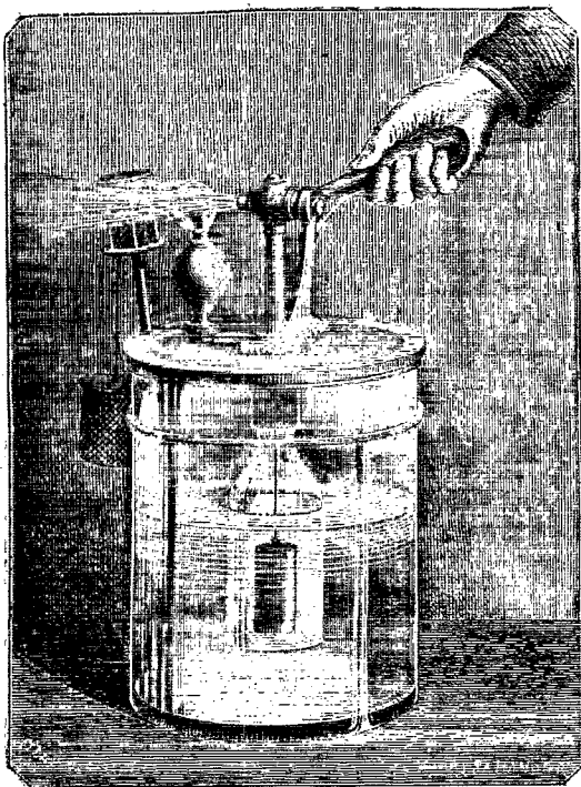
FIG. 3. — Briquet Gay-Lussac.
