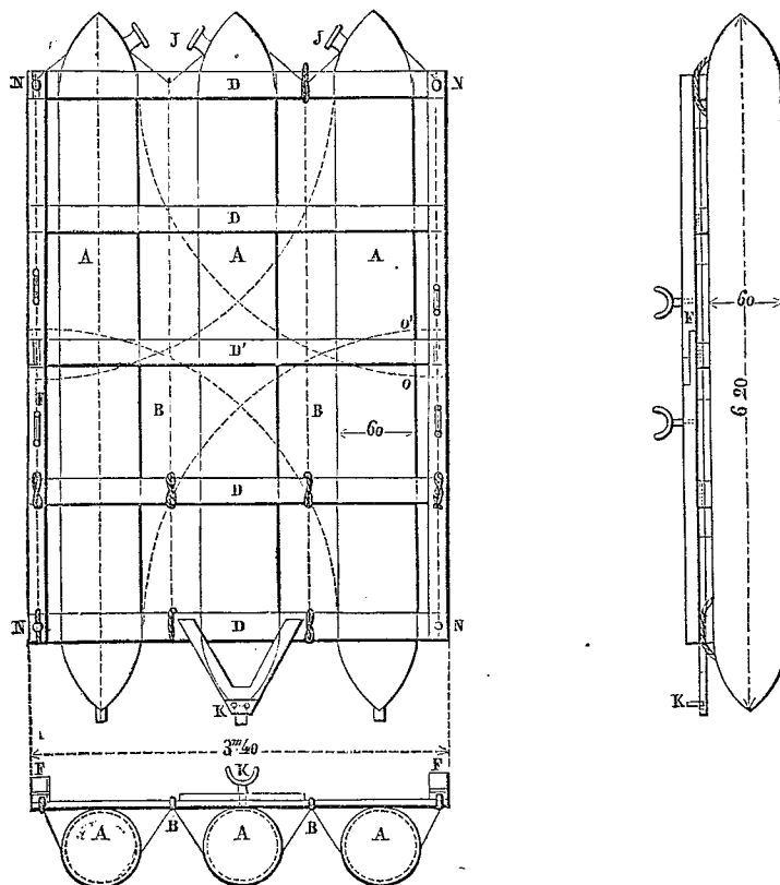
FIG. 4. — Radeau américain Perry; plan, coupe et projection latérale.
