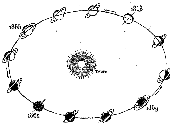
FIG. 1. — Variation perspective des anneaux de Saturne, et position de la Terre le 4 juin 1869.
