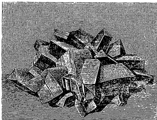
FIG. 5. — Forme cristalline du sulfate de cuivre.
