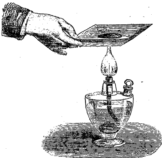
FIG. 2. — Étain fondu sur une carte.
