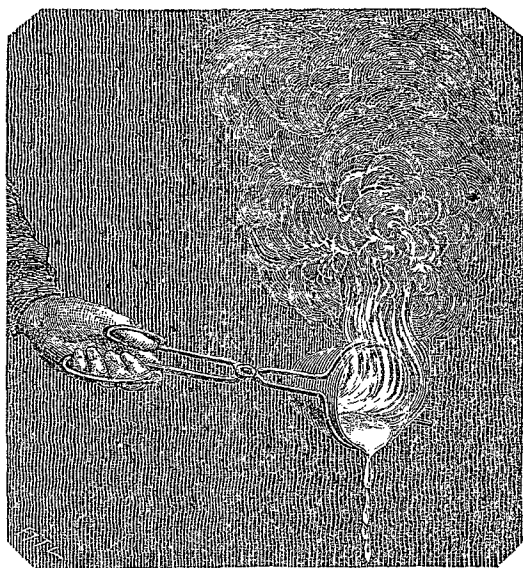
Fig. 1. — Combustion du zinc dans un creuset.
