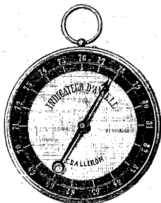
FIG. 1. Appareils Ansell pour reconnaître la présence du feu grisou.
