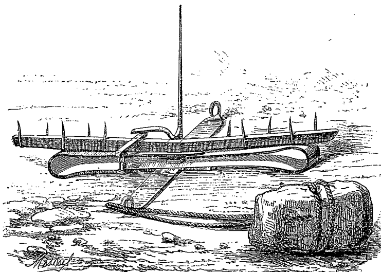
Piège à saumons tendu. — Dessin de Mesnel, d'après une photographie de H. de la Blanchère.
