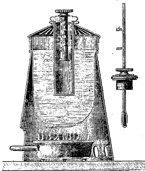
FIG. 2. — Aleuromètre de Boland.
