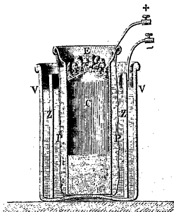
FIG. 1. — Élément d'une pile de Daniell.
