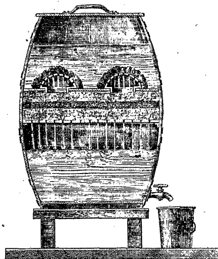
FIG. 2. — Filtre-fontaine à charbon.
