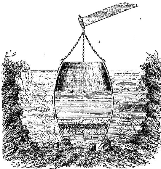
FIG. 3. — Filtre permanent établi dans une mare.
