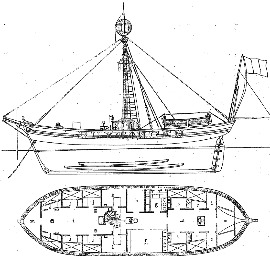
Élévation et plan d'un feu flottant jaugeant 150 tonneaux.
