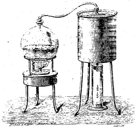
Appareil Salleron pour déterminer la quantité d'alcool contenue dans le vin.
