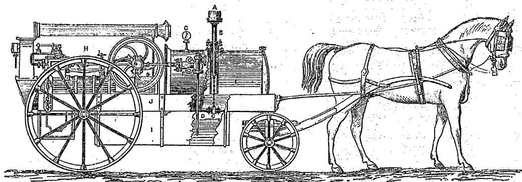
Appareil locomobile pour l'injection des bois. — Dessin de Kautz.
