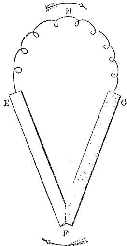
FIG. 1. — Barreaux d'antimoine et de bismuth soudés.
