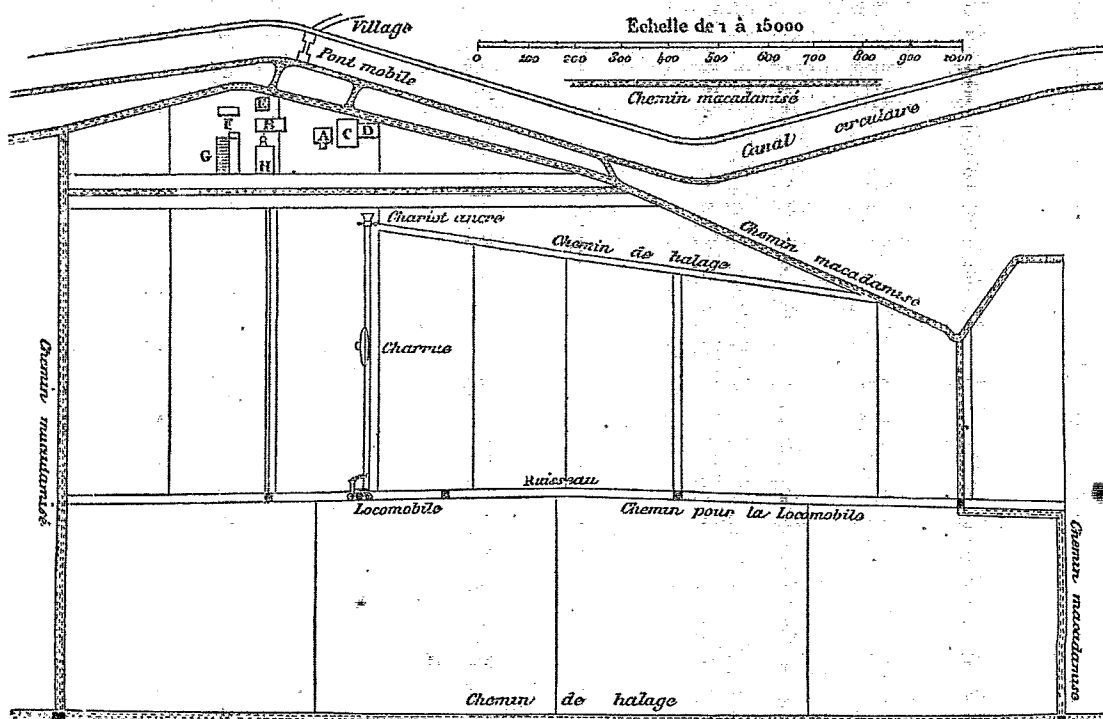
Plan de la ferme des Bains, au lac de Harlem (Hollande).
