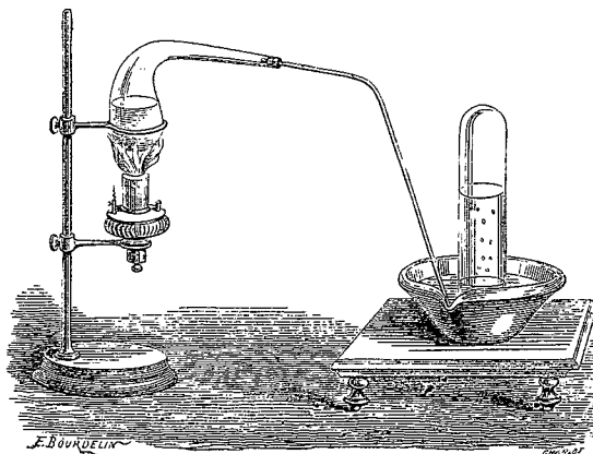
FIG. 1. — Préparation du cyanogène.
