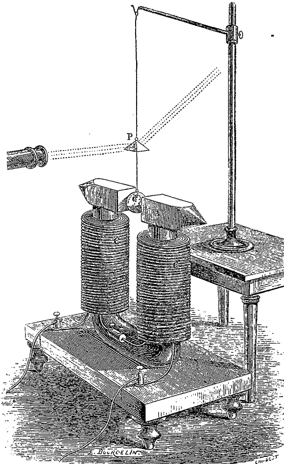
Expérience de Tyndall.
