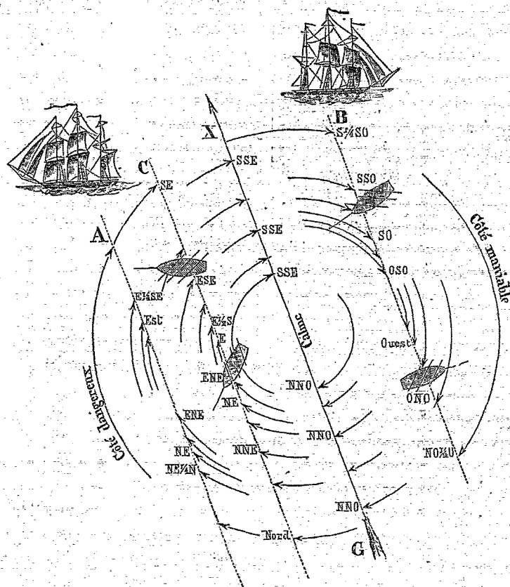
Fig. 2. — Tourbillon de l'hémisphère sud.
