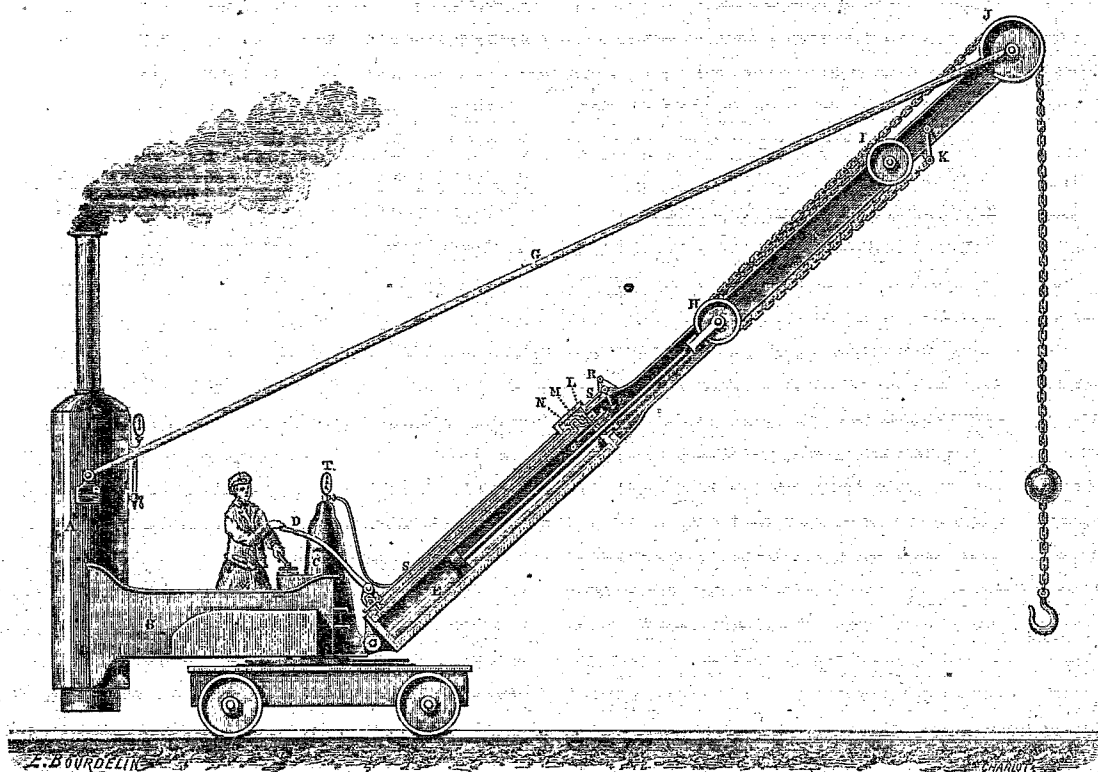
Grue locomobile à vapeur, à action directe; système J. Chrétien. — Dessin de Bourdelin.
