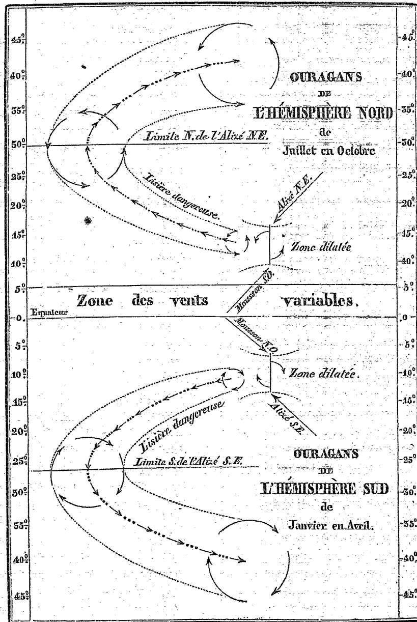
Parcours moyen des ouragans. — D'après M. Keller.
