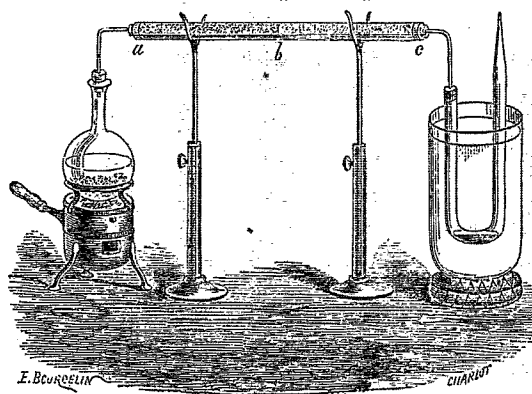
FIG. 3. — Préparation de l'acide cyanhydrique.
