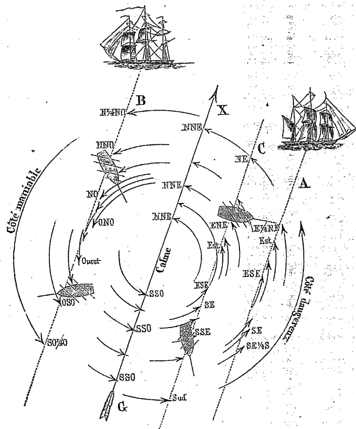
FIG. 1. — Tourbillon de l'hémisphère nord.
