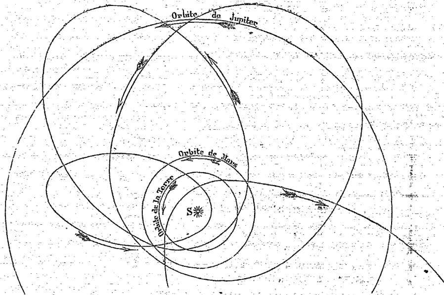
Orbites entrelacées de six comètes voisines.
