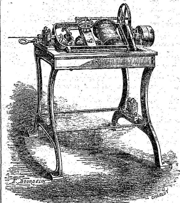
Machine à filer inventée et construite par M. Pragneau, de Bordeaux.
