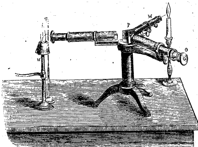
FIG. 4. — Le Spectroscope.
