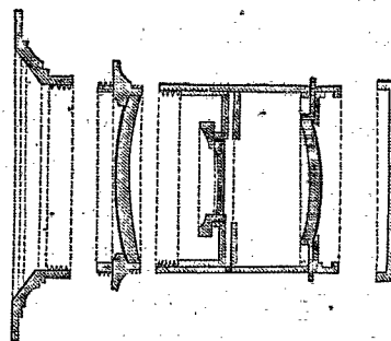
Triplet Ross et Dallmeyer.
