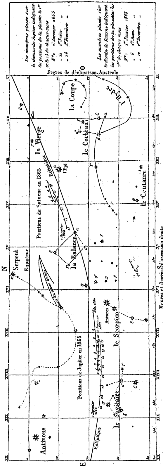
Positions de Jupiter et de Saturne en 1865.
