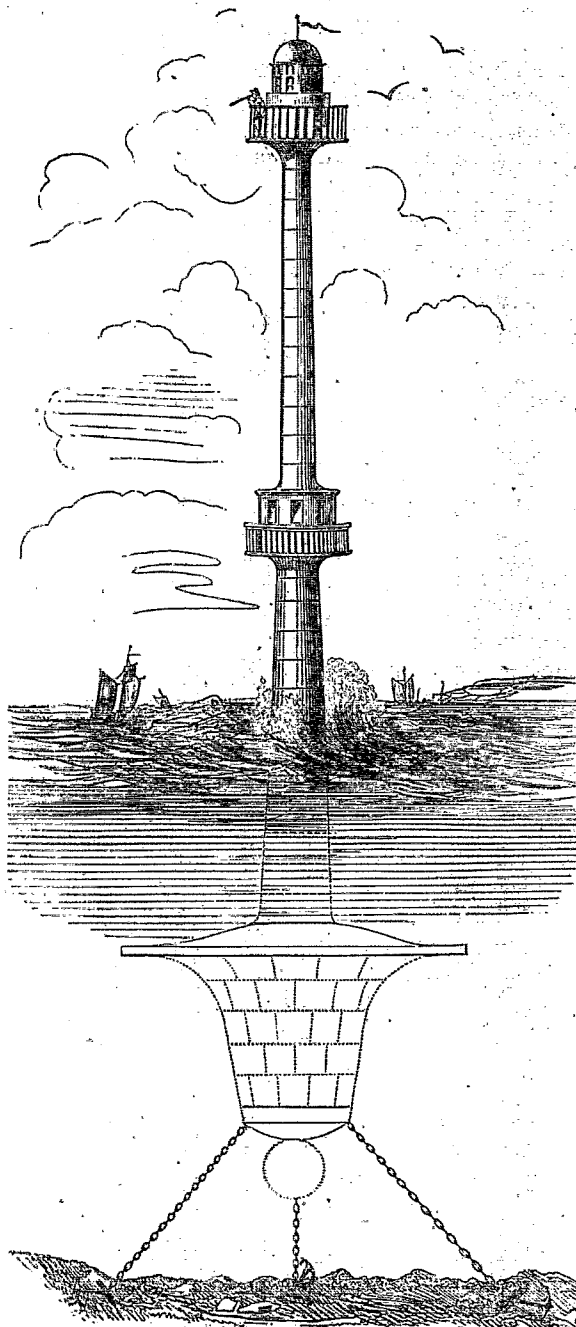
Projet de phare flottant.
