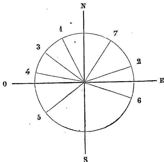
Rose de la direction des principales chaînes de montagnes de France.
