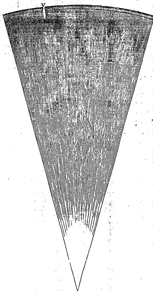
Coupe montrant à peu près les volumes relatifs de l'écorce solide et de la masse liquide du globe. — V, volcan.
