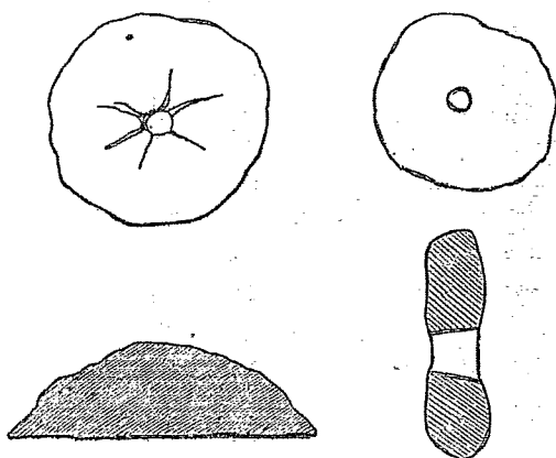
Formes de deux grêlons recueillis par M. Lowe à Nottingham.
