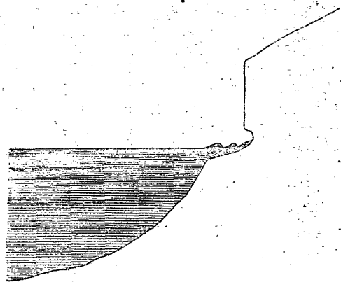
Profil d'une falaise de la Méditerranée.
