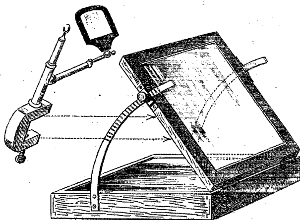
FIG. 18. — Pupitre transparent et loupe pour la retouche des négatifs.
