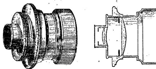
FIG. 22. — Objectif orthoscopique.
