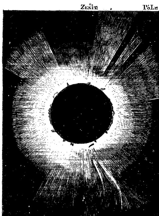
Observations faites à la station du Desierto de las Palmas . Dessin de Gagniet.
