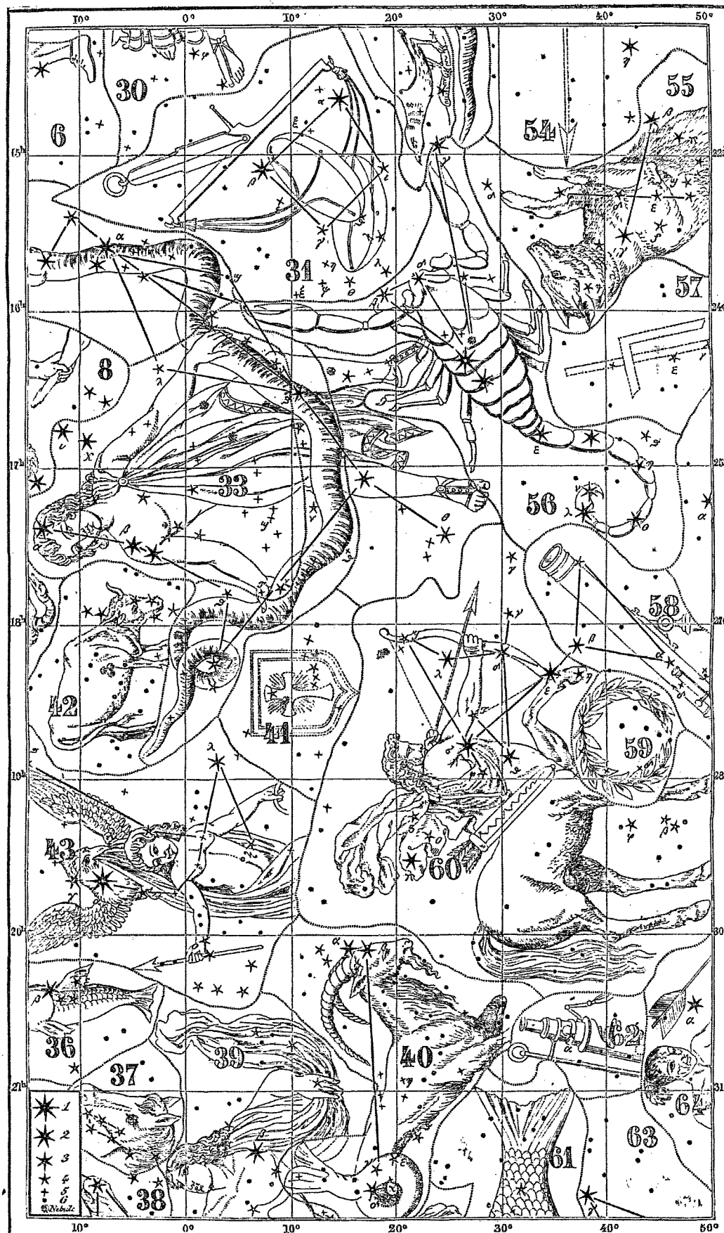
Cartes célestes. — Planche VII.
