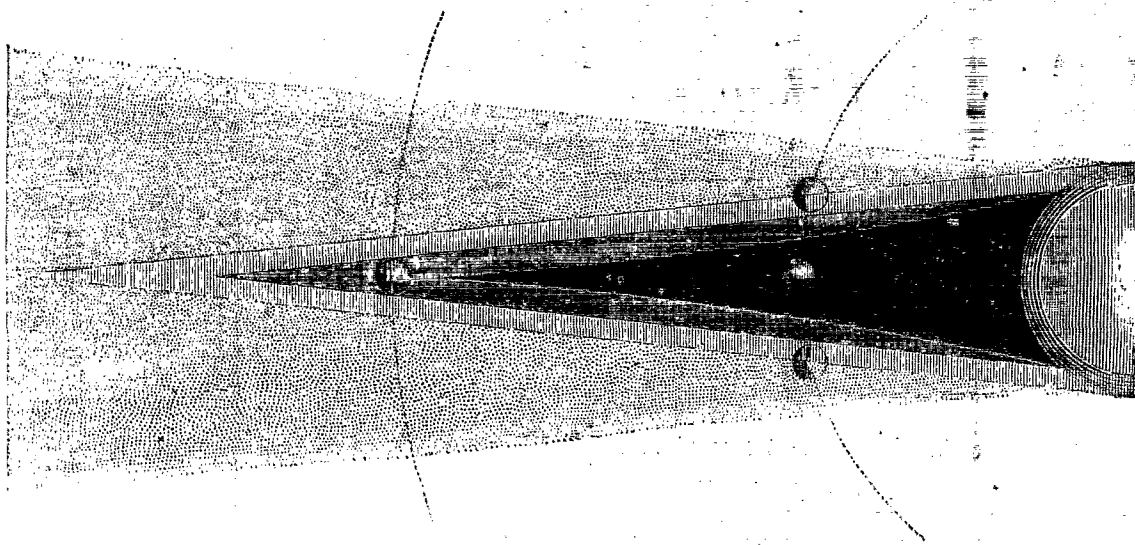
Théorie des éclipses de Lune.
