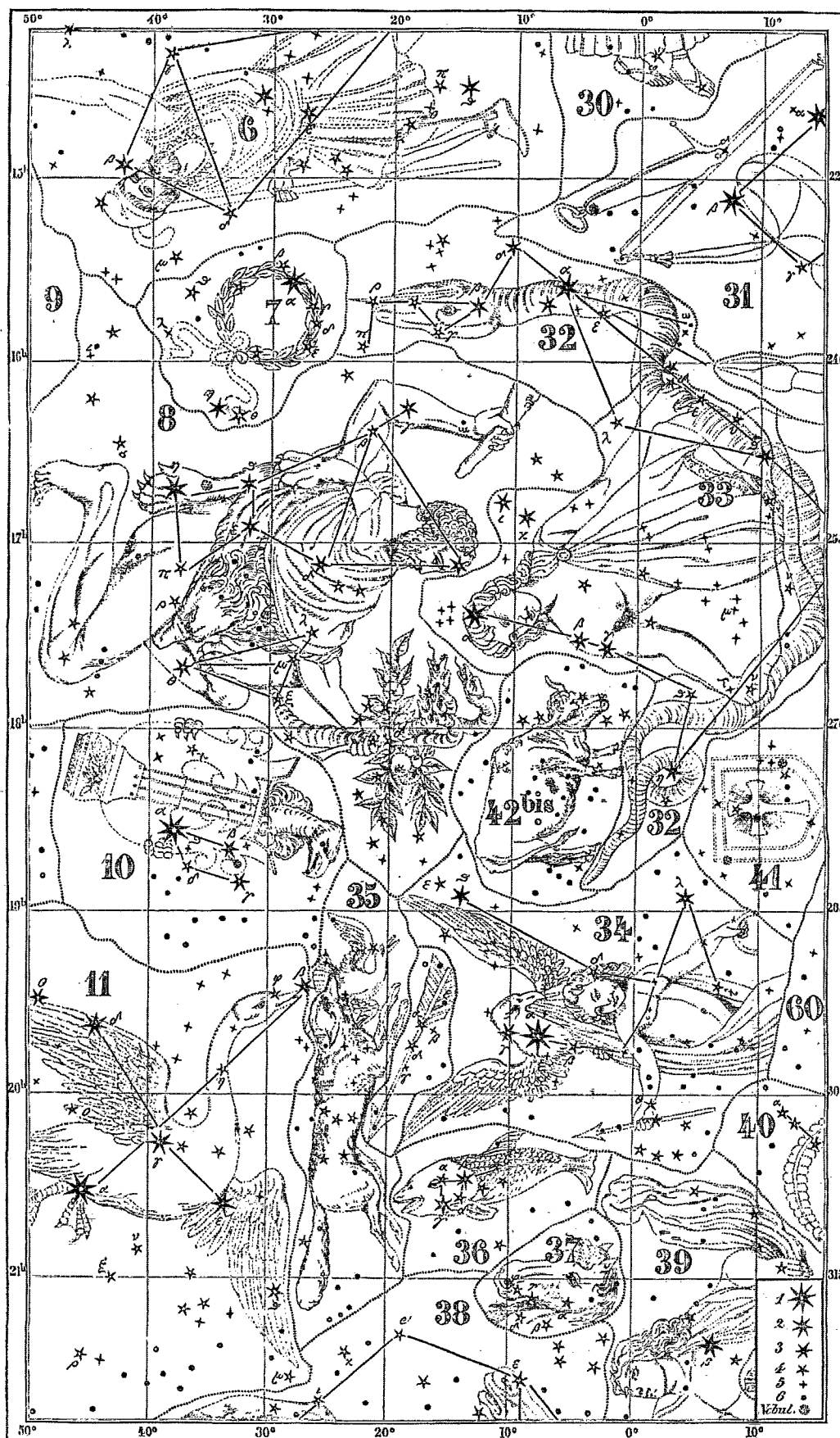
Cartes célestes. — Planche VI.
