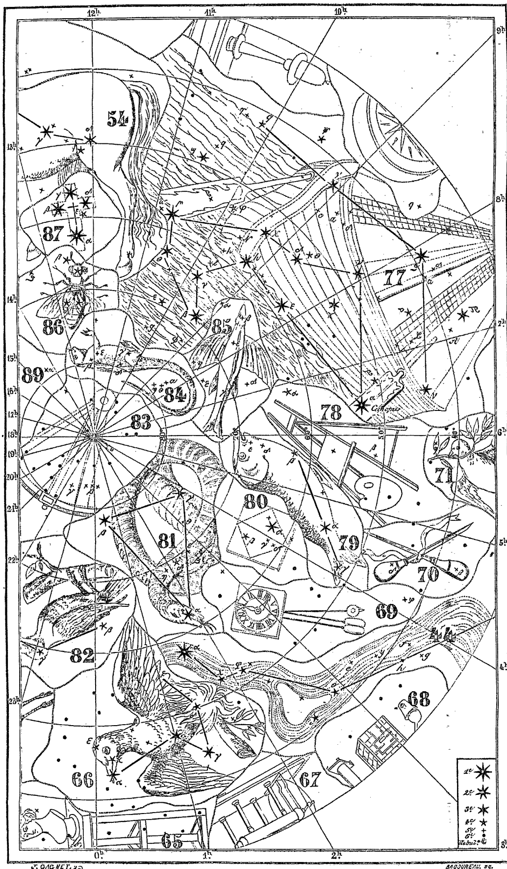
Cartes célestes. — Planche XII.
