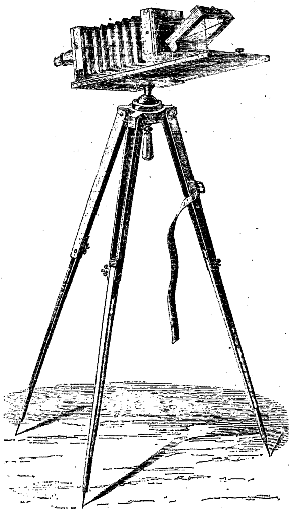
FIG. 19. — Appareil photographique de campagne.
