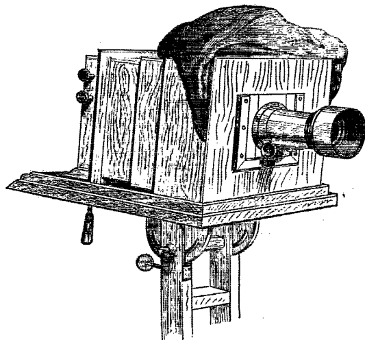
FIG. 4. — Chambre noire vue par devant.
