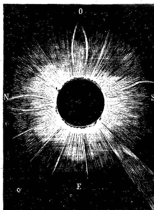
Observations faites à Tarazona. — Dessin de Gagniet.
