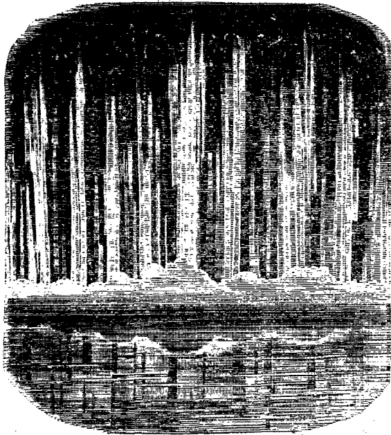
Aurore australe.
