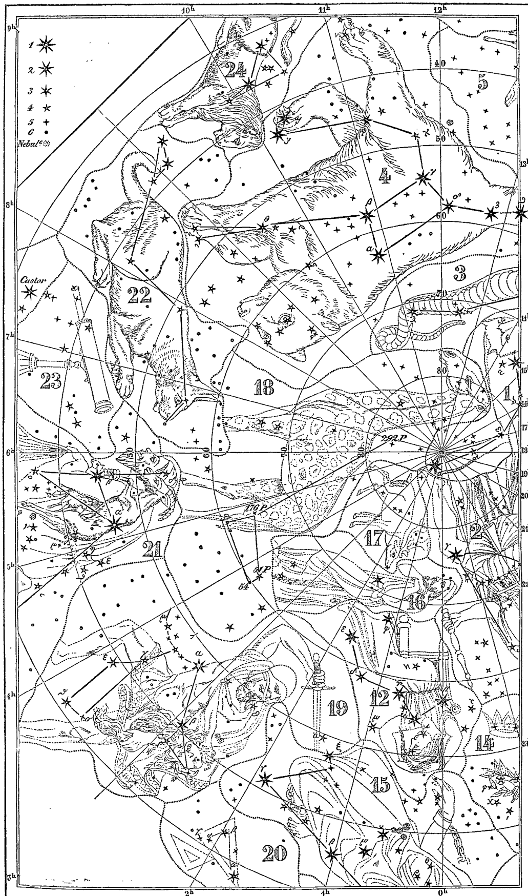
Cartes célestes. — Planche II.
