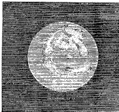
Aspect de Mars pendant l'opposition.
