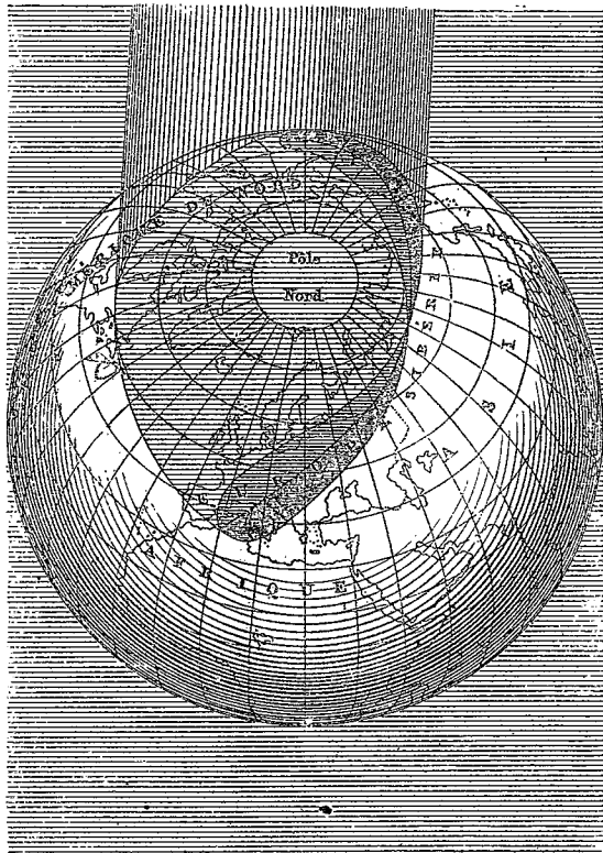
La Terre sous l'éclipse de Soleil du 17 mai 1863.
