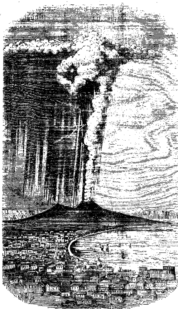
Éruption du Vésuve en 1855.
