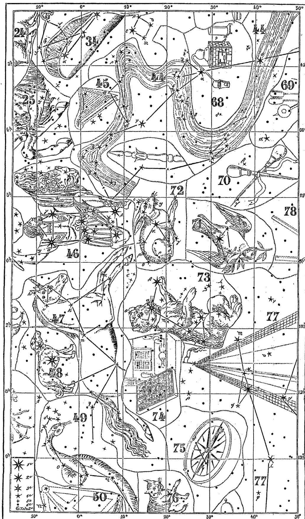
Cartes célestes. — Planche IX.
