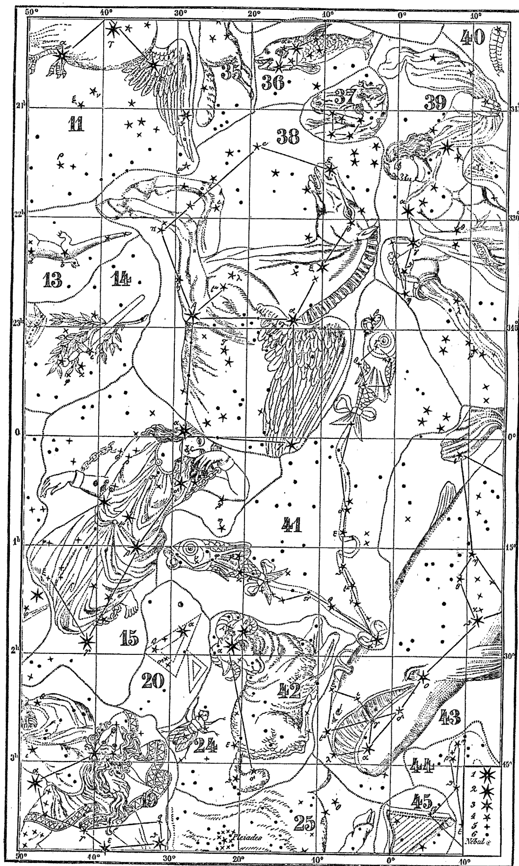
• Cartes célestes. — Planche III.
