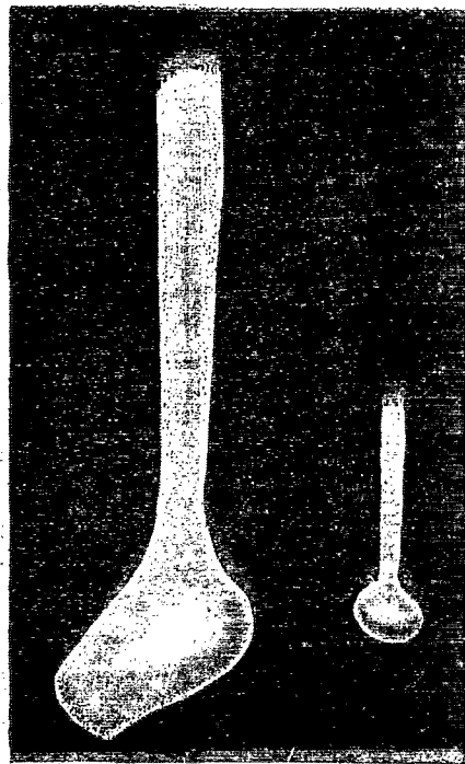
Comètes dessinées par M. Chacornac.
