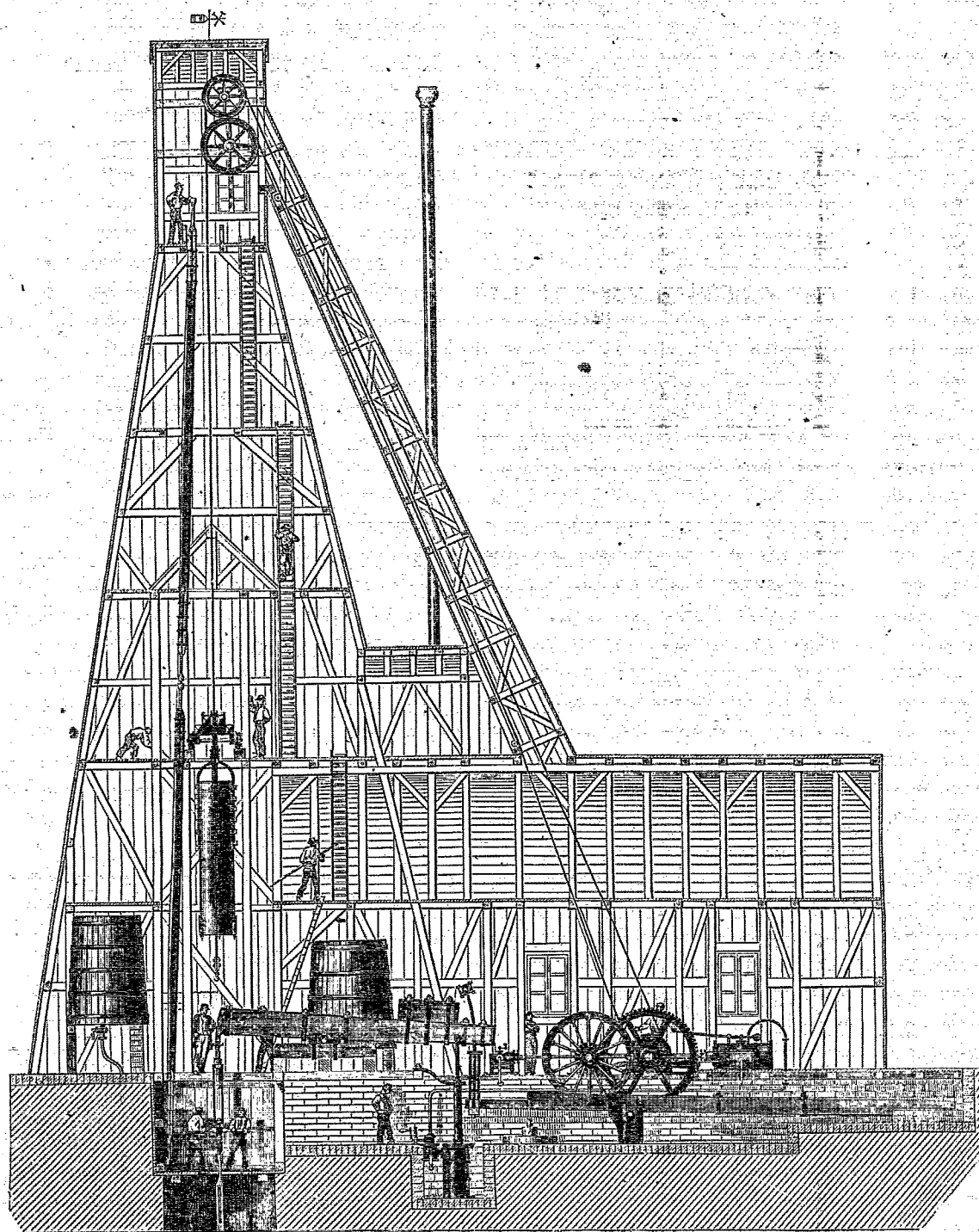
Fig. 7. — Puits artésien de Passy : coupe en longueur du bâtiment pendant le travail du forage.
