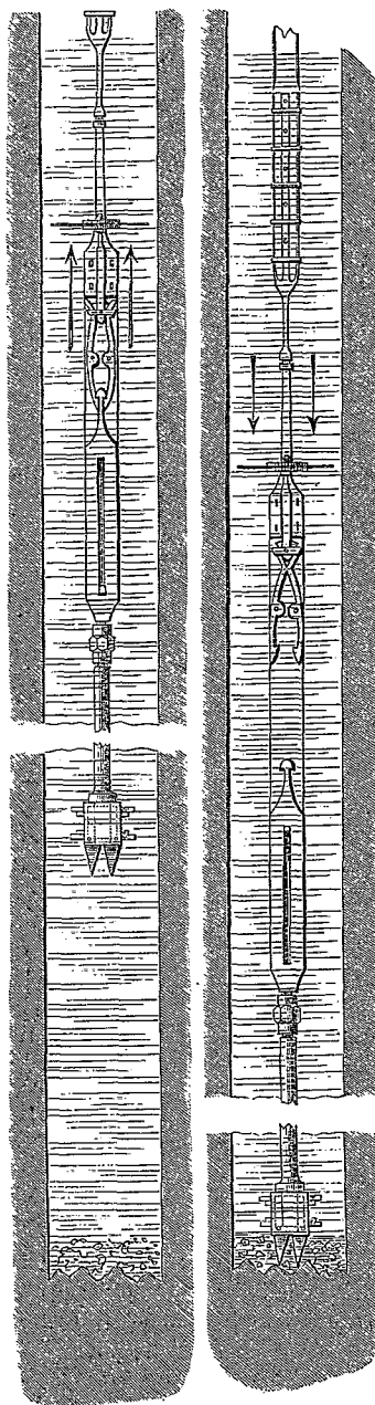
FIG. 4 et 5. — Manœuvre du déclie.
