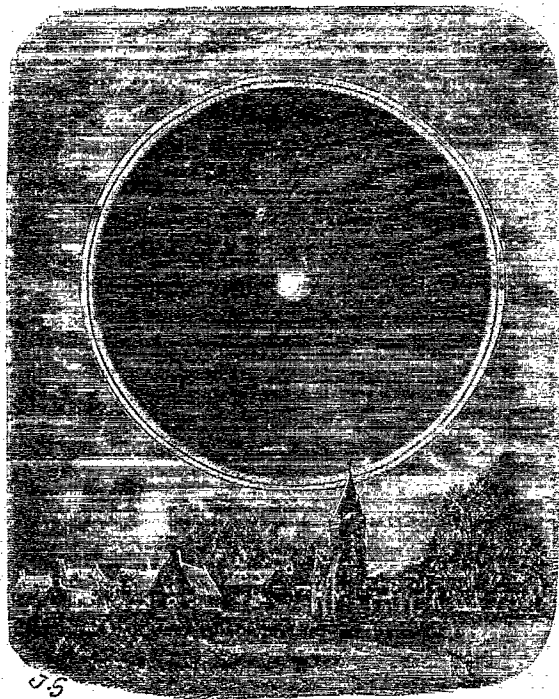
Halo lunaire.
