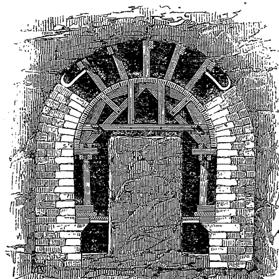
FIG. 8. — Méthode par section divisée. — Construction de la voûte.
