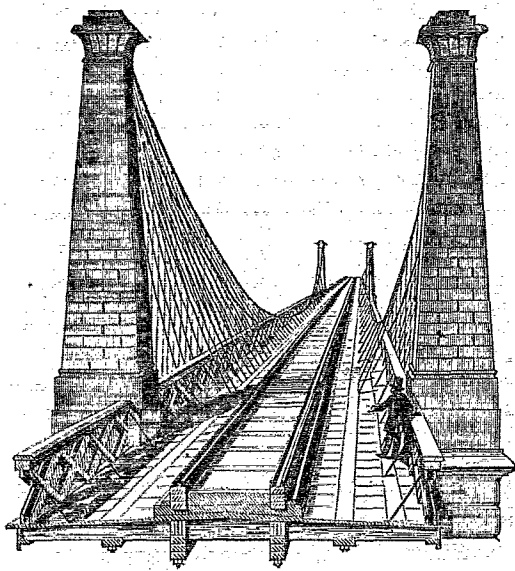
FIG. 2. — Pont du Niagara. — Coupe en travers et perspective du tablier supérieur.
