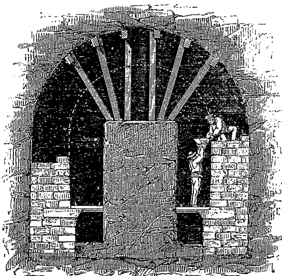
FIG. 7. — Méthode par section divisée. — Achèvement du ciel de l'excavation.
