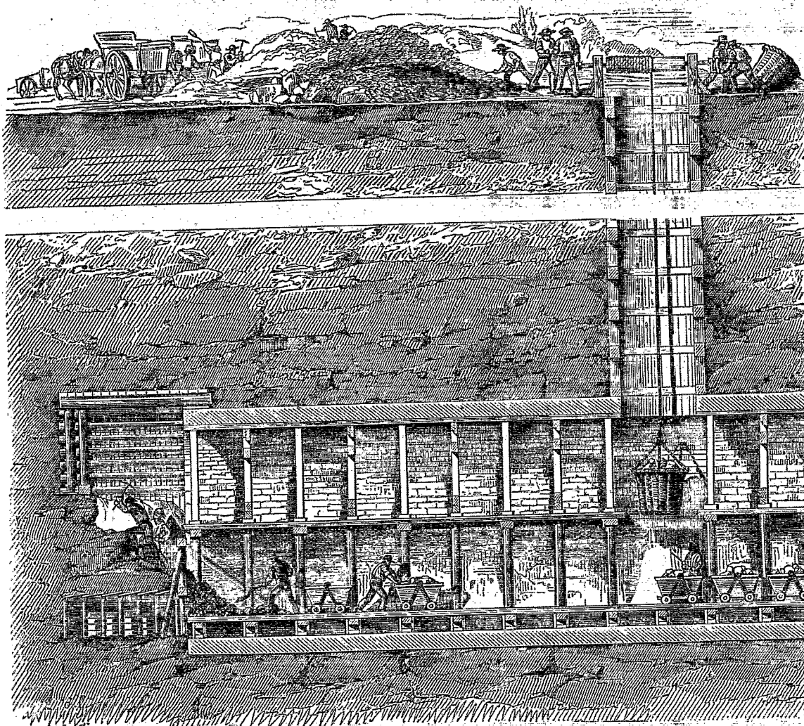
FIG. 2. — Coupe d'un puits d'extraction et de sa galerie.
