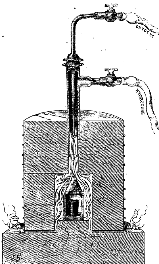
FIG. 7. — Chalumeau à gaz hydrogène et oxygène.
