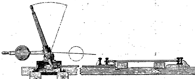
FIG. 5. Aiguilles simples; coupe verticale, pour faire comprendre la manœuvre.
