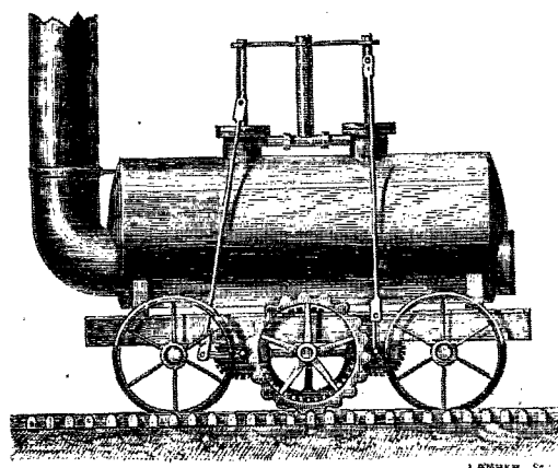
FIG. 2. — Locomotive à roues dentées, de Blenkinsop (1811).
