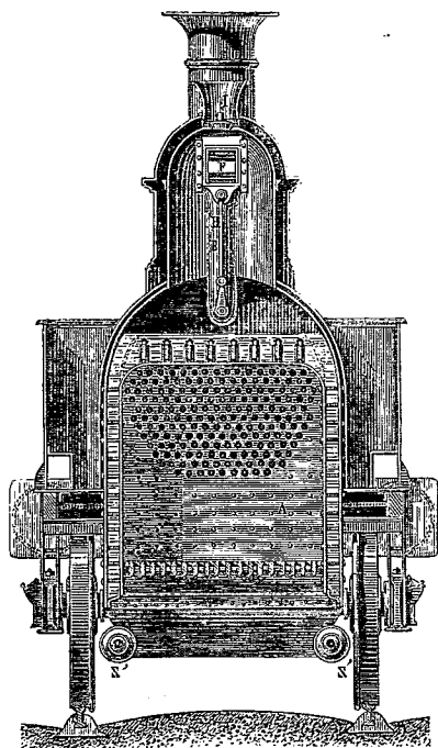
FIG. 2. Coupe transversale par la boîte à feu.
