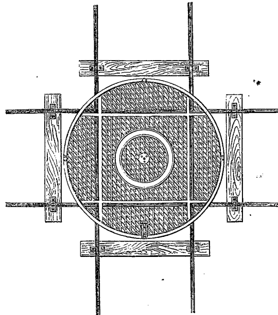
FIG. 9. Plaque tournante pour deux voies perpendiculaires l'une à l'autre.
