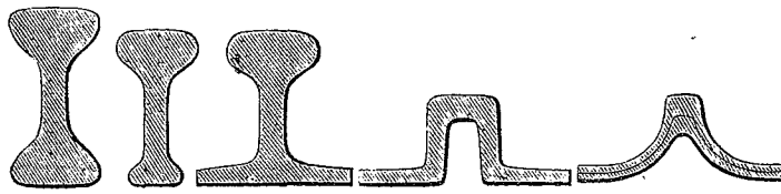
FIG. 1. Diverses formes de rails : --- Rail à double champignon, à simple champignon, à patin (rail Vignolles) ; rail Brunel ; rail Barlow.
