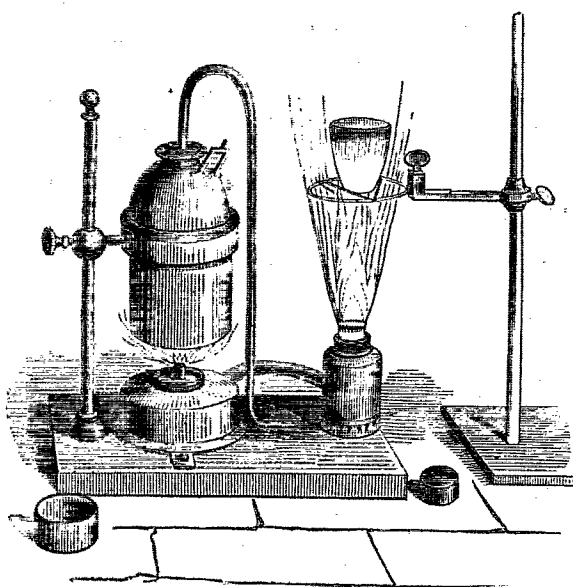
FIG. 5. — Éolipyle.
