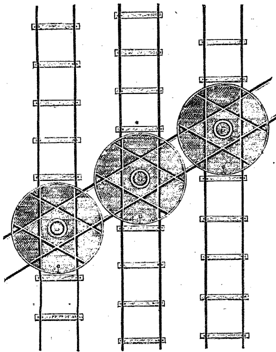
FIG. 12. Plaque tournantes pour trois voies parallèles et une oblique.
