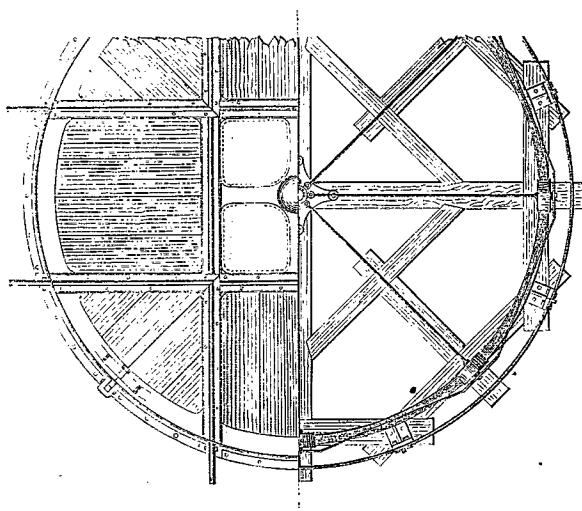
FIG. 7. Plaque tournante en fonte; plan horizontal.
