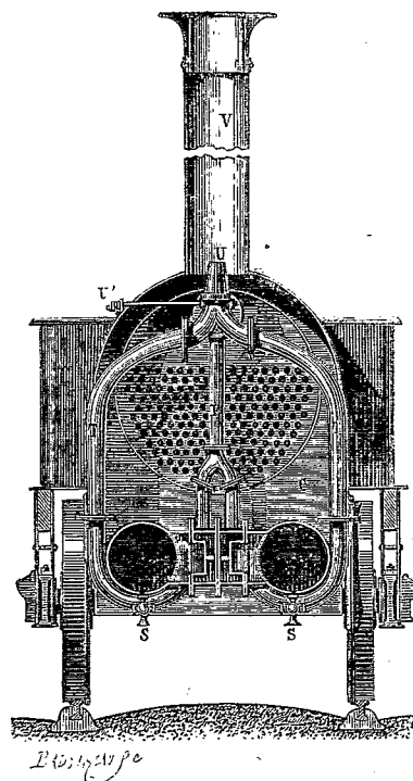
FIG. 3. Coupe transversale par la boîte à fumée.
