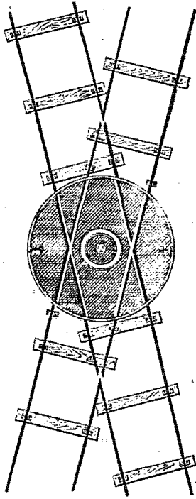
FIG. 10. Plaque tournante pour deux voies obliques.
