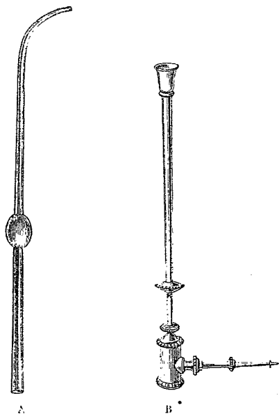
FIG. 1. — A, chalumeau des ateliers; B, chalumeau des laboratoires.
