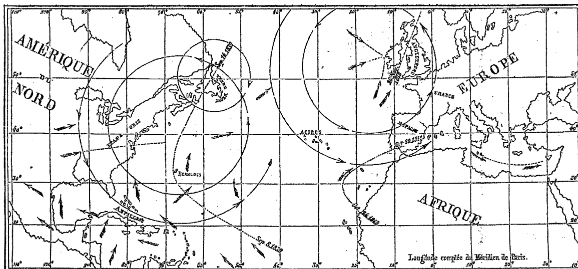
FIG. 2. Carte de la marche de plusieurs Cyclones.
