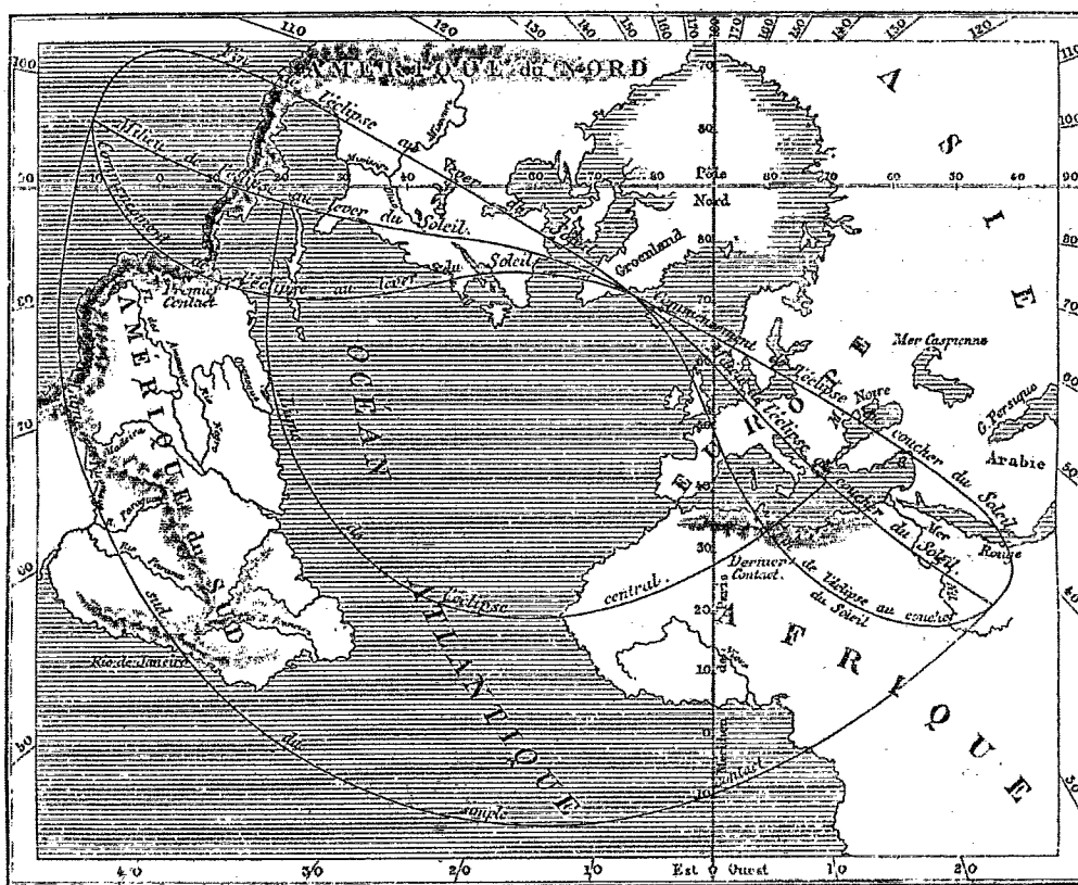
Carte de l'éclipse de soleil du 31 décembre 1861.
