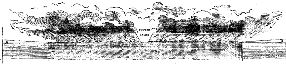
FIG. 1. Coupe supposée d'un Cyclone.
