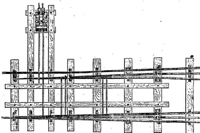
FIG. 6. Aiguilles doubles pour croisement triple.
