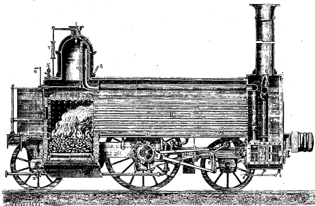
FIG. 1. Coupe longitudinale d'une locomotive.
