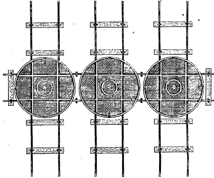
FIG. 11. Plaque tournantes pour trois voies parallèles et une perpendiculaire.
