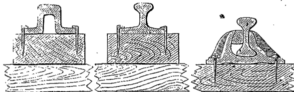
FIG. 2. Divers modes d'assemblage de voies.
