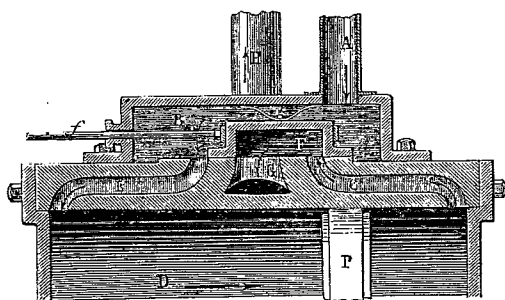
FIG. 4. Tiroir; première position.
