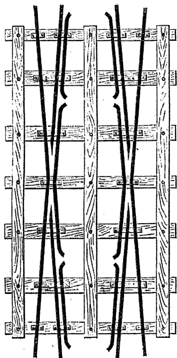
FIG. 3. Croisement de voie simple.
