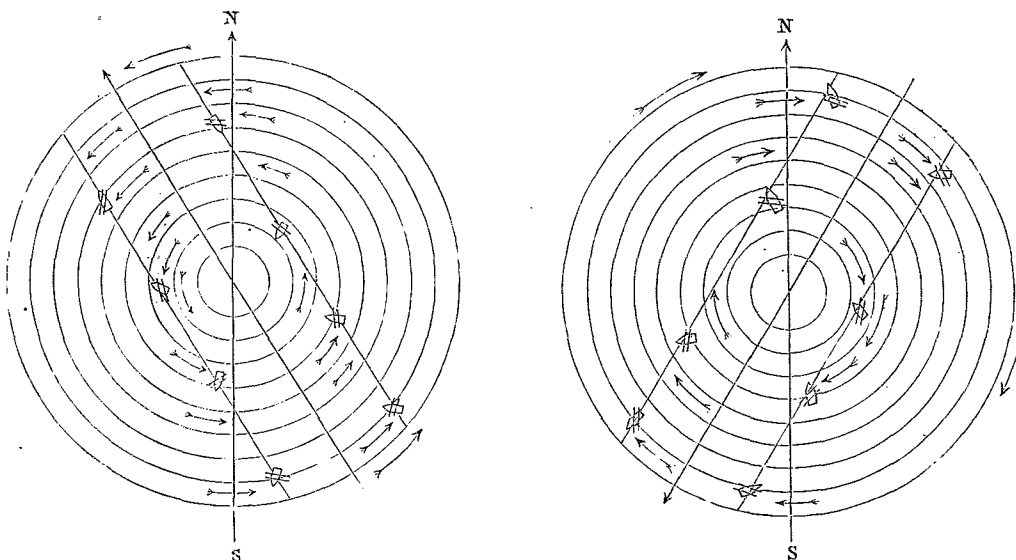
FIG. 3. Navires fuyant le centre du Cyclone.
