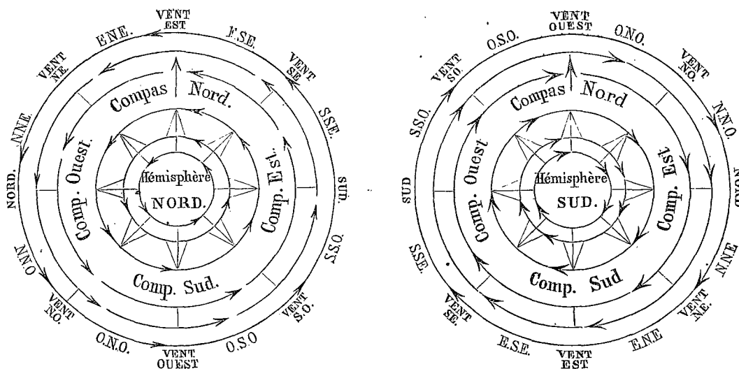
FIG. 4. Roses des tempêtes.
