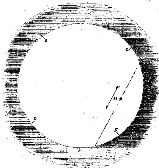
Marche apparente de Mercure sur le disque solaire le 2 novembre 1861.
