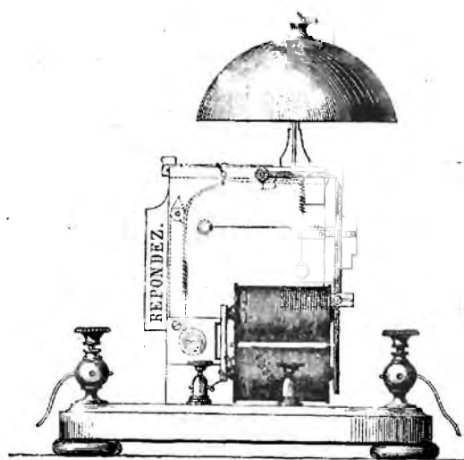
FIG. 9. — Sonnerie Bréguet.
