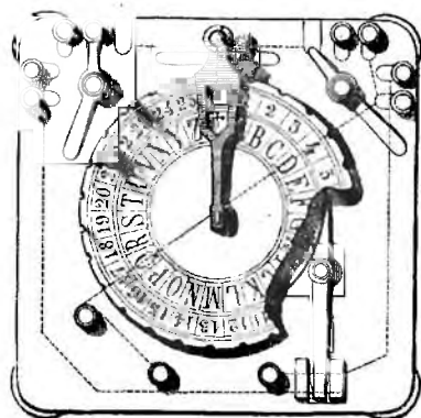
FIG. 6. — Manipulateur Bréguet.
