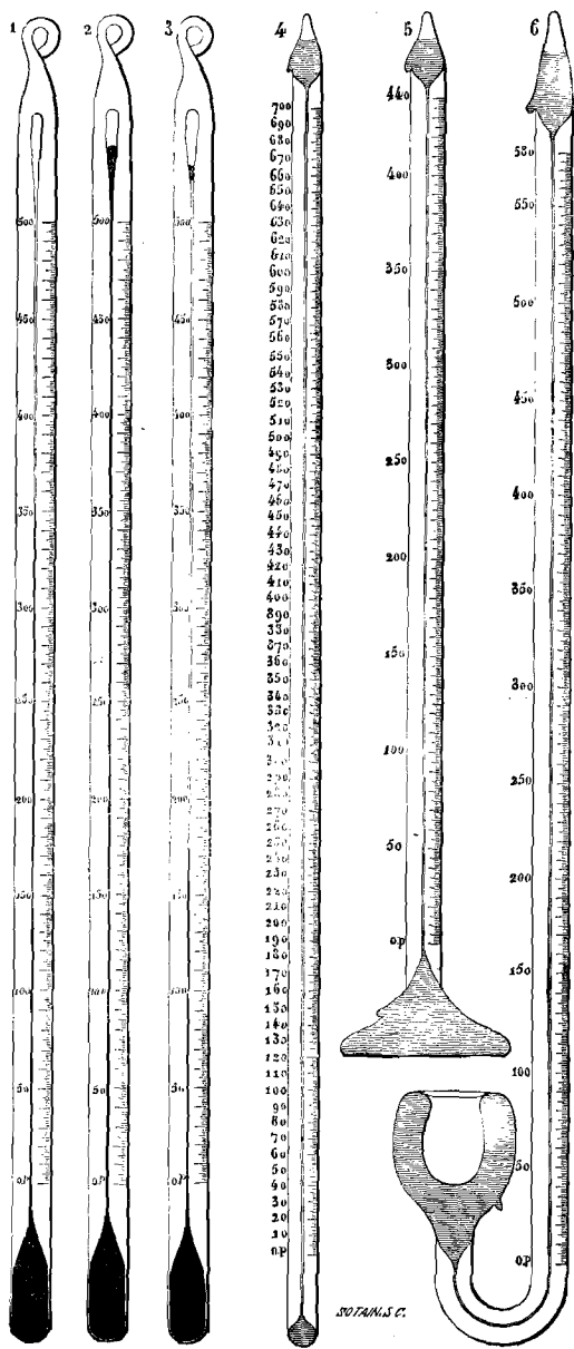
Thermomètres métastatiques.
