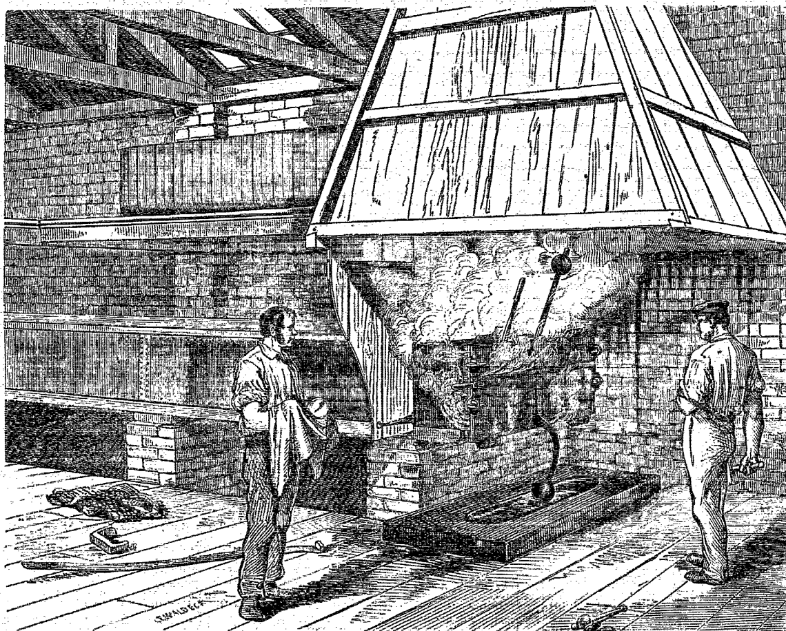
FIG. 6. Réservoir à vapeur pour la préparation des bois destinés à la courbure.
