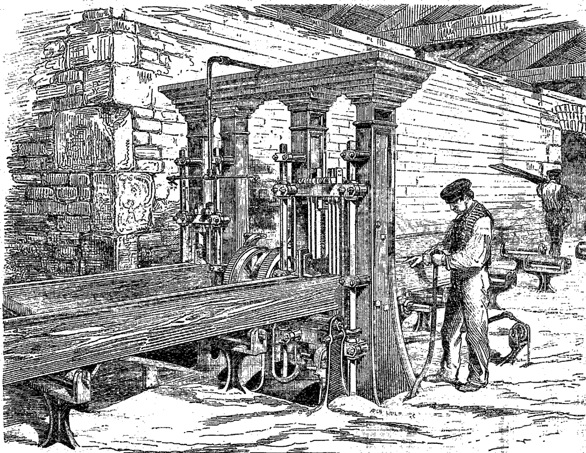
FIG. 1. Scie verticale à plusieurs lames.
