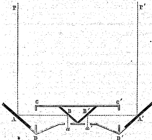
FIG. 1. Plan du téléstéréoscope.
