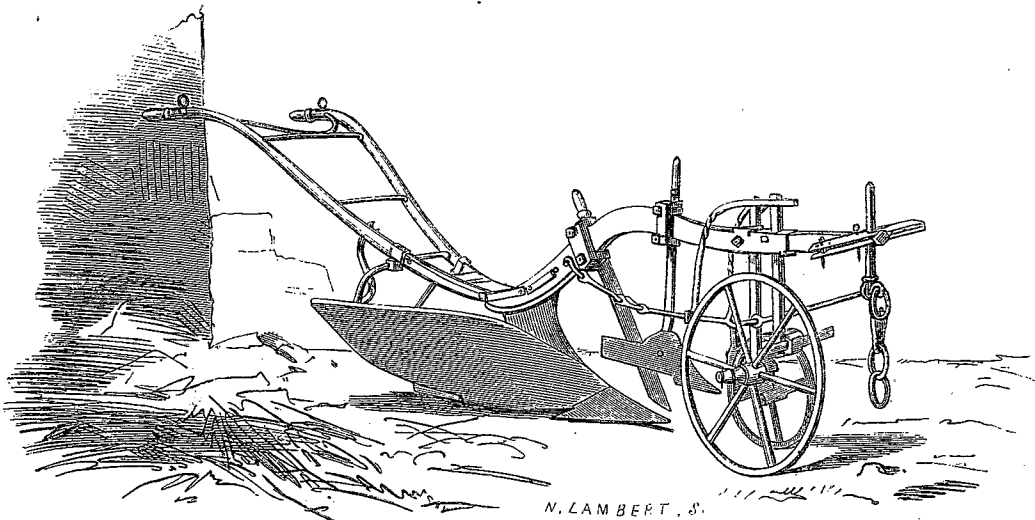
La Charrue Howard. — Dessin de Lambert.
