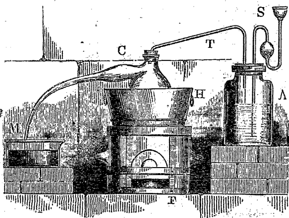
FIG. 3. Préparation du phosphore rouge.
