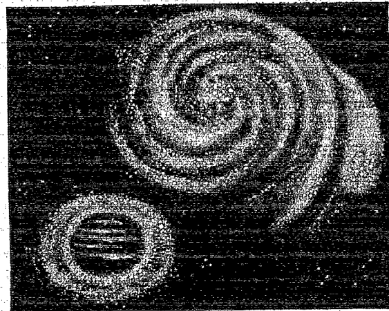
Nébuleuse annulaire et Nébuleuse spirale.
