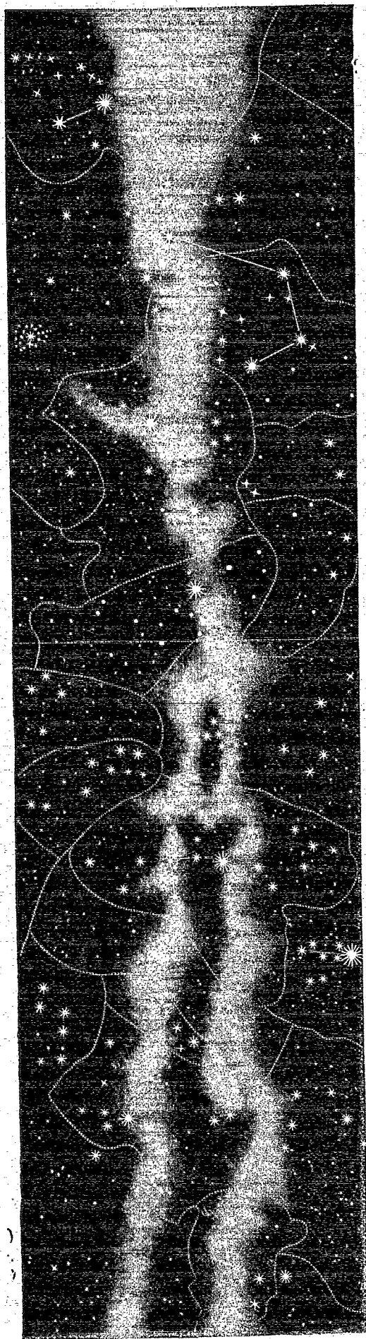
La Voie lactée. — Partie Nord.
