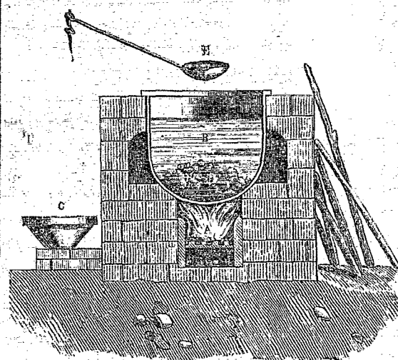
FIG. 1. — A, feu du fourneau. — B, mine de soufre en fusion; les matières terreuses se déposent au fond de la chaudière. — C, vase dans lequel le soufre épuré se refroidit et se solidifie. — E, cuiller pour puiser le soufre dans la chaudière et le verser dans le vase C.
