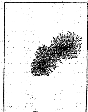
Taches observées sur le disque du soleil dans le courant de 1826, par M. Capocci.
