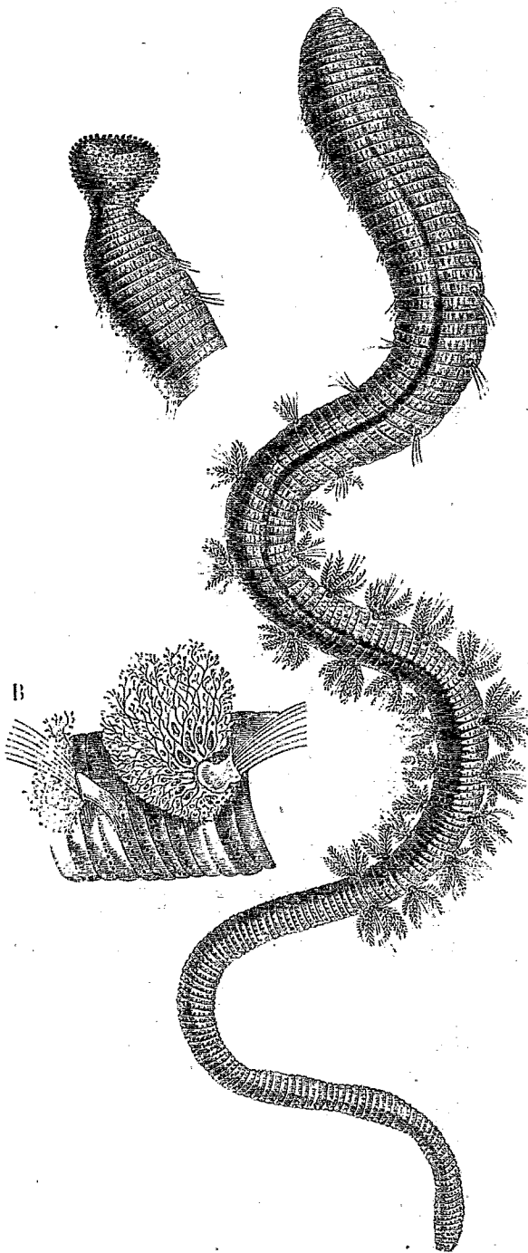
L'Arénicole des pêcheurs. — A, extrémité antérieure du corps, montrant la trompe; B, un des anneaux de la partie moyenne du corps, grossi, vu de côté, pour montrer les branchies et les rames des pattes.
