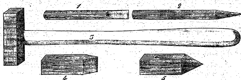
Instruments du géologue. — Ciseau, pointe, marteaux.
