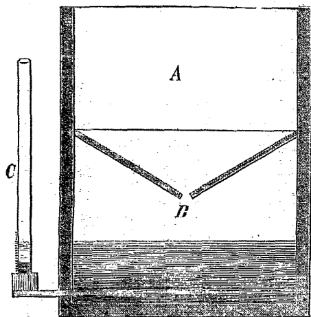
Pluviomètre ou Udomètre.
