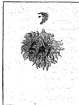
Taches observées sur le disque du soleil dans le courant de 1826, par M. Capocci.
