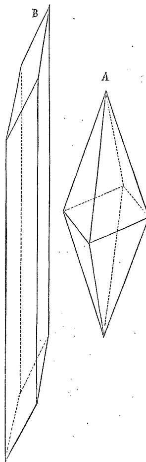
FIG. 4. Cristaux de soufre.
