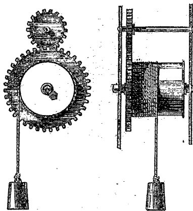
FIG. 1. Poids moteur des horloges, vu de face et de profil.
