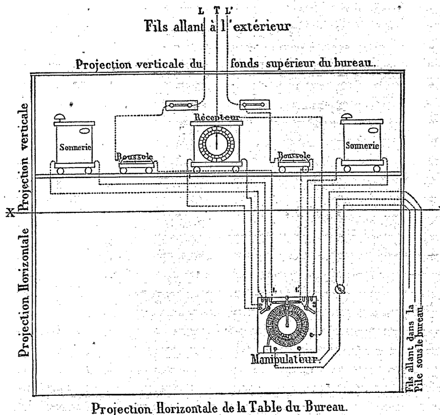
Appareil télégraphique des chemins de fer.
