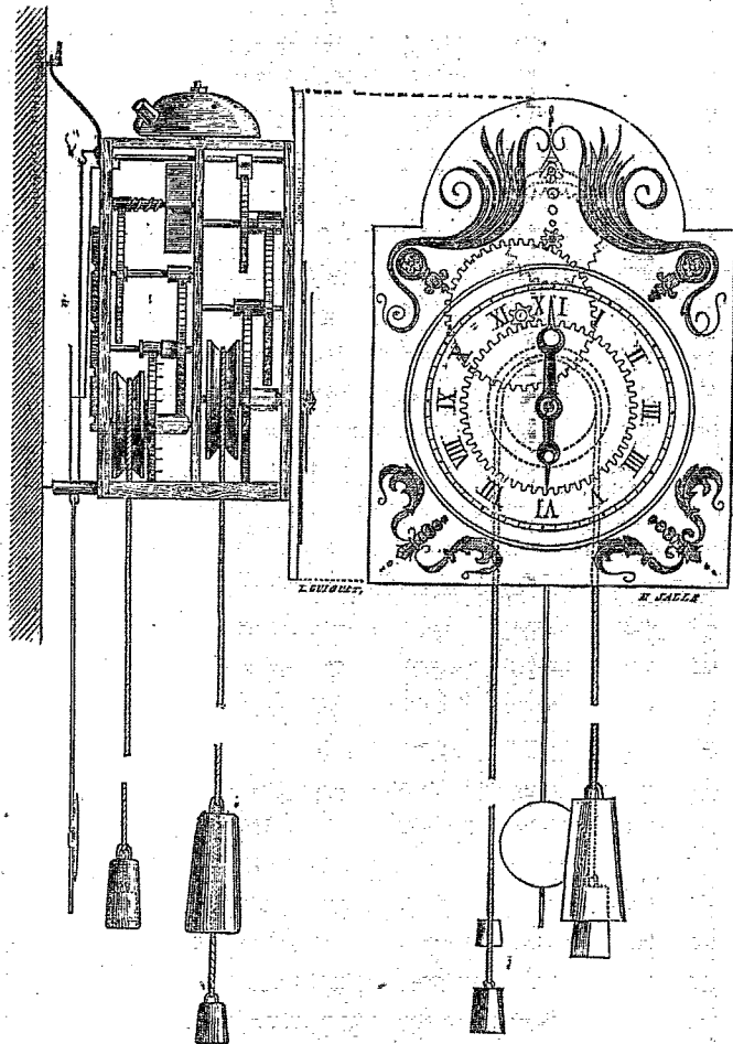
FIG. 2. Horloge à poids, vue de profil et de face.
