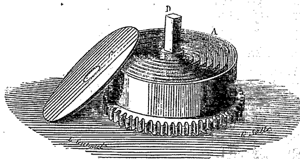
FIG. 5. Ressort moteur des horloges enfermé dans le barillet A muni d'une roue dentée. — B, axe à tête carrée D pour remonter le ressort détendu. — C, couvercle du barillet, découvert dans la figure pour laisser voir le ressort.
