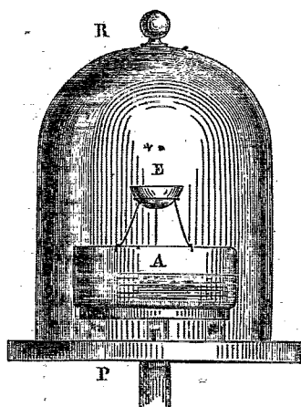
R, récipient où l'on a fait le vide. — A, vase contenant de l'acide sulfurique. — E, capsule légère, en cuivre, où l'on met de l'eau qui se gèle en quelques instants avec une bonne machine pneumatique.
