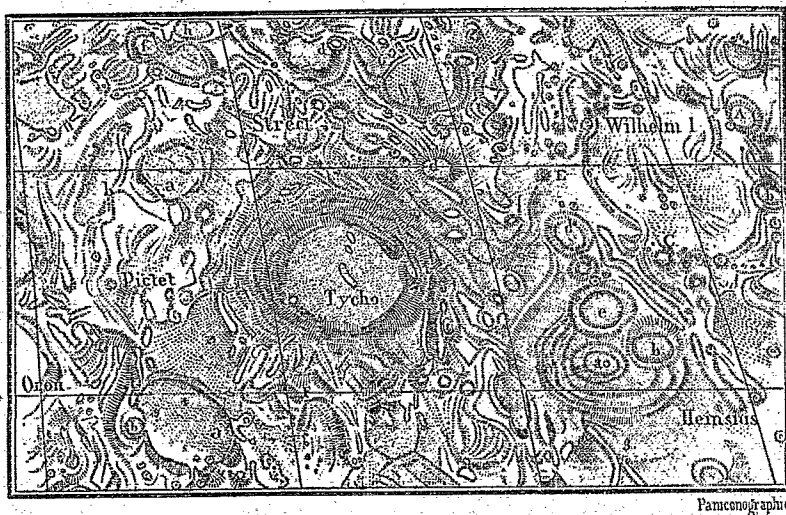
Le canton de Tycho, dans la Lune. — Fac-simile d'un fragment de la Carte de la Lune de MM. Beer et Madler.
