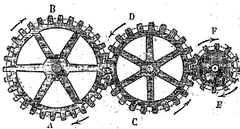
FIG. 3. Mouvement des cercles contigus, d'après Aristote.
