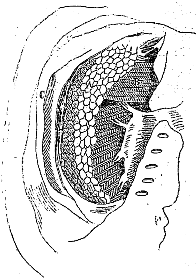
Organe électrique de la Torpille. — A, section en travers, un peu oblique; B, direction des prismes où siège l'électricité; C, les téguments écartés pour laisser voir l'organe; — D, section perpendiculaire des prismes.
