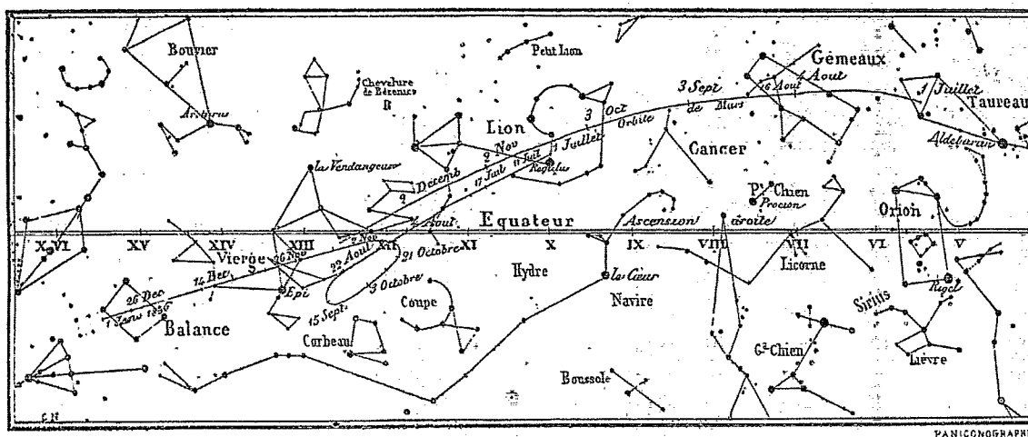
La courbe supérieure indique la marche de Mars; — la courbe inférieure, celle de Vénus.
