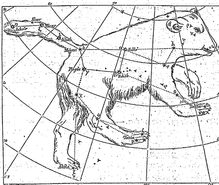
Constellation de la Grande-Ourse (*).
