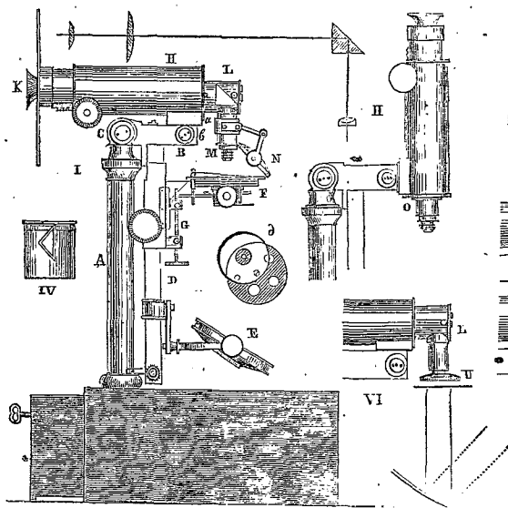
Fig. 9. Microscope de Charles Chevalier.
