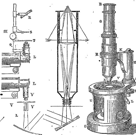
Fig. 10. Microscope de Nachet.
