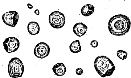
FIG. 13. Tapioka, grossi 400 fois.
