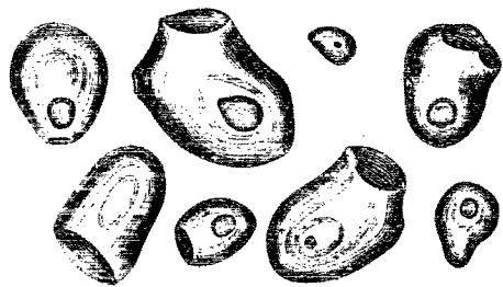
FIG. 15. Sagou, grossi 400 fois.
