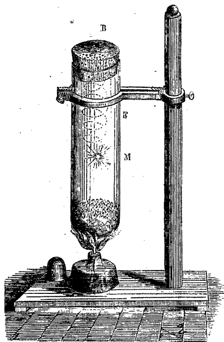
FIG. 2. Support pour placer commodément le tube sur une lampe à alcool ou sur des charbons allumés. Un fil de fer ou d'acier détrempe FM, fixé à un bouchon B qui ne ferme pas exactement le tube, est amorcé en M par un petit morceau d'amadou.
