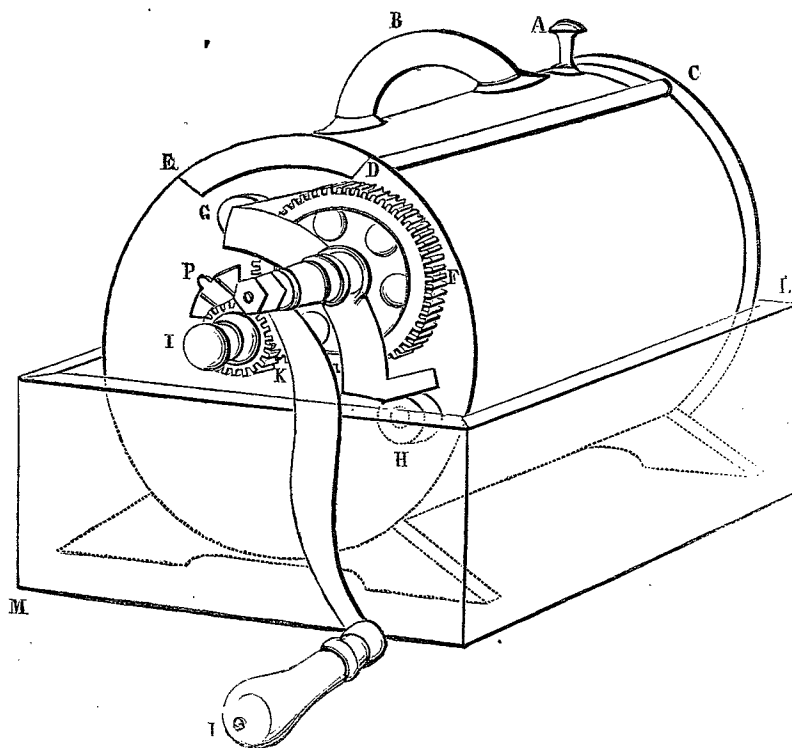
Baratte Valcourt. — FIG. 1.
