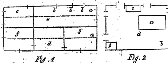
La figure 1 indique la distribution des chambres; la maison n'a qu'un rez-de-chaussée. — La figure 2 est le plan agrandi de la chambre e.
