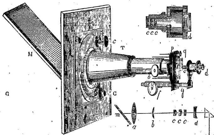
FIG. 12. Microscope solaire.
