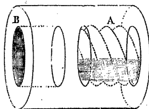
FIG. 13. Mandrin ordinaire.
