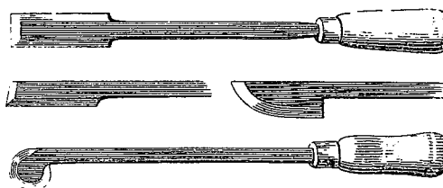
FIG. 9. Fermoirs.
