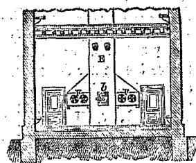
Fig. 4. Coupe en travers du bâtiment; vue prise en regardant la cheminée d'appel.
