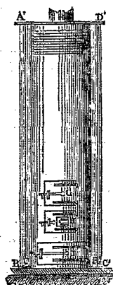
Fig. 5. Élévation du calorifère.
