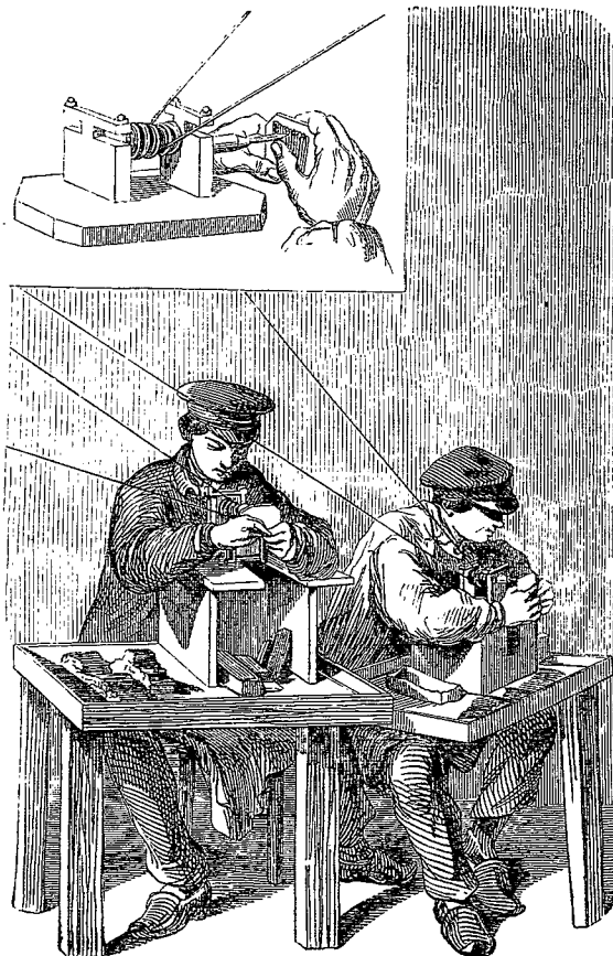
Fig. 4. Drillage ou perfectionnement du trou.
