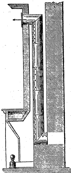
Fig. 1. Mode de ventilation et de chauffage applicable aux habitations les plus pauvres. (Coupe en travers.)
