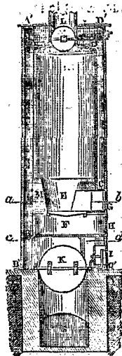
Fig. 6. Coupe verticale du calorifère par ef.
