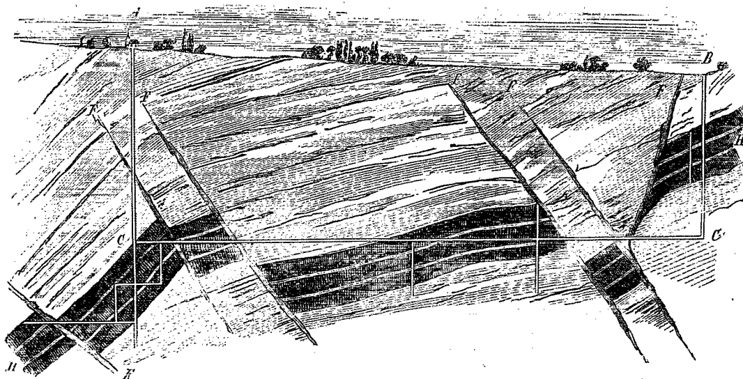
Coupe de la couche de houille de Blanzay dans le sens de son inclinaison, du puits Saint-Pierre au puits de la Maugrand, département de Saône-et-Loire.
