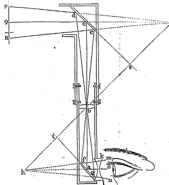
Fig. 4. Le Polémoscope d'Hévélius.
