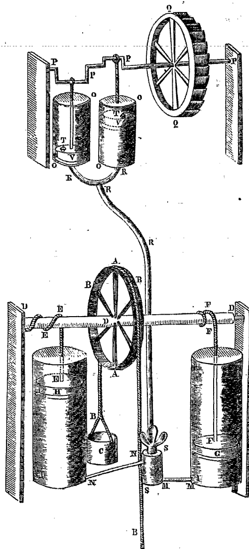
Fig. 3. Première machine atmosphérique sans vapeur, de Papin.
