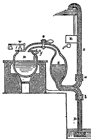
Fig. 4. Machine de Savery. (Coupe verticale.)
