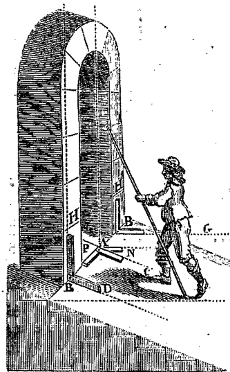
Fig. 3. Berceau cylindrique rampant.
