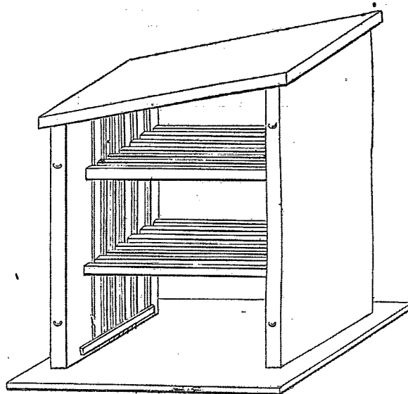
Ruche à cadres ou à châssis verticaux. — Vue intérieure
