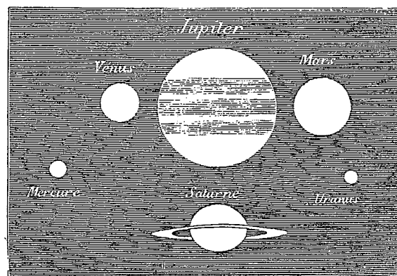
Fig. 3. Apparences relatives des planètes à la fin de l'année.
