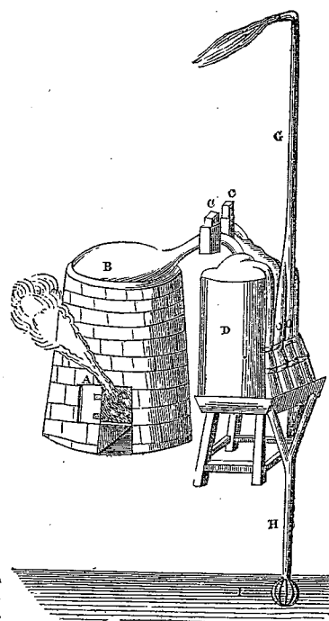
Première machine de Savery, d'après les Transactions philosophiques (1700).
