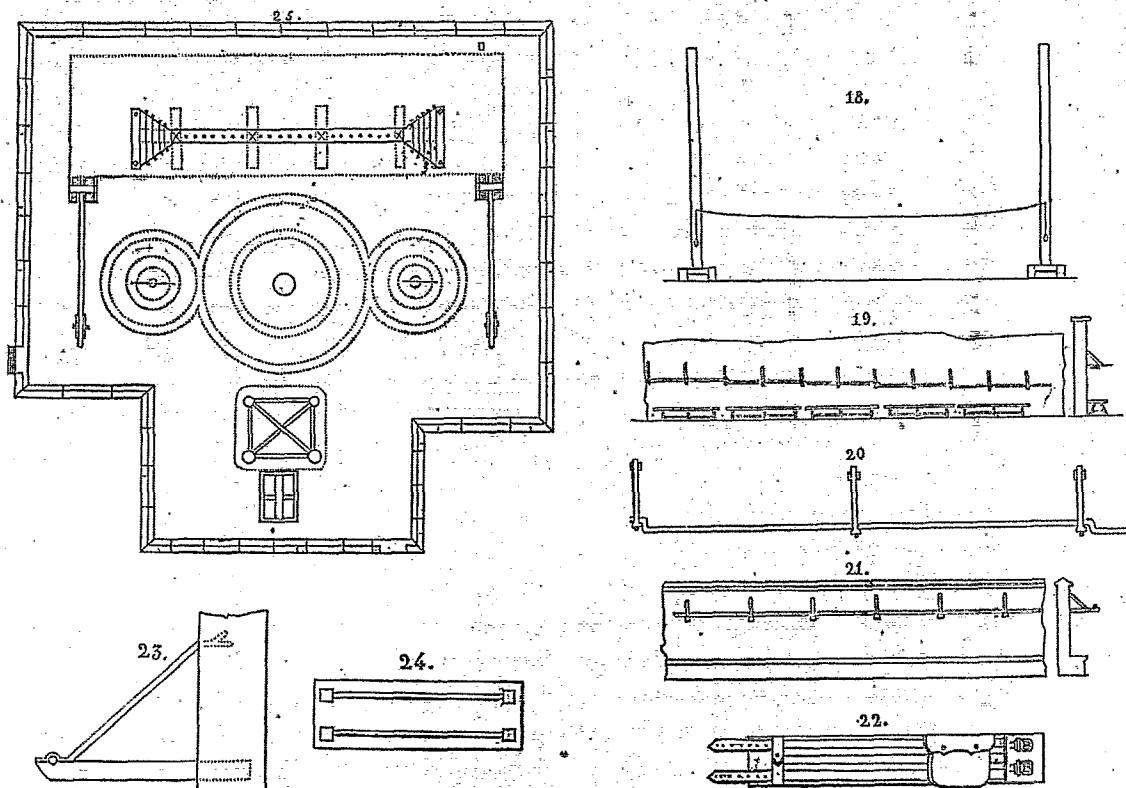
(18. Sautoir. — 19. Barres horizontales pour les différents âges (exercices dits de fermeté). — 20. Développement d'une partie de la fig. 19. — 21. Barres horizontales pour hommes. — 22. Ceinture de gymnastique.)
