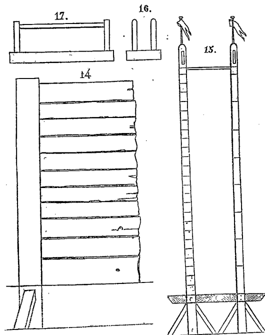
(14. Panneau à franchir, ou mur factice. — 15. Élévation des mâts verticaux (voy. le plan fig. 13). — 16. Barres parallèles vues de profil. — 17. Les mêmes vues de face.)
