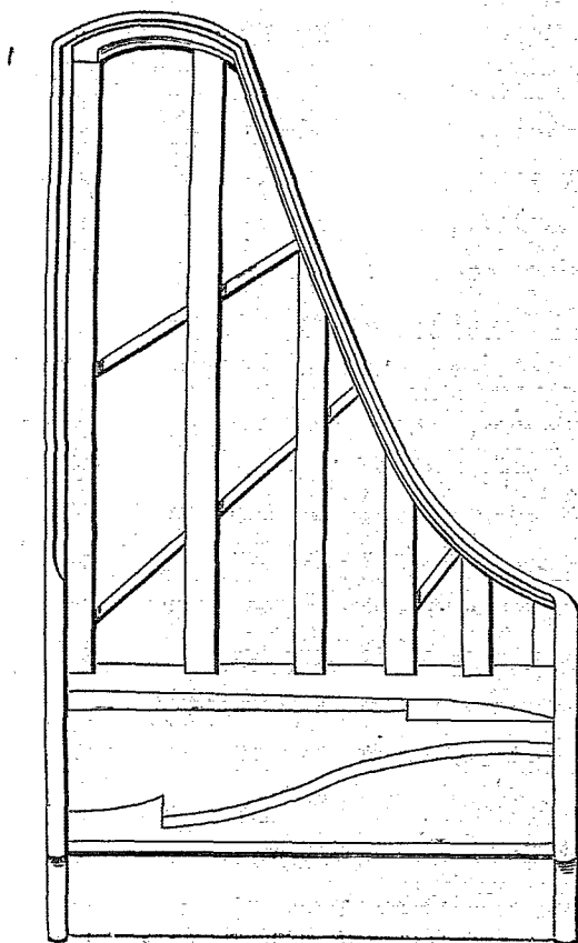
(Fig. 1. Boîte du piano.)
