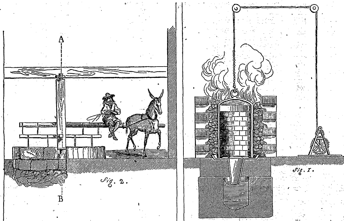
(Machine à broyer le minéral d'argent. — Coupe sur la ligne AB.)
