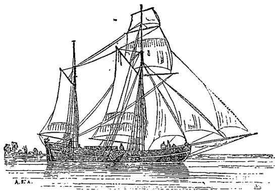
(Ga'ïote hollandaise large, les amures à babord, vue par le travers.)
