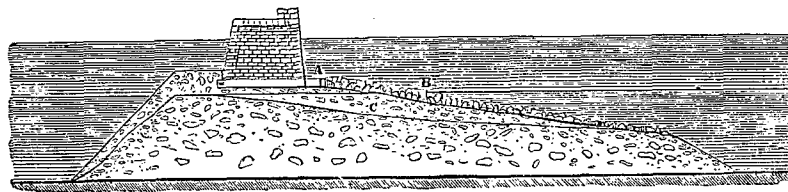
(Fig. 4. Profil en exécution pour l'achèvement de la digue de Cherbourg.)
