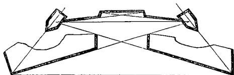
(Fig. 7. — Front de Vauban. Troisième tracé.)
