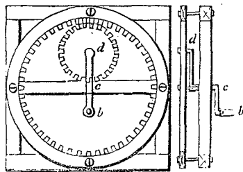
(Fig. 9.) (Fig. 9 bis.) (Epicyclic rectiligne de Lahire.)
