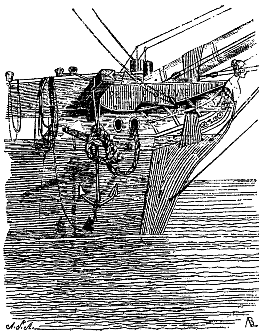
(Avant d'un brig marchand. — Voy. Bossoir.)
