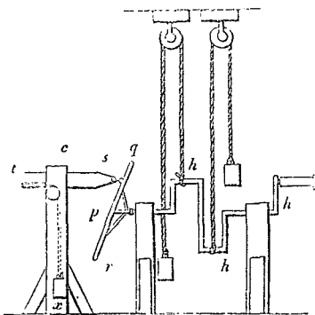
(Fig. 10. — Mouvement circulaire continu en rectiligne alternatif.)
