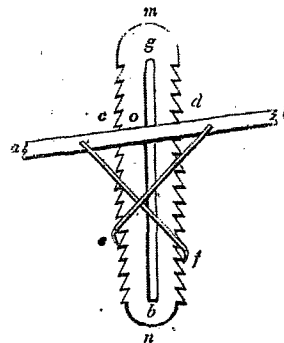
(Fig. 6. — Transformation du mouvement circulaire alternatif en rectiligne continu.)
