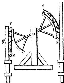
(Fig. 16. — Mouvement circulaire alternatif changé en rectiligne alternatif.)
