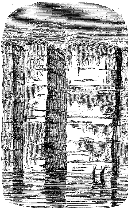
(Fissures déblayées par la mer dans l'île de Sky.)
