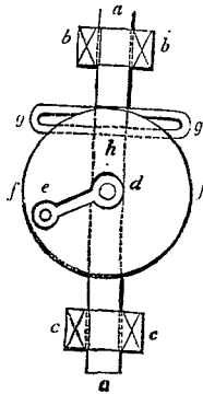
(Fig. 7. — Transformation du mouvement circulaire continu en rectiligne alternatif.)
