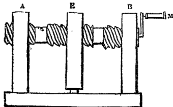
(Fig. 5. — Vis différentielle de M. de Prony.)
