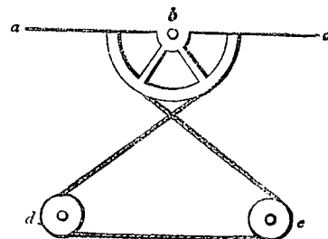
(Fig. 14. — Mouvement circulaire alternatif en rectiligne alternatif.)
