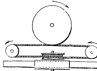
(Fig. 12. — Renvois de mouvements circulaires dans deux plans perpendiculaires.)
