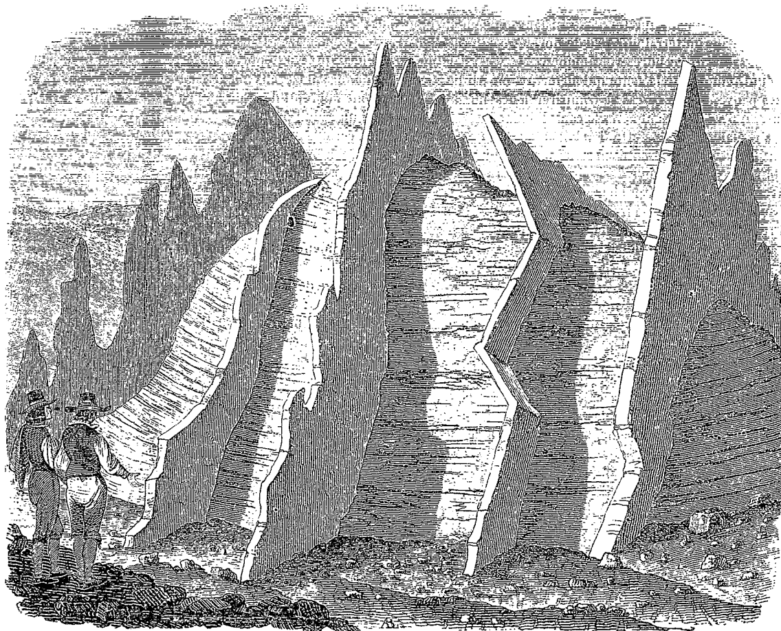
( Fissures moulées dans le val de Bove ( Etna ). )
