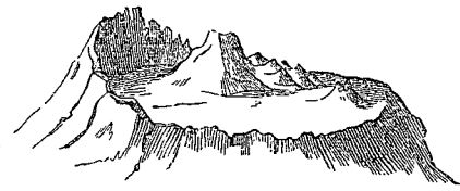
(Vue générale du cratère avant l'éruption d'août 1834. — Les escarpements du Palo sont à gauche.)
