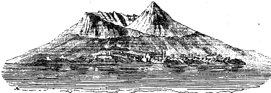
(Vue du Vésuve après l'éruption de 79.)
