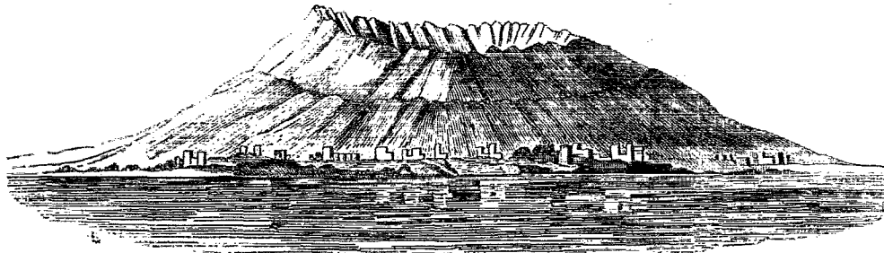
(Vue du Vésuve avant l'éruption de 79.)
