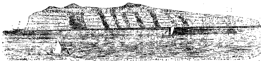
(Fissures injectées par une roche trappéenne dans une falaise, près de Shuishnish (archipel des Hébrides).)
