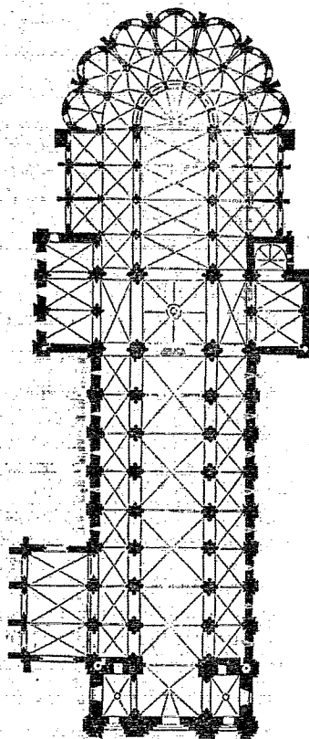
(Plan de l'église de l'Abbaye-aux-Hommes, à Caen.)
