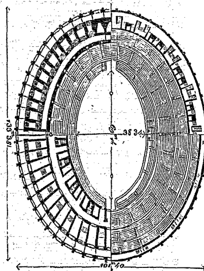
(Plan de l'amphithéâtre de Nîmes, à quatre hauteurs différentes.)
