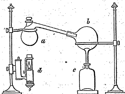
a Cornue en verre dans laquelle on verse du nitre d'abord, et ensuite de l'acide sulfurique. — b Ballon où se rendent les vapeurs d'acide nitrique. — c Flacon où ces vapeurs coulent après être redevenues liquides. — d Lampe servant à chauffer le mélange contenu dans la cornue a.
