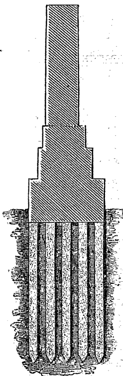
(Fig. 2. — Pilastre fondé sur pilots en sable, à l'arsenal de Bayonne.)
