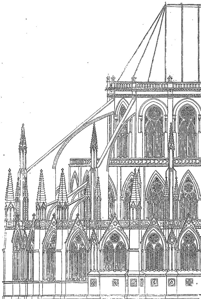
(Abside de Notre-Dame de Paris.)
