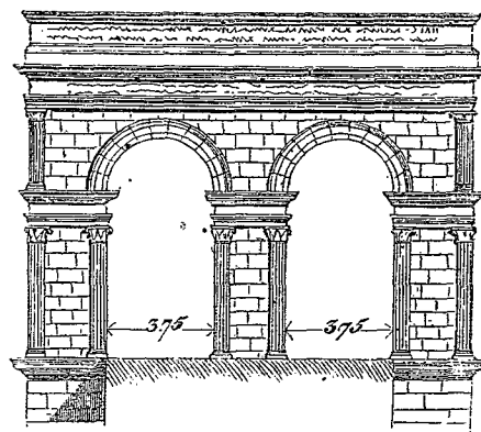
(Arc ou porte de Saintes, département de la Charente-Inférieure.)
