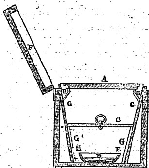
(Fig. 2. — Coupe de la boîte qui sert à fixer la couche d'iode sur la feuille d'argent plaqué.)
