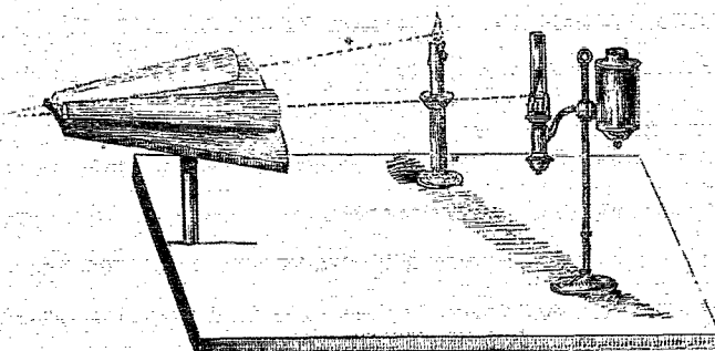
(Photomètre. — Fig. 1.)
