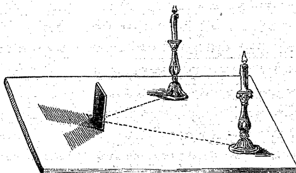
(Photomètre. — Fig. 2.)
