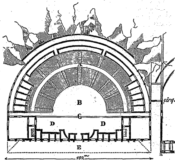
(Plan du théâtre d'Orange, département de Vaucluse.)
