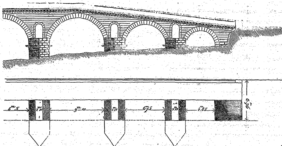
(Dessin d'une partie du pont de Sommières, dans le département du Gard.)
