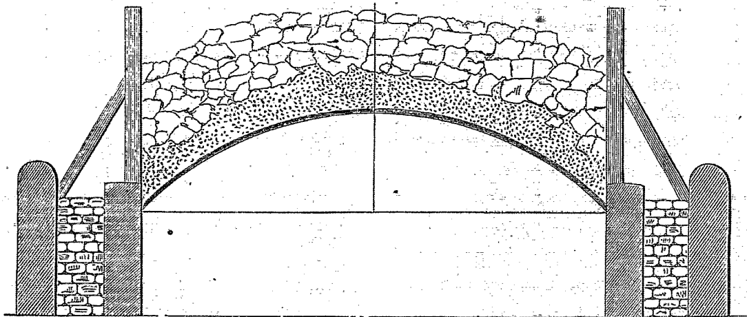
(Fig. 1. — Épreuve subie par une voûte mince en briques et en ciment de Vassy. — Un centième de grandeur naturelle.)
