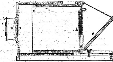
(Fig. 4. — Chambre noire.)
