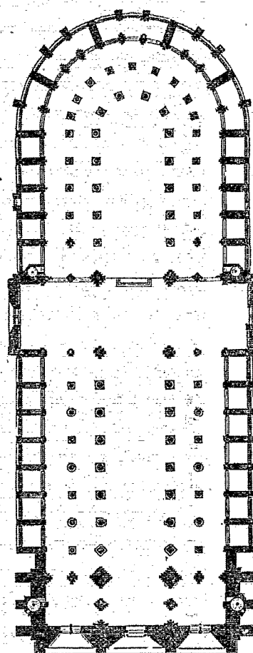
(Plan de Notre-Dame de Paris.)
