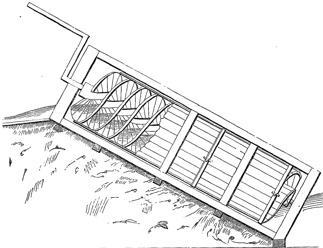
(Fig. 1. — La vis d'Archimède.)
