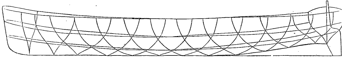
(Élévation bâisée du bateau-onde.)
