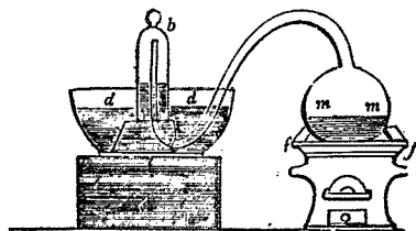
mm Mercure dans un matras à tube recourbé; l'éprouvette b, l'intérieur du matras et le tube contiennent de l'air. — ff Fourneau pour chauffer le matras. — dd Mercure pour intercepter la communication avec l'air extérieur.
