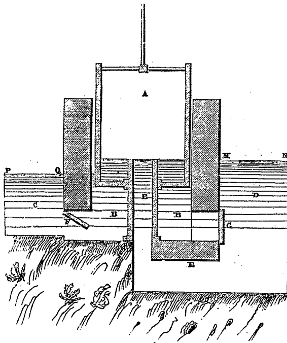
(Machine de Jappelli pour le dessèchement des marais.)
