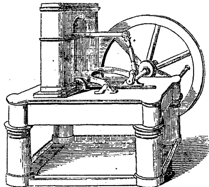
(Nouvelle presse monétaire. — Voyez le Balancier, 1836, p. 104.)
