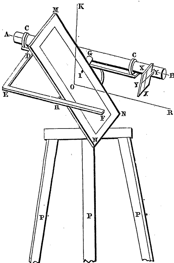
(Nouveau miroir ardent de Peyrard.)
