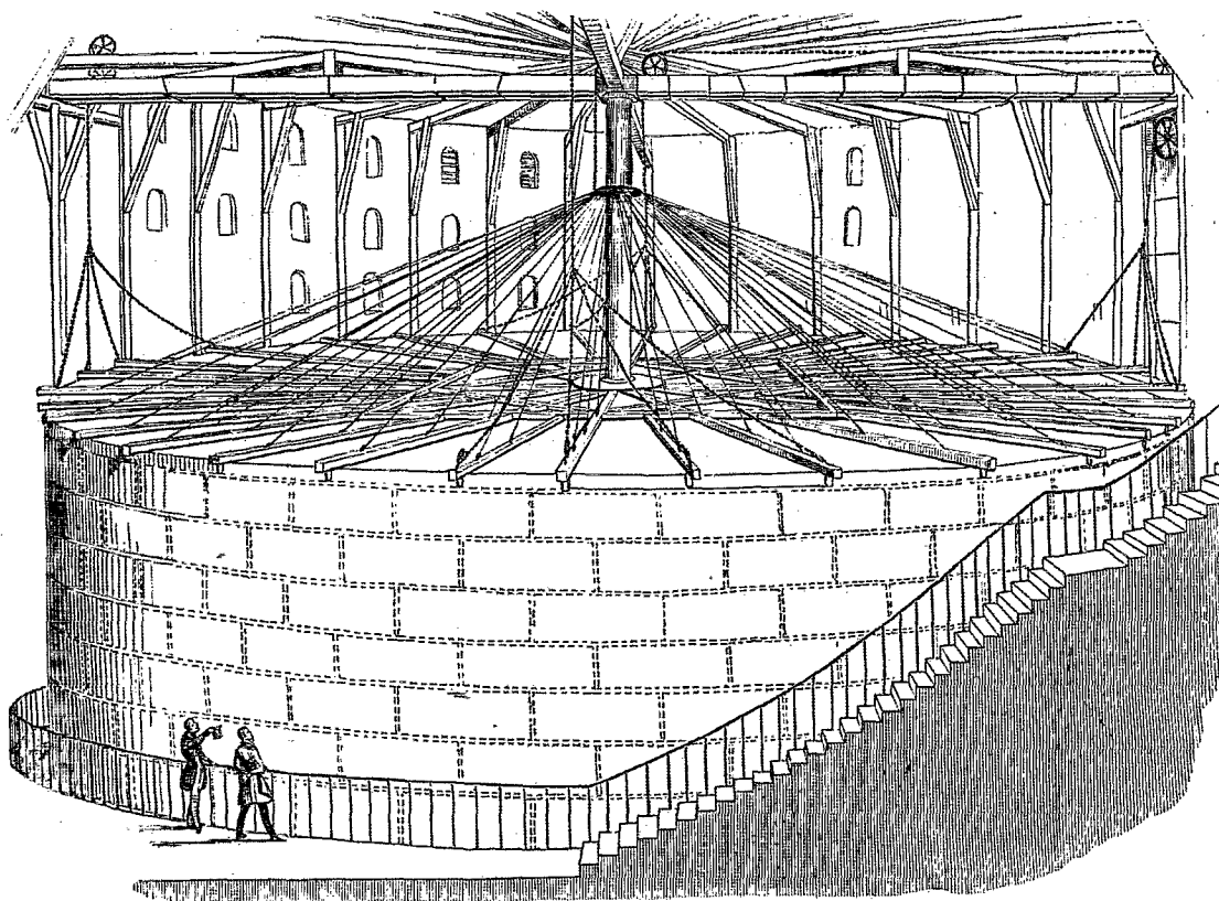
Gazomètre de la Compagnie française d'éclairage par le gaz, à Paris. — Ce dessin représente la cloche en plaques de tôle dans laquelle arrive le gaz et du sommet de laquelle il sort par un tuyau. L'appareil de suspension est indiqué par les cordes qui se réunissent à la colonne centrale, p. 147.
