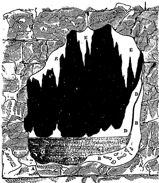
Coupe de la caverne à ossements de Kirkdale.
