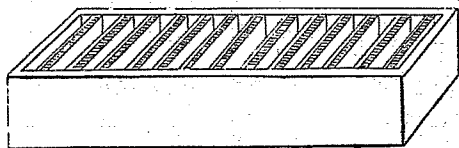
(Pile à auges. — Les élémens cuivre et zinc, soudés ensemble, sont séparés par des cases remplies d'eau acidulée.)
