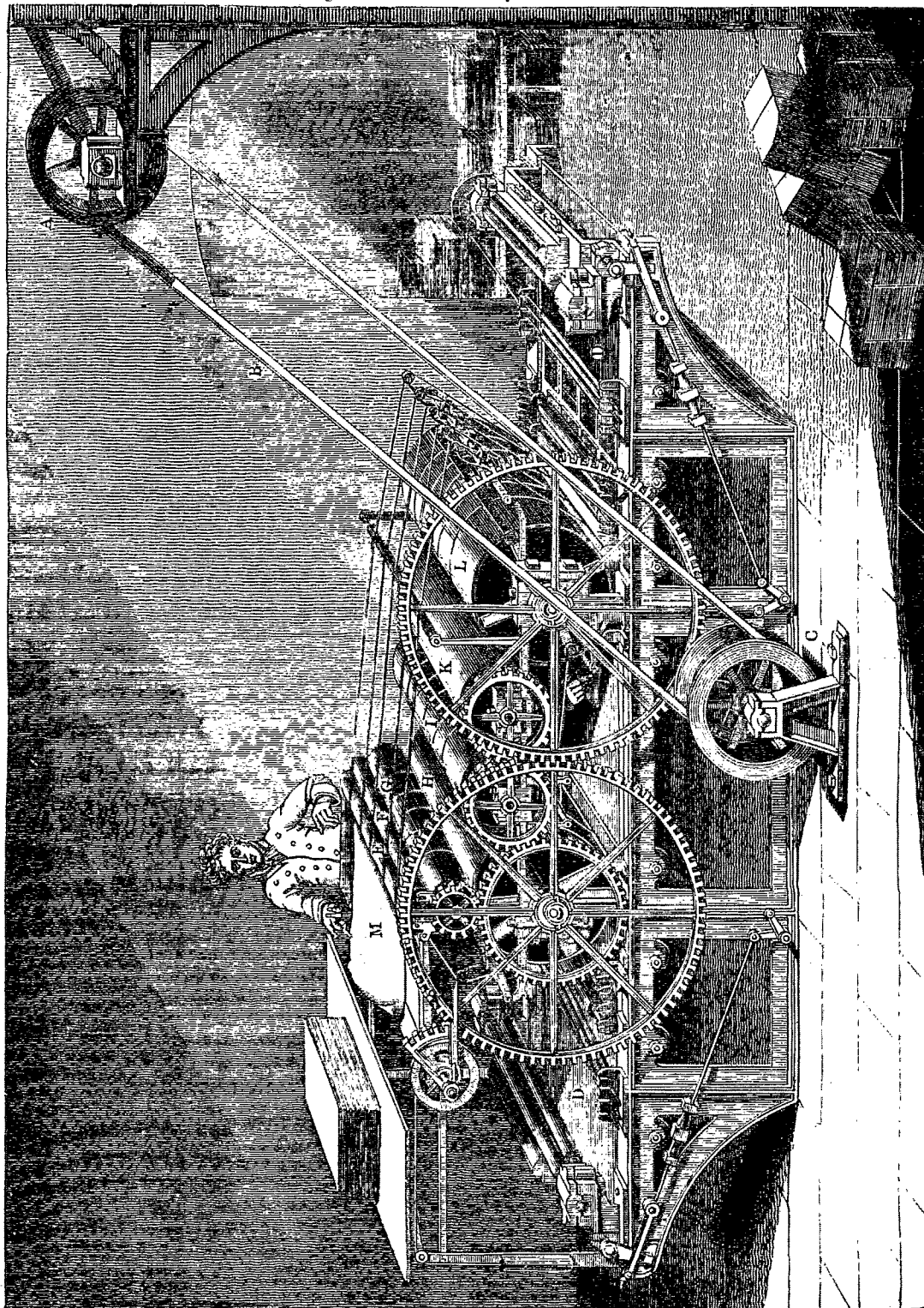
( Presse mécanique de Cower employée pour l'impression du Magasin pittoresque )
