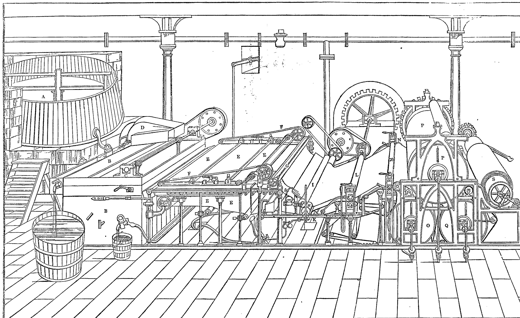
( Machine à fabriquer le papier. )
