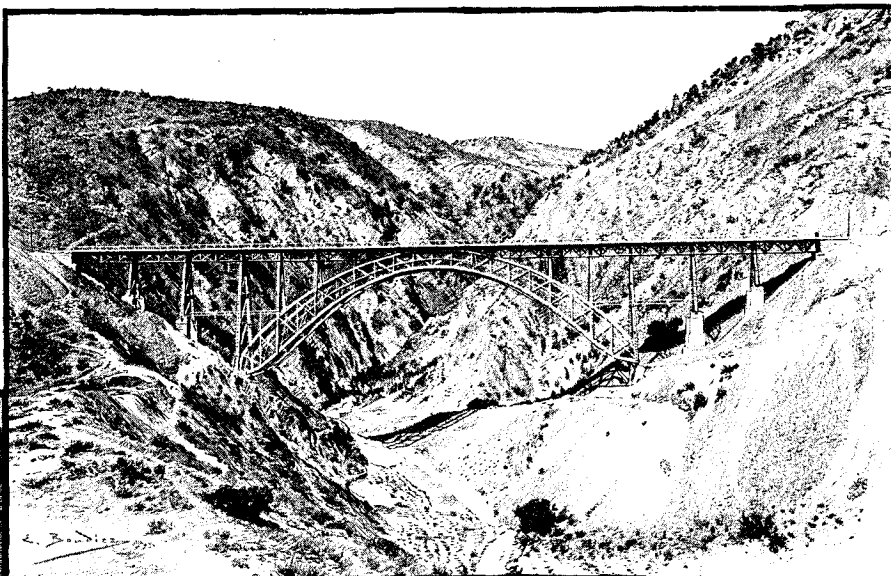
VIADUC DE BACH-KEUL.
