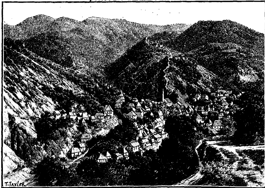
RELIEF DU NORD DE LA BOSNIE. — DESSIN DE TAYLOR.
