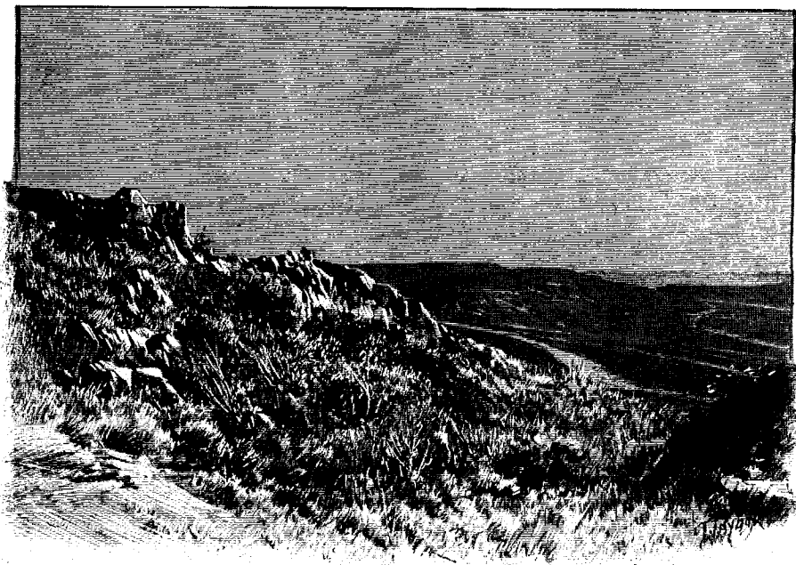
CRÊTES DE QUARTZITES AU NORD DE JOHANNESBURG. — DESSIN DE TAYLOR.
