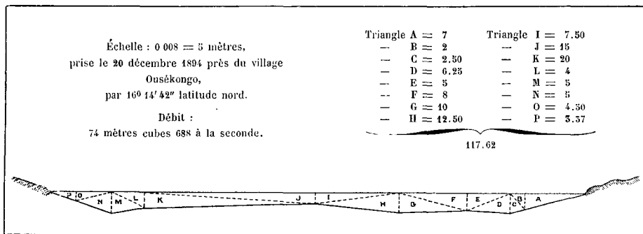
COUPE DE LA RIVIÈRE WÔM AUPRÈS DU VILLAGE DE GOUTIKORA (PAGE 29).
