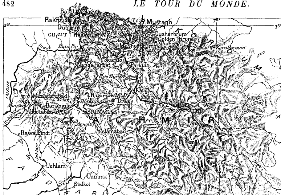
CARTE DE L'ITINÉRAIRE DE M. CONWAY DANS L'HIMALAYA.
